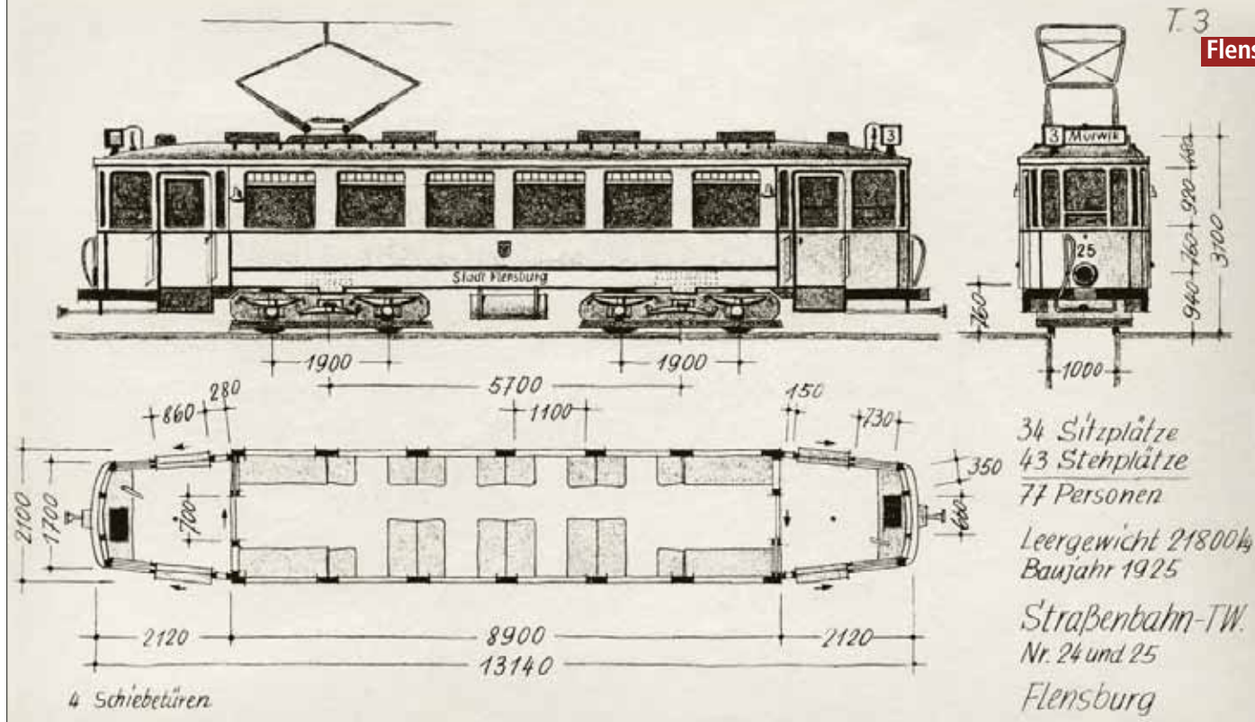
Die drei 1925 gebauten vierachsigen HAWA-Triebwagen verkehrten bis 1934 auf der elektrifizierten Kleinbahnstrecke nach Glücksburg. Trotz der modernen Fahrzeuge blieben die Beförderungszahlen Anfang der 1930er-Jahre hinter den Erwartungen zurück
