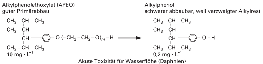
Abb. 9.19 Primärabbau von Alkylphenoethoxylaten (APEO).
