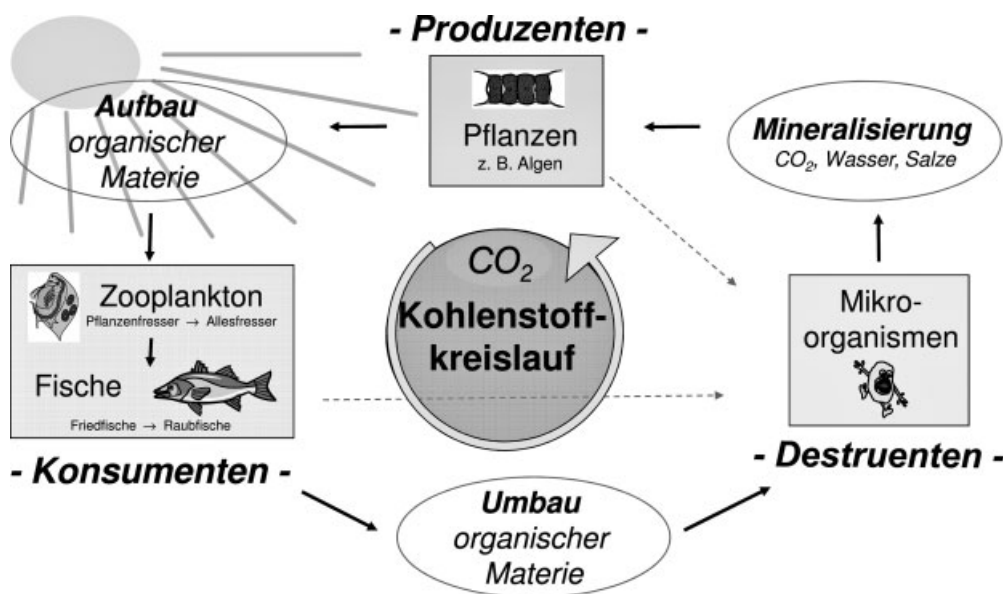
Abb. 9.9 Schema der aquatischen Nahrungskette.
