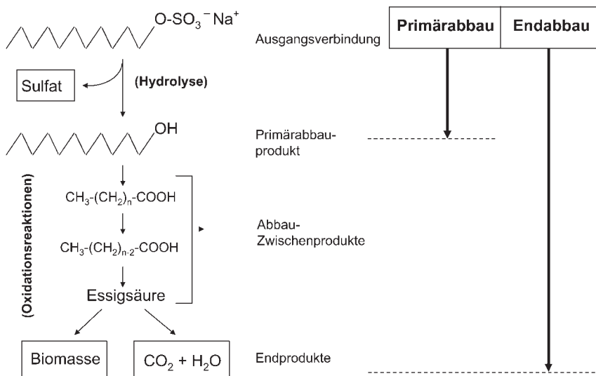
Abb. 9.13 Abbaueweg von Fettsäurealkoholsulfaten (FAS).
