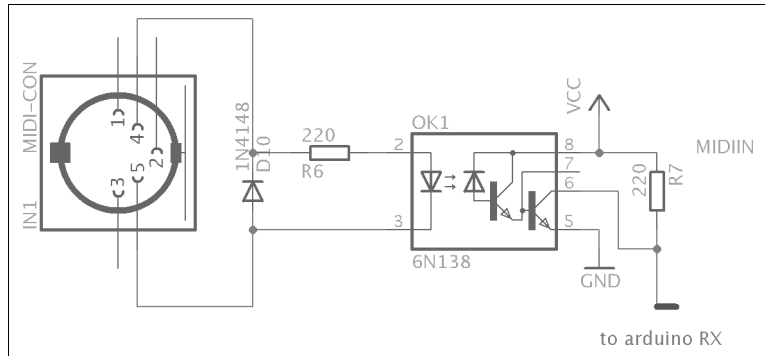
Abbildung 10-4 ► Schaltbild MIDI-Input
