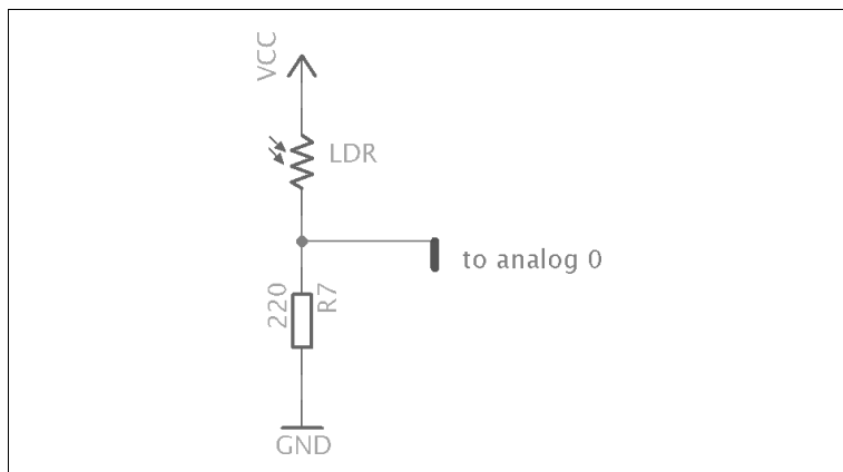
Abbildung 5-6 ► Lichtsensor-Aufbau
