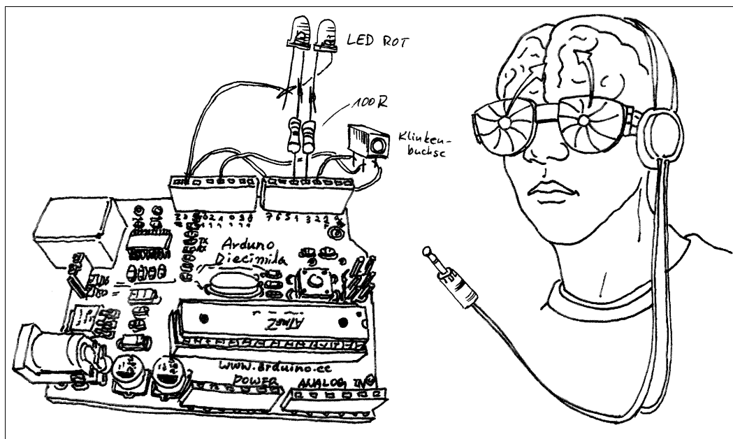
▲ Abbildung 4-5 BrainMachine-Schaltung
