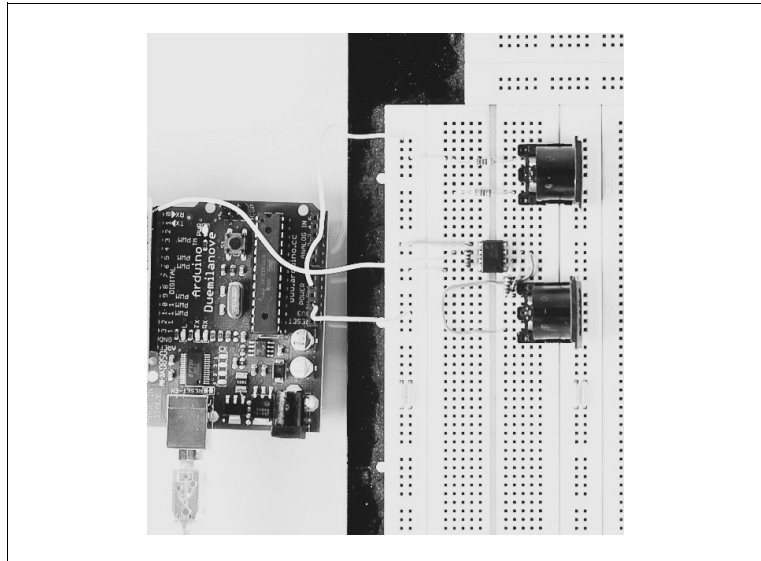
Abbildung 10-5 ► Schaltung MIDI-Input und MIDI-Output
