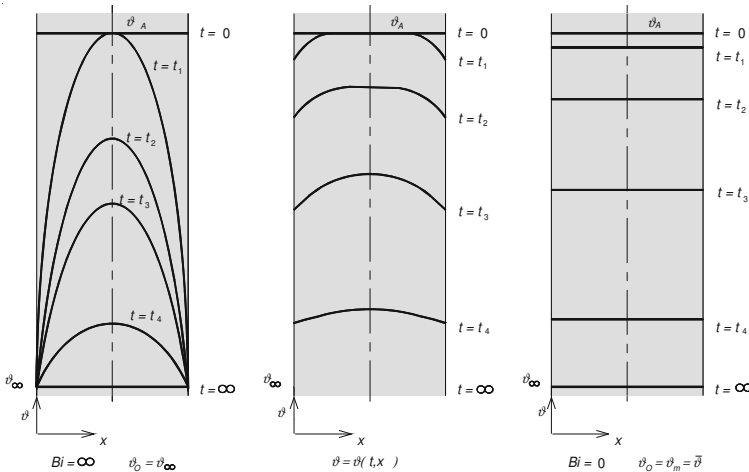
Bild 2.16: Temperaturverlauf bei Extremfällen
