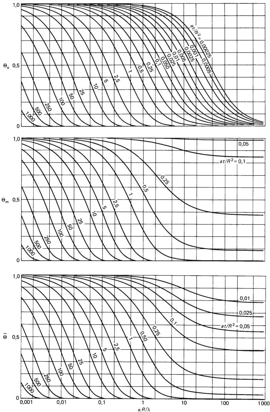
Bild 2.12: Temperaturverlauf der instationären Wärmeleitung in einem Kreiszylinder [2.1]
