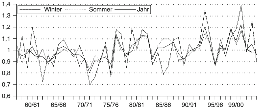
Abb. 3.9 Indizes der Erzeugungsmöglichkeit schweizerischer Wasserkraftwerke
