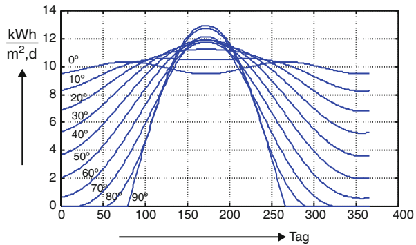
Abb. 7.27 Jahresgang der Tagesenergie auf einer horizontalen Fläche für verschiedene Breitengrade (extraterrestrische Einstrahlung 1353 \text{ W/m}^2 )
