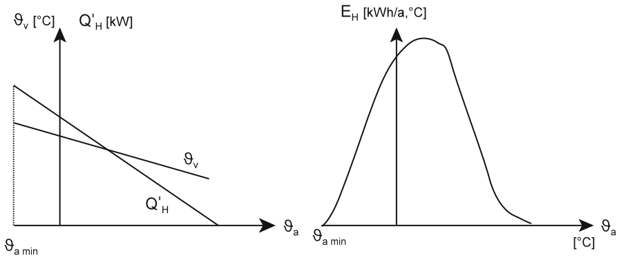
Abb. 5.54 Wärmeleistungsbedarf, Vorlauftemperatur und Jahresenergiebedarf in Abhängigkeit von der Außentemperatur
