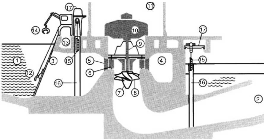
Abb. 4.5 Laufwasserkraftwerk mit Kaplan-Turbine: 1 Oberwasser, 2 Unterwasser (Saug-rohr), 3 Rechen, 4 Einlaufspirale, 5 Stützschaufeln, 6 Laufschaufeln, 7 Laufrad, 8 Laufrad-schaufeln, 9 Turbinenwelle, 10 Generator, 11 Maschinenhaus, 12 Rechenreinigungsmaschine, 13 Geschwemmsele, 14 Zangengreifer, 15 Dammbalken, 16 Nuten, 17 Krane [4.10]
