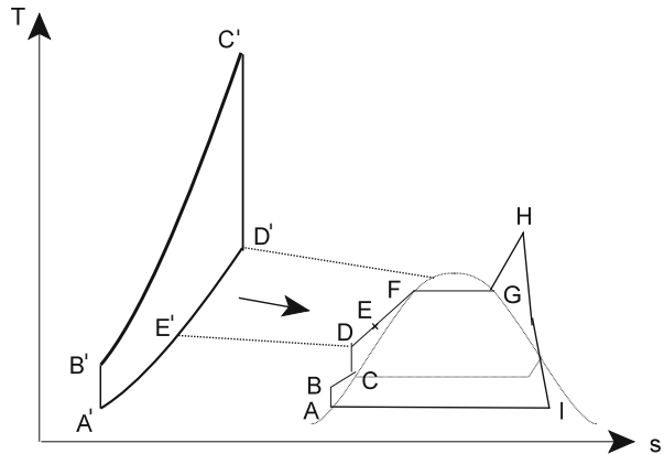
Abb. 5.10 T,s Diagramm des Kombiprozesses
