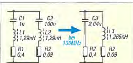
Bild 6: Entstehung eines scheinbaren Parallelschwingkreises durch Zusammenfassen der in Reihe liegenden Blindimpedanzen bei einer bestimmten Frequenz
