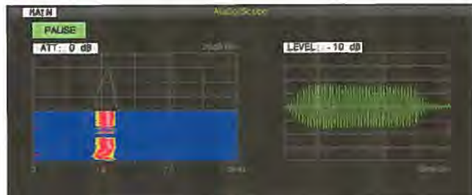
Bild 12: Das Audio-Scope mit einer Darstellungsbreite von 3 kHz; empfangen wurde ein CW-Signal bei geringer Filterbandbreite. Der Knick entstand durch kurzzeitiges Ändern der CW-Ablage.
