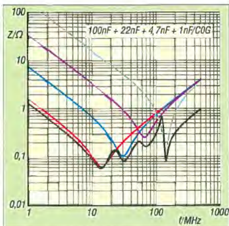
Bild 7: Impedanzverlauf bei vier parallel liegenden Kondensatoren und Staffelung der Werte im Verhältnis 5:1; der kleinste Kondensator besteht aus verlustarmer C0G-Keramik.
