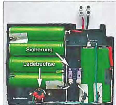
Bild 2: Geöffneter, umgebauter Akkupack mit Sicherung und Ladebuchse und der Klemme für den Anschluss des Verbrauchers
