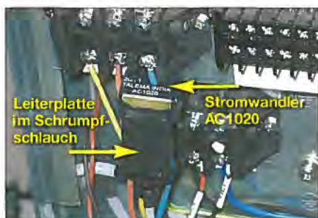
Bild 1: Einsatz des Stromwandlermoduls direkt an einer Schraubklemme
