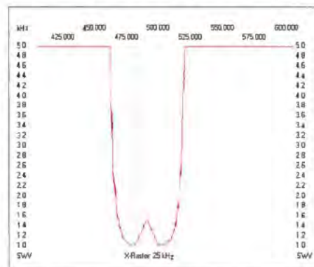
Bild 8: Das ominöse „W“ bei der Messung mit dem FA-NWT Screenshots: DK1KQ
