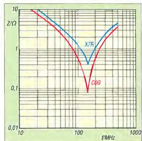
Bild 3: Typischer Impedanzverlauf von 1-nF-Kondensatoren der Größe 0805 in den Keramiksorten X7R und C0G (aus einem Datenblatt des Herstellers AVX [1])
