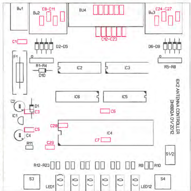
Bild 11: Bestückungsplan des Steuergeräts; die rot markierten Bauteile sind auf der Unterseite aufzulöten; Abmessungen 100 mm × 100 mm, M 1:1
