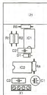
Bild 5: Bestückungsplan des Stromwandlers
