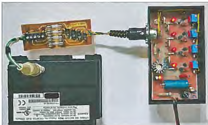
Bild 1: Ansicht während des Ladevorganges; im Ladekabel ist die Schutzschaltung auf einer Platine untergebracht.
