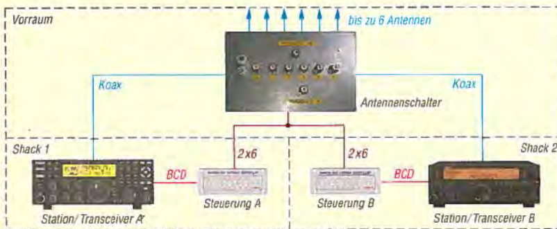
Bild 6: Befinden sich die Funkgeräte in zwei Shacks, ist je Transceiver ein Steuergerät nötig. Die Steuerleitungen sind am Antennenschalter parallelgeschaltet.
