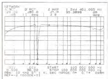
Bild 2: Frequenzgang der Kombination aus Sonde und Vorverstärker
