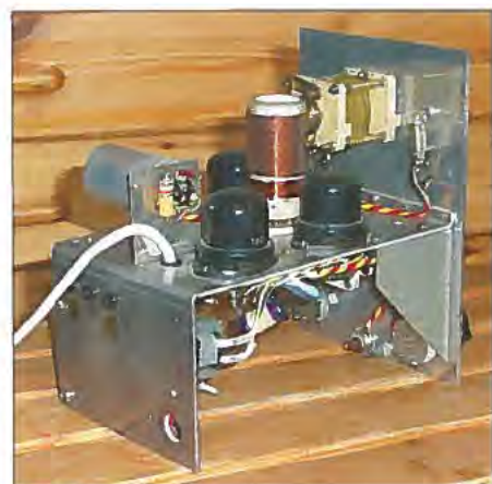
Bild 9: Innenleben des DASH-Empfängers aus dem 1950er-Jahren
