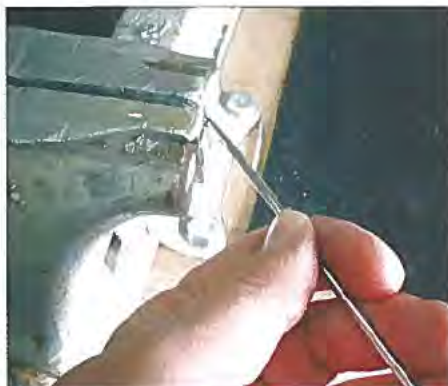
Bild 2: Bearbeitung eines Antennenelements im Schraubstock
