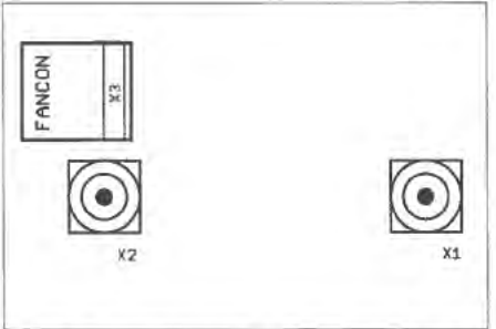
Bild 15: Bestückungsplan der Oberseite des externen Messkopfs mit den Steckern
