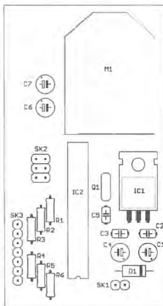
Bild 8: Bestückungs- plan der Platine für die Roboter- ansteuerung; Abmessungen 86 × 51 mm 2 , M 1:1
