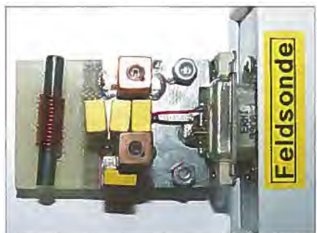
Bild 1: Mustersaufbau der Spezialantenne mit Sperrfilter für 990 kHz Foto: DB1NV
