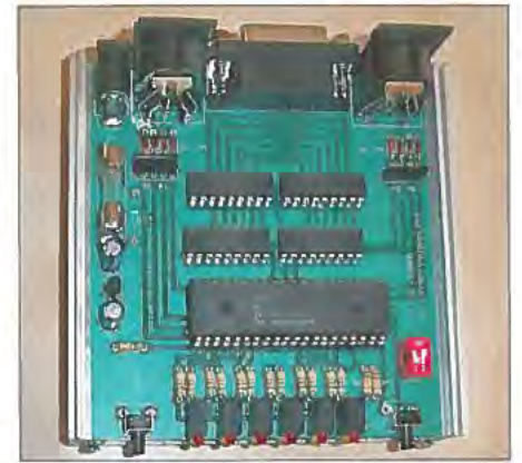
Bild 7: Aufgebaute Prototyp-Platine, eingeschoben in die untere Gehäusehälfte
