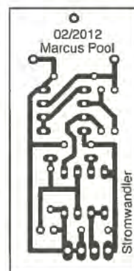
Bild 4: Layout; Abmessungen 24,3 x 49,6 mm², M 1:1
