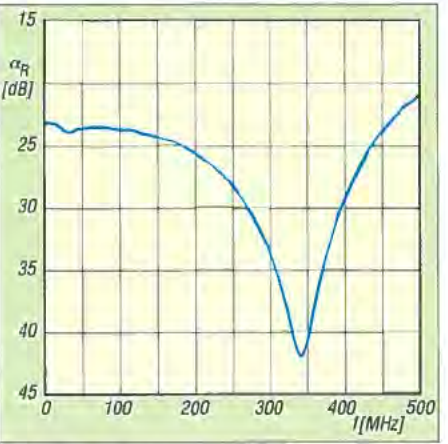
Bild 11: Die Rückflussdämpfung \alpha_R des externen Detektors/Leistungsmessers liegt im Frequenzbereich von 1 MHz bis 450 MHz stets über 23 dB, was einem SWV von s \leq 1,15 entspricht.
