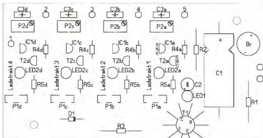
Bild 4: Bestückungsplan des Lilon-Ladegeräts; Abmessungen 115 mm x 60 mm, M 1:1
