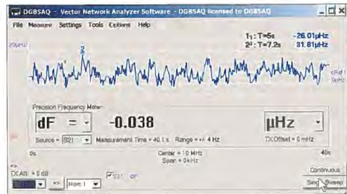
Bild 6: Externer Frequenzstandard gegen sich selbst gemessen, gemittelt mit gleitendem Durchschnitt über 1 s Messdauer. Das ebenfalls eingeblendete Frequenzmeter-Werkzeug zeigt die über die gesamte Messdauer ermittelte Frequenz an.
