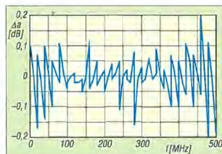
Bild 18: Die Abweichung der Anzeige des frequenzkompensierten Messkopfs liegt bei einem Eingangspegel von U_E = 10 dBm und softwaremäßiger Korrektur stets unter 0,2 dB.
