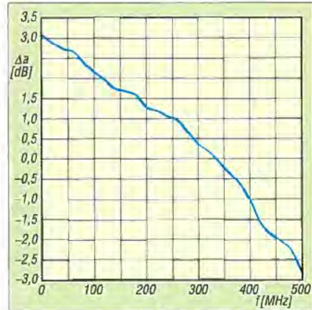
Bild 4: Abweichung der Anzeige vom Sollwert ohne Verwendung der Korrekturtabelle
