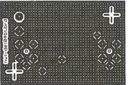
Bild 13: Leiterplattenlayout der Oberseite; Abmessungen 45 mm × 30 mm, M 1:1,3
