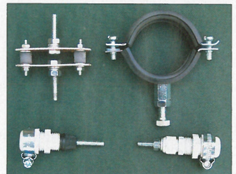
Bild 7: Zum Teil selbst hergestellte Bauteile: oben links ein Achsenausgleich, rechts die Befestigungsschelle für den Vakuumdrehkondensator, unten je eine isolierende Kupplung für 12,7-mm- und 8-mm-Achsen
