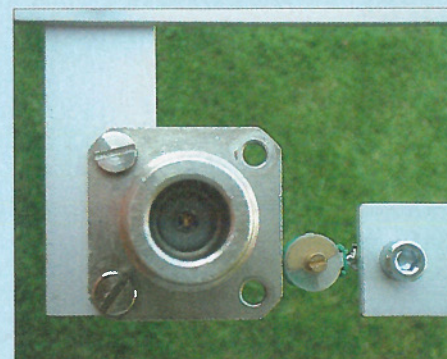
Bild 7: Der Trimmer zur Anpassung der Antenne befindet sich neben der Antennenbuchse und ist gut zugänglich.
