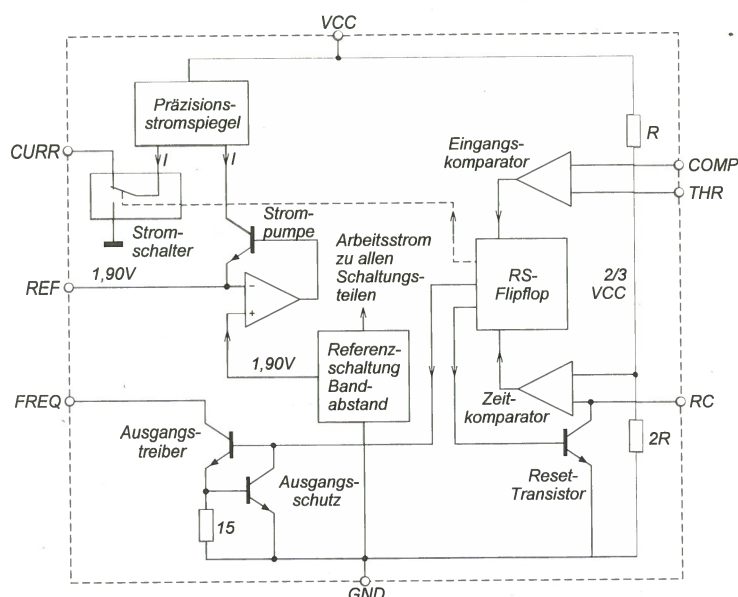
Bild 1: Blockschaltbild des KA331
