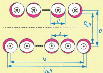
Bild 9: Die reale Spule vereint beide Arten von Stromverdrängung. Der Stromschwerpunkt wandert nach innen, dadurch wird der für die Induktivität maßgebende Durchmesser D_{\text{eff}} kleiner.
