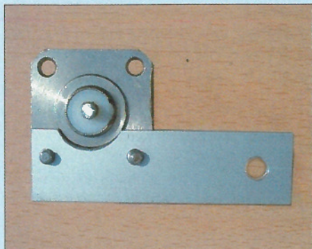
Bild 3: Die N-Einbaubuchse wird mit zwei M3-Schrauben befestigt.
