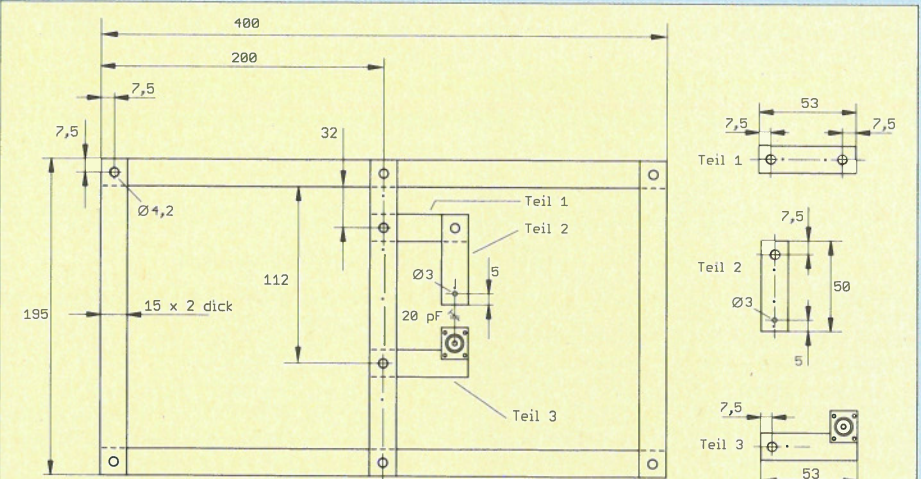
Bild 2: Abmessungen der Fensterscheibenantenne
