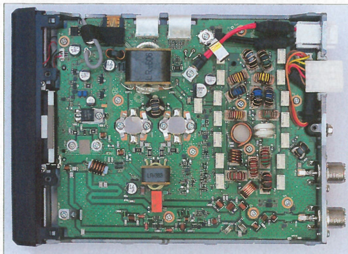
Bild 5: Innenansicht der Haupteinheit von unten; die grau erscheinenden Flächen sind elastische Kissen mit Metallgewebeerfläche, die bei geschlossenem Deckel guten Kontakt zu ihm herstellen, um HF-technischen Belangen Genüge zu tun.
