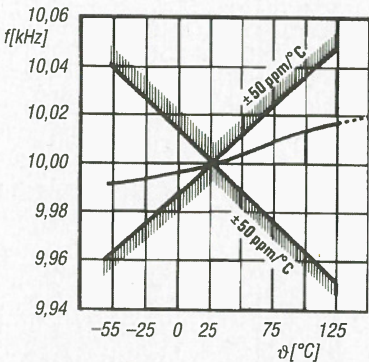
Bild 4: Typische Abhängigkeit der Ausgangsfrequenz f von der Temperatur θ; die spezifizierten Maximalwerte betragen ±50 ppm/°C
