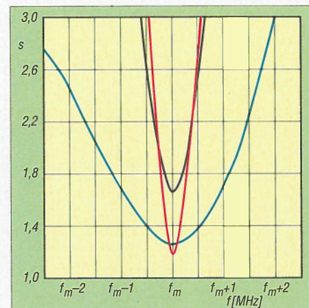
Bild 7: Gemessene SWVs auf 40 m (rot), 20 m (blau) und 15 m (schwarz); Mittenfrequenzen f_m bei 7,0 MHz, 14,35 MHz und 21,75 MHz
