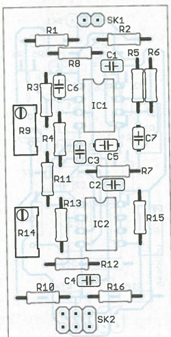
Bild 8: Bestückungsplan der Sensorbaugruppe; Abmessungen 65 mm × 32 mm, M 1:1
