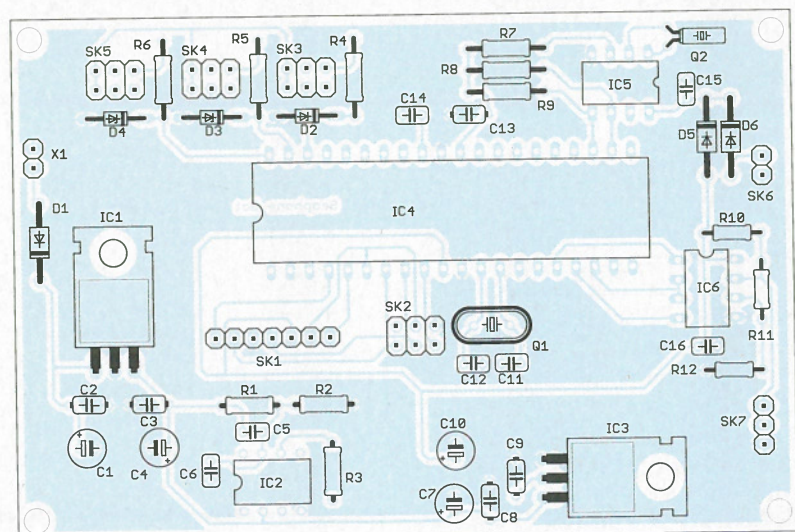
Bild 9: Bestückungsplan der Controllerbaugruppe; Abmessungen 104 mm × 69 mm, M 1:1
