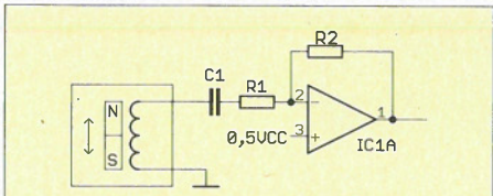
Bild 5: Einfacher Vorverstärker
