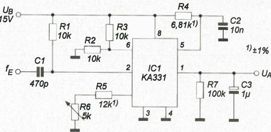
Bild 8: Frequenz-Spannungs-Umsetzer für Eingangsfrequenzen bis f E = 10 kHz mit einer Nichtlinearität von ±0,06 %;
