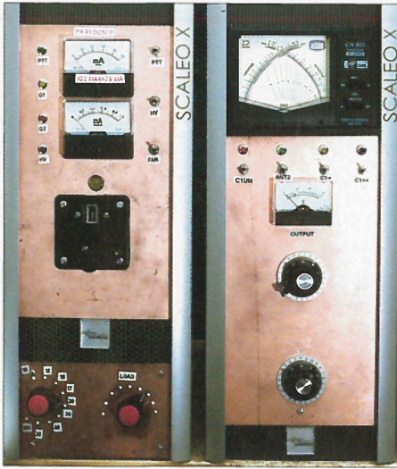
Bild 3: L-Antennenkoppler mit eingebautem SWV-Messgerät neben der Röhrenendstufe; beide ließen sich sehr gut in einem leeren Industrie-PC-Gehäuse unterbringen.
