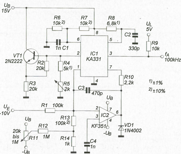
Bild 7: Spannungs-Frequenz-Umsetzer für Eingangsspannungen U E = 0 ... -10 V (f A = 1 Hz ... 100 kHz) mit einer Nichtlinearität von ±0,03 %;
