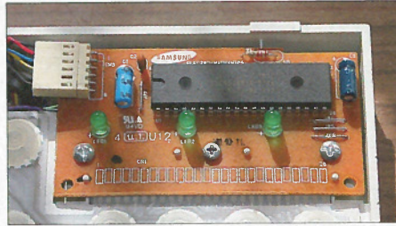
Bild 4: Auf der Platineunterseite mit dem großen Tastatur-IC lassen sich die Verbindungsdrähte zu den Tasten anlöten.
