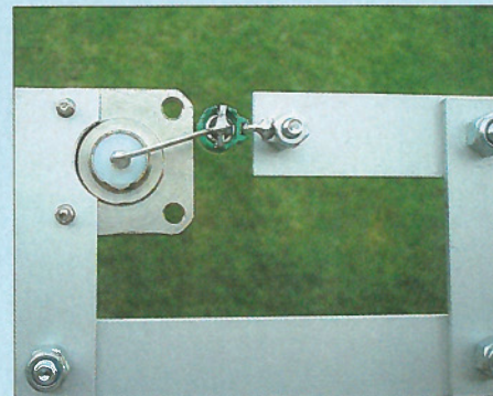
Bild 6: Rückseitige Ansicht des eingebauten Trimmerkondensators
