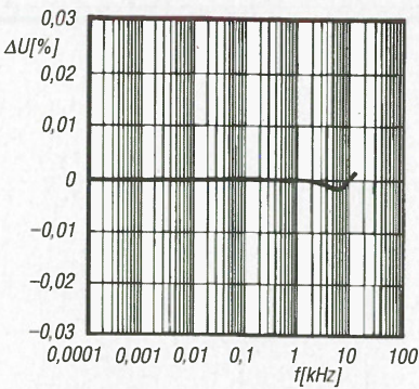
Bild 3: Linearitätsfehler der Ausgangsspannung ΔU A in Abhängigkeit von der Eingangsfrequenz f
