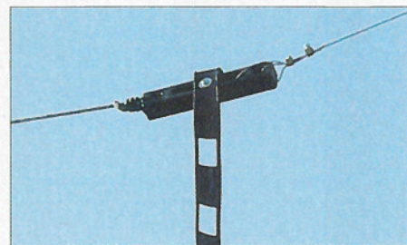
Bild 3: Isolator an der Einspeisung mit Abspannung links und Antennendraht rechts Fotos: DK7ZB
