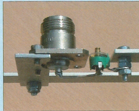
Bild 5: Einbaulage des Trimmers zwischen Antenne und Anschlussbuchse
