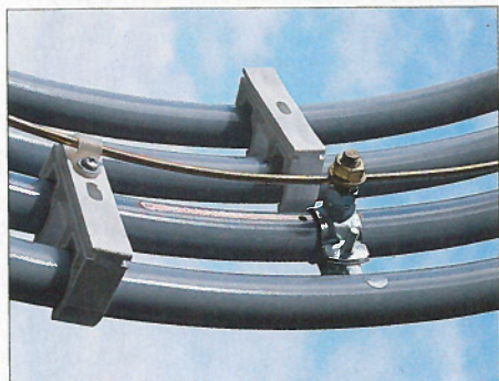
Bild 4: Eine Besonderheit dieser Magnetantenne ist der mittlere „Gamma Match“ optimierbare Anpassbereich, um so auf Umgebungseinflüsse zu reagieren.
