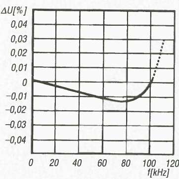
Bild 6: Linearitätsfehler der Ausgangsspannung ΔU A in Abhängigkeit von der Eingangsfrequenz f für die Schaltung in Bild 7
