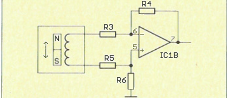
Bild 6: Für den Vorverstärker besser geeignete Variante
