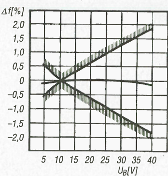
Bild 5: Typische Abhängigkeit der Ausgangsfrequenz f von der Betriebsspannung U B ; Grenzwerte eingetragen
