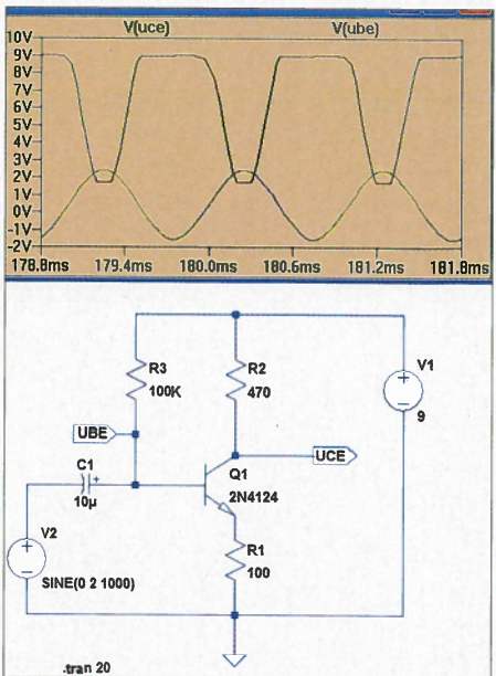
Bild 21: Zu große Eingangssignale führen zur Übersteuerung der Stufe. Eine lineare Signalverstärkung ist somit unmöglich.
