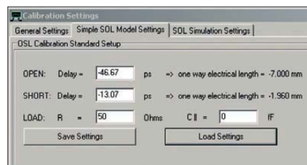
Bild 14: Eingabewerte für Calibration to Center of Thru mit Rosenberger-Cal-Standards aus Bild 9 (nach OZ7OU)
