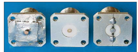
Bild 10: Eigenbau-SOLT-Kalibrierelemente in N-Norm; physikalische Bezugsebene ist die plane Flanschrückseite ( Open –17,62 ps wegen der Endkapazität, Short 0 ps, Delay zur genormten Bezugsebene 43,44 ps).
