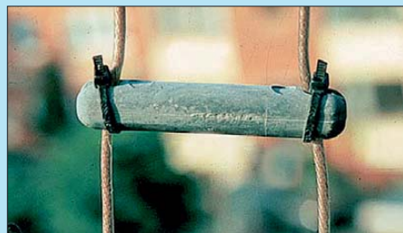
Bild 10: Fixierung des Spreizers mit Plastik-kabelbindern
