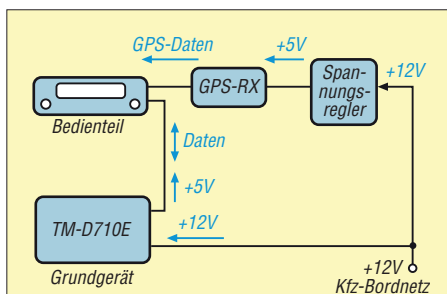
Bild 4: Anschluss eines konventionellen GPS-Moduls an den TM-D710E
