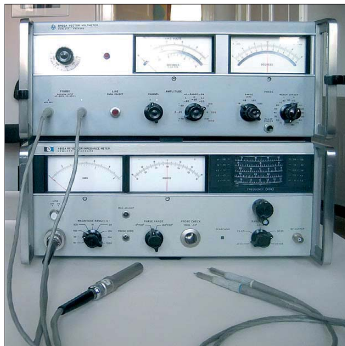
Bild 8: Messplatz, mit dem die HF-Eigenschaften des Symmetrierübertragers ermittelt wurden
