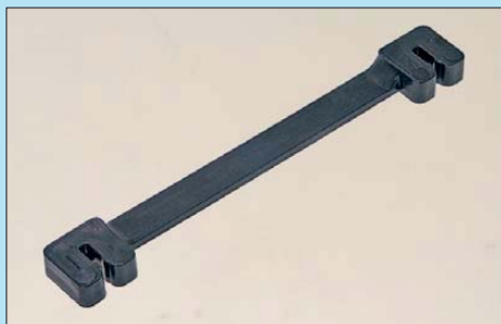
Bild 14: Vom Gewächshaus zur Antenne; diese auf die Leiter aufsteckbaren Spreizer sind extrem leicht und gut handhabbar.
