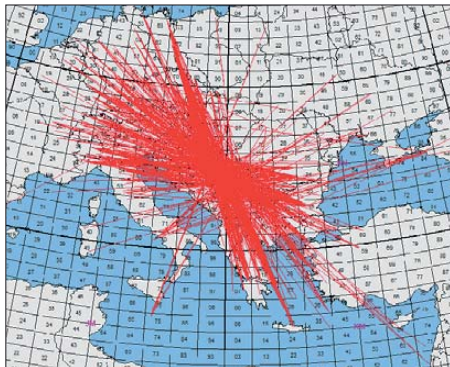
Sporadic-E-Wolken über Serbien am 9. 6. 12
