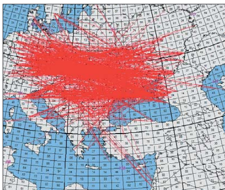
144-MHz-Verbindungen vom Westen Deutschlands bis ans Kaspische Meer am 1. 7. 12
