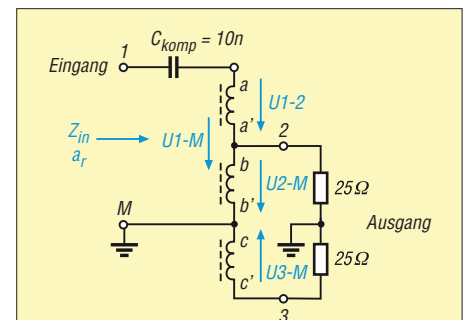
Bild 4: Schaltbild des kompensierten Symmetrierübertragers und Nennbelastung mit 2 \times 25,5 \, \Omega
