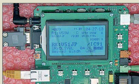
Genial digital: die universelle, frei programmierbare Plattform für digitalen Amateurfunk „UP4DAR“, konstruiert von Michael Dirska (DL1BFF) und Denis Bederov (DL3OCK)
