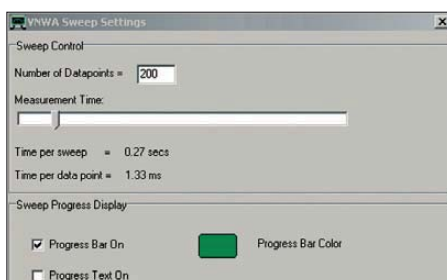
Bild 5: Vor dem Kalibrieren müssen die Anzahl der Messpunkte sowie die Zeit für einen Frequenzdurchlauf festgelegt werden.
