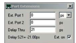
Bild 15: Verschieben der Bezugsebene von Center of Thru (aus Bild 14) nach Male Reference Plane
