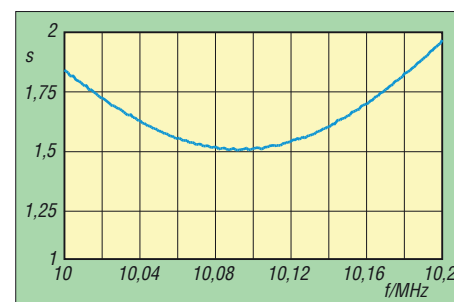
Bild 7: Stehwellenverhältnis des Kelemen DP-WARC im 30-m-Band nach dem Abgleich
