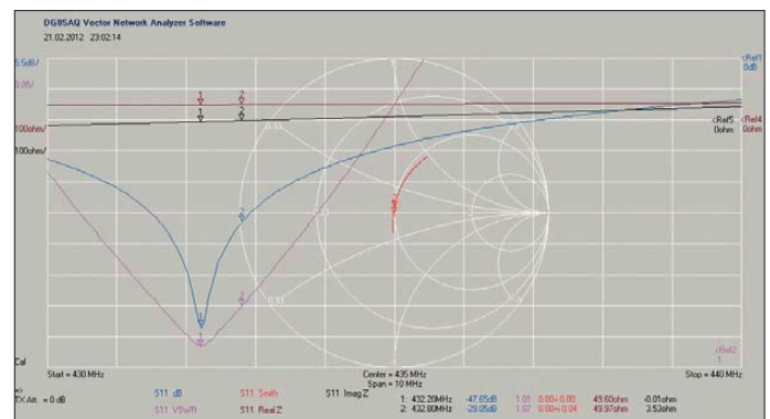
Bild 6: S_{11} -Messungen an einer Halo-Antenne: Rückflussdämpfung (blau), Stehwellenverhältnis (violett), Lage der Anpassung am 50-Ω-Punkt im Smith-Diagramm (rot), Wirk- (gelb) und Blindwiderstand (schwarz)
