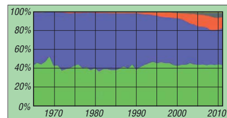
Verteilung der verschiedenen Sendeararten seit 1965; die Farben stehen für die Sendeararten: grün = Telegrafie, blau = Telefonie, rot = RTTY, grau = PSK.
