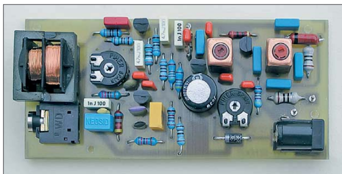
Bild 1: Die Leiterplatte des AM-Prüfgenerators ist vor der Inbetriebnahme in ein Metallgehäuse einzubauen.
