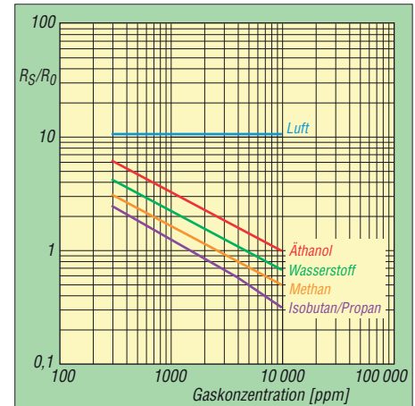
Bild 5: Empfindlichkeit des TGS2610 in Abhängigkeit der Konzentrationen unterschiedlicher Gase
