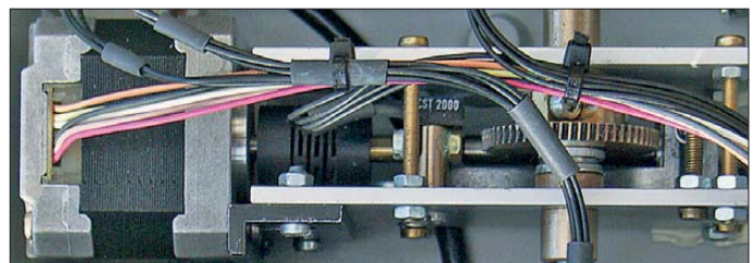
Bild 4: Schrittmotor 1, Kupplung und Schneckengetriebe sowie Gabellichtschranke der Antriebseinheit des Abstimm drehkondensators
