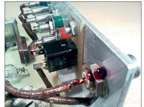
Bild 2: Verdrahtung an der Rückseite der Frontplatte; zum roten Lack s. Text
