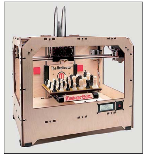
Bild 2: Der Replicator zusammen mit einem gedruckten Schachspiel
