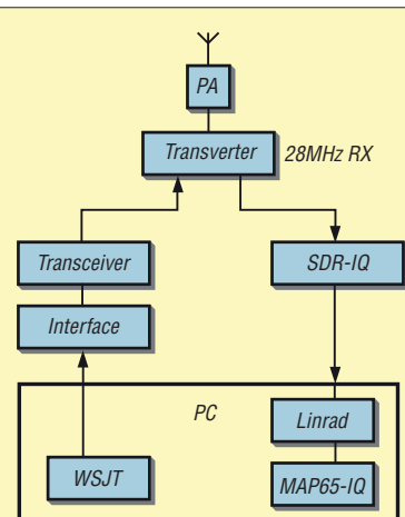
Bild 9: Colin Roberts, G4ZFJ, sendet WSJT mit dem PC, dessen NF-Ausgangssignal per Interface über Transceiver, Transverter und Endstufe zur Antenne gelangt [6]. Empfangsseitig ist der Transverter mit dem SDR-IQ und dieser per USB mit dem PC verbunden. Die Signale (einer Polarisationsebene) werden von Linrad und MAP65-IQ weiterverarbeitet.
