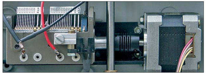
Bild 6: Schrittmotor 2, Kupplung und Gabel- lichtschranke der Antriebseinheit des Drehkondensators zur Impedanzan- passung
