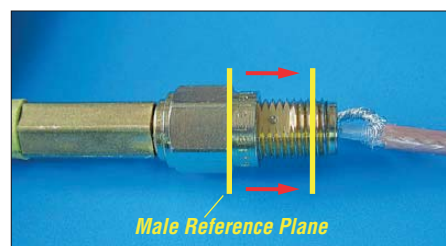
Bild 21: Impedanzmessung am eingesteckten RG59; die Reference Plane muss rechts im Thru liegen. Alternativ kann dorthin auch direkt kalibriert werden (mit Rosenberger-Cal-Standards: Open -4,67 ps , Short +28,93 ps ).
