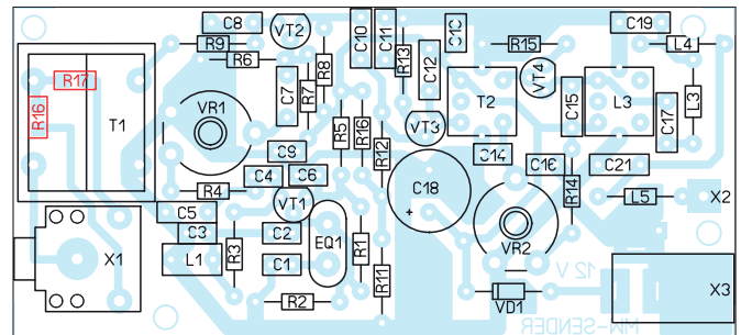
Bild 4: Bestückungsplan des AM-Prüfgenerators; die beiden rot markierten Bauelemente sind auf der Leiterseite (Unterseite) aufzulöten.
