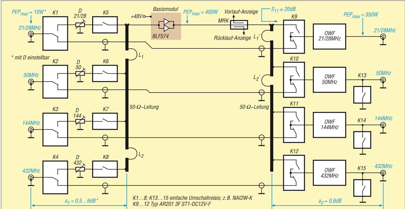
Bild 4: Blockschaltbild der kompletten Breitband-Endstufe mit BLF574-PA-Modul gemäß Bild 2, Umschaltrelais, Dämpfungsgliedern und Oberwellenfiltern
