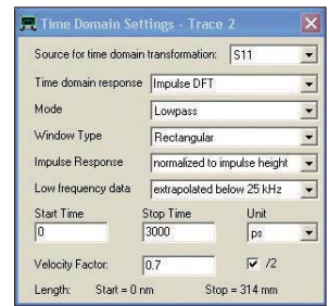
Bild 25: Einstellungen zur Längenmessung einer Koaxialleitung
