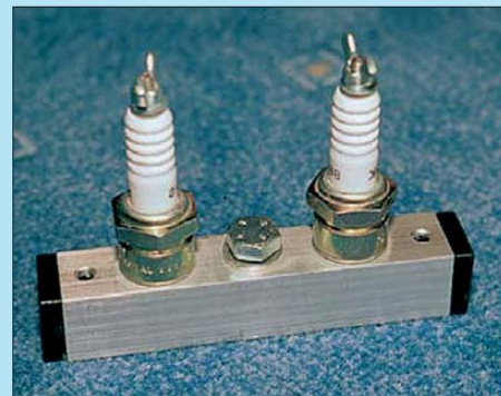
Bild 22: Überspannungsschutz mit Zündkerzen, ein ehemaliges Produkt von Alfred Annecke
