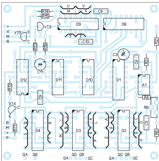
Bild 4: Bestückungsplan der Steuerelektronik; Abmessungen 80 mm x 80 mm, M 1:1; die Platinenlayouts für alle drei Leiterplatten stehen im Download-Bereich auf www.funkamateurl.de zur Verfügung.
