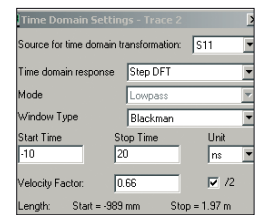
Bild 22: Einstellungen zum Messen des Wellenwiderstands eines Koaxialkabels
