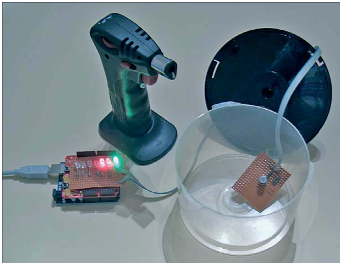
Bild 1: Beim Versuchsaufbau in einer leeren CD-Spindel erfolgte der Test mit Feuerzeuggas. Da es schwerer als Luft ist, sammelt es sich im Behälter und führt über den dort positionierten Gas-sensor TGS2610 zum Auslösen eines Alarms.
