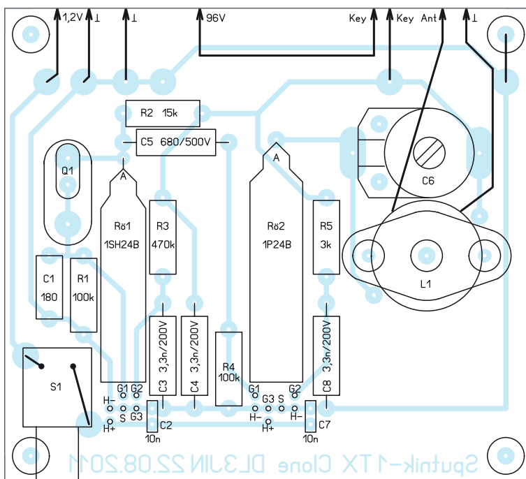
Bild 9: Bestückungsplan der einseitigen Platine
