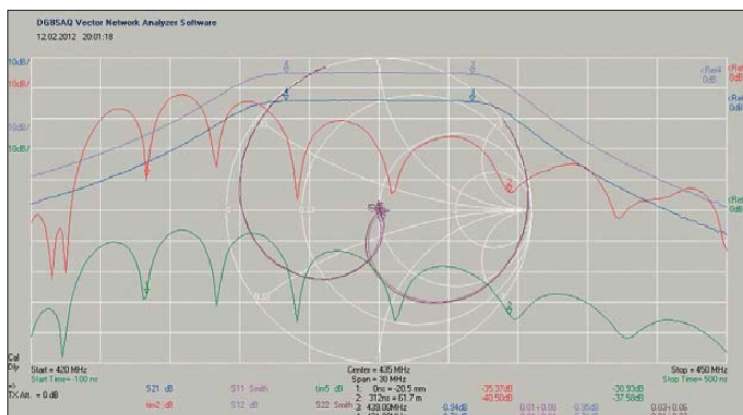
Bild 28: S_{11} (violett) und S_{22} (braun) drängen sich wunschgemäß sehr eng um den 50\text{-}\Omega -Punkt im Smith-Diagramm. Der Abgleich gelingt alternativ mit einer Darstellung im Zeitbereich: \text{tim2} (rot) und \text{tim5} (grün).
