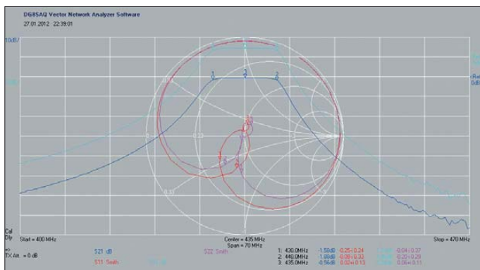
Bild 26: Dem VNWA bleibt nichts verborgen; zwar sieht die Durchlasskurve gut aus, doch die Ein- und Ausgangsimpedanzen haben nur bei 435 MHz näherungsweise 50\ \Omega plus induktivem Anteil.
