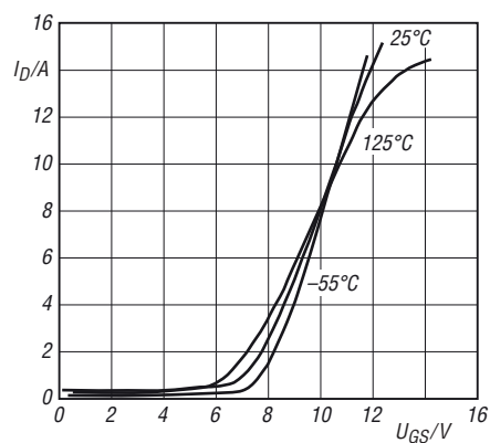
Bild 6: Abhängigkeit des Drain-Stroms I_D von der Gate-Source-Spannung U_{GS} bei unterschiedlichen Betriebstemperaturen \theta_B
