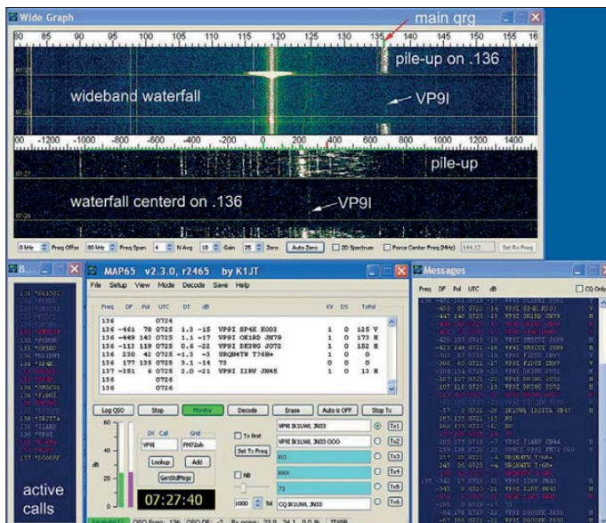
Bild 1: MAP65-Screenshot des Pile-ups von VP9I bei IK1UWL; diese DXpedition funkte 2012 mit nur einer Kreuz-Yagi auf 144 MHz via EME. Links sind die anrufernden Stationen mit ihren Frequenzen aufgelistet und rechts die gesendeten Nachrichten. In der Mitte werden die auf der eingestellten Frequenz empfangenen Signale mit ihren Parametern Frequenzversatz DF, Signalpolarisation Pol, Zeitversatz DT und Feldstärke dB decodiert.
