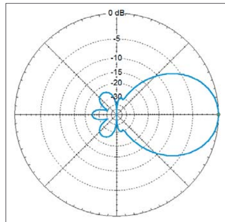
Bild 6: Im Freiraum simuliertes horizontales Richtdiagramm der 5-Element-50-Ω-Yagi
