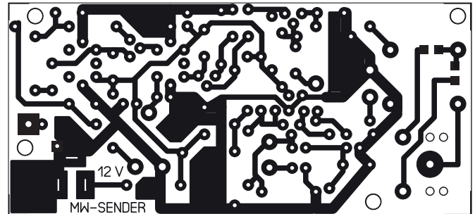
Bild 3: Layout des AM- Prüfgenerators; Abmessungen 87 mm × 40 mm, M 1:1
