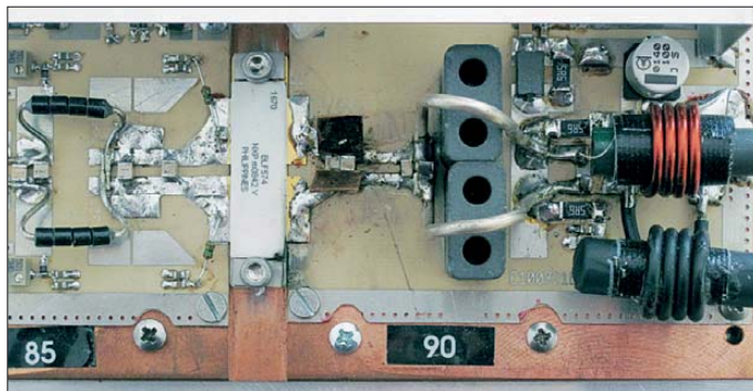
Bild 1: Auf einem Kühlkörper montiertes Breitbandverstärkermodule mit BLF574; links Eingangs-LC-Netzwerk, rechts Ausgangs-LC-Netzwerk, gefolgt von 1:4-Transformator und Balun
