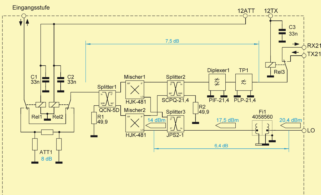
Bild 4: Schaltplan des Mischers; dieser arbeitet in Image- Reject-Schaltung und erreicht eine Spiegel- wellenunterdrückung von 24 dB.
