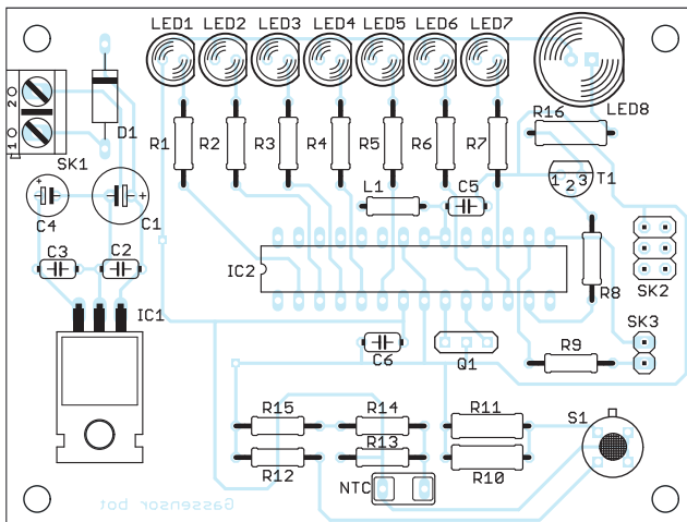
Bild 7: Bestückungsplan; die Leiterplatte des Gaswarngeräts ist 83,8 mm x 63,5 mm groß. Platinenlayouts stehen auf [6] zum Herunterladen bereit oder werden auf Wunsch per E-Mail versandt.
