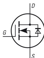
Bild 1: Innenschaltung des IXZH10N50LA/B
