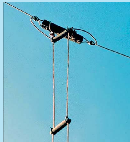
Bild 19: Mechanische Details am Mittenisolator mit 90° Drehung der Zweidrahtleitung zur Antennenebene
