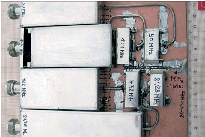
Bild 3: Teilansicht von Tiefpassfilterbank (links), Dämpfungsgliedern sowie 50-Ω- Mikrostreifenleitung (rechts, etwa Mitte) Fotos: DJ1EE
