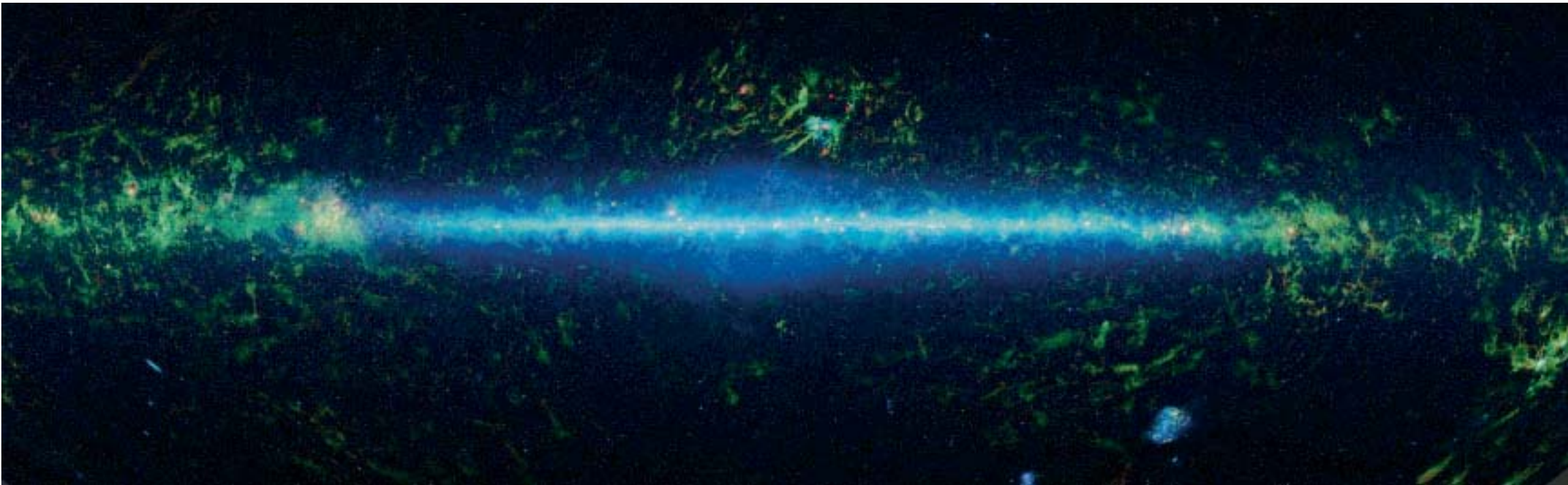
Der von „Wise“ abgetastete Himmel im infraroten Spektralbereich – projiziert auf zwei Dimensionen
