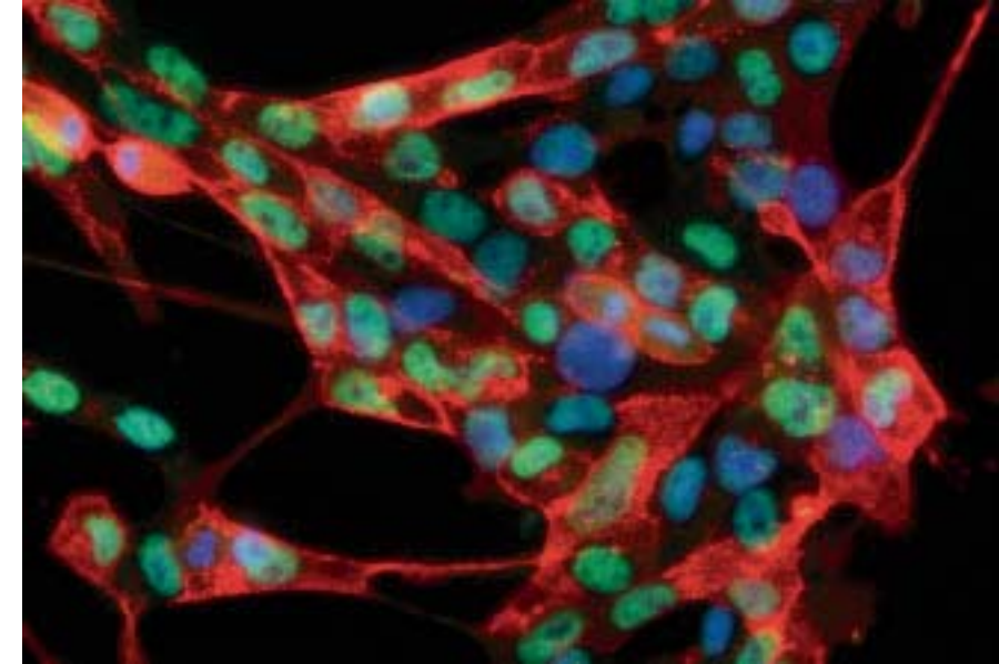
Eine Ansammlung von „iNSC“ – induzierte Nerven-Stammzellen.
