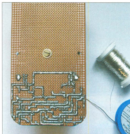
Bild 5: Ansicht der mit 0,2-mm-Kupferdraht auf der Unterseite hergestellten Leiterzüge
