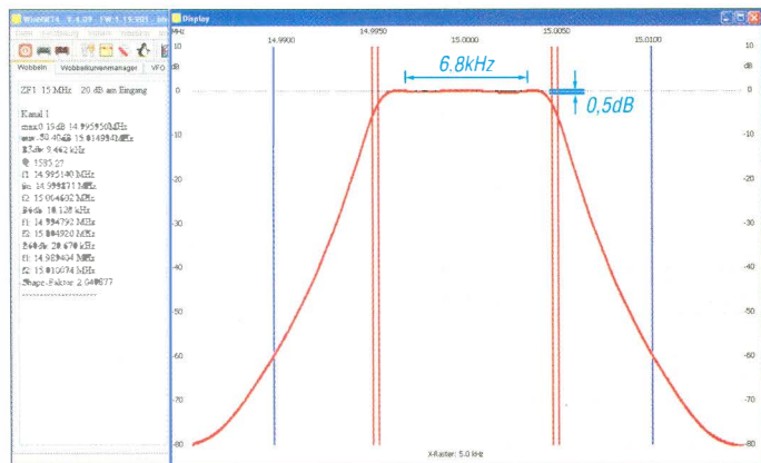
Bild 25: ZF1-Vorfilter 15 MHz, AM breit
