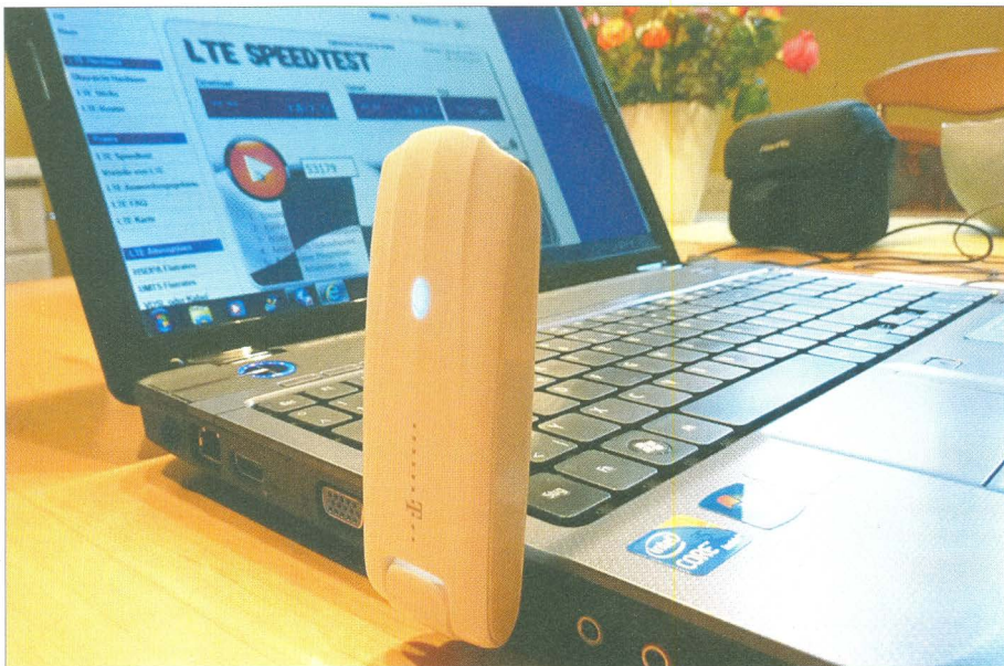
Bild 1: Notebook mit LTE/HSPA-Stick; dieser beherrscht HSPA auf 2,1 GHz mit maximal 42 MBit/s sowie LTE im Bereich 800, 1800 und 2600 MHz Foto: DK6ZD
