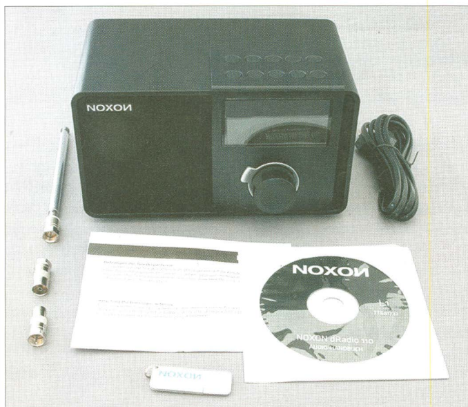
Bild 1: Lieferumfang; gedruckte Anleitung zur Antennenmontage, gesprochene Geräteanleitung (MP3-CD-ROM), Teleskopstabantenne, Adapter für Außenantennenanschluss, USB-Stift mit Sprachmenü, Netzkabel
