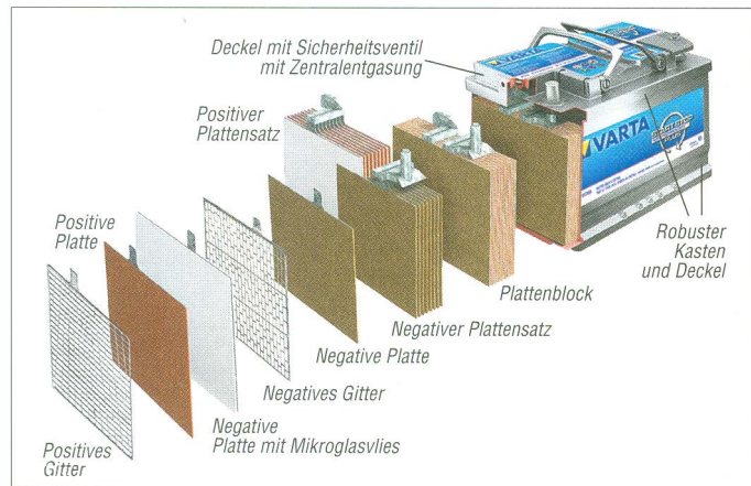
Bild 1: Montagezeichnung eines Vlies-/AGM-Akkumulators von Varta; das Vlies aus Mikroglasfasern legt die Schwefelsäure im Blei-Akkumulator fest.
