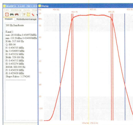
Bild 29: CW-Bandbreite 500 Hz
