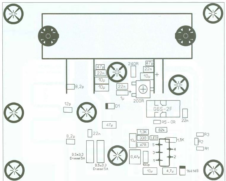
Bild 5: Bestückungsplan der Platine für die 70-cm-Endstufe; es sind beide Typen des Leistungsverstärkermoduls einsetzbar (80 mm × 100 mm, M 1:1).
