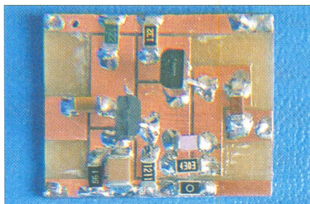
Bild 3: Breitbandverstärker mit SMD-Bauteilen auf einer gefrästen Leiterplatte
