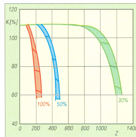
Bild 7: Erreichbare Lebensdauer (Zyklenanzahl Z) von Bleigel-Akkumulatoren in Abhängigkeit von der Entladungstiefe nach [5]
