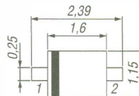
Bild 1: Pinbelegung und Abmessungen (SOD-323)
