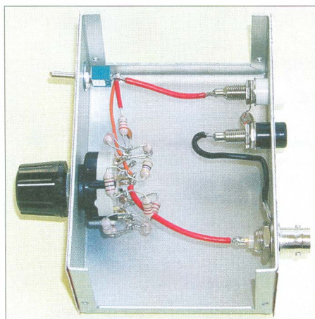
Bild 4: Anpassgerät mit abgenommenem Gehäusedeckel; zwischen Antennen- und Erdbuchse befindet sich eine Glühlampe als Überspannungsschutz.
