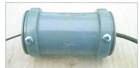
Bild 5: In einer HT-Rohrmuffe montierter Breitbandübertrager Fotos: DF1OG
