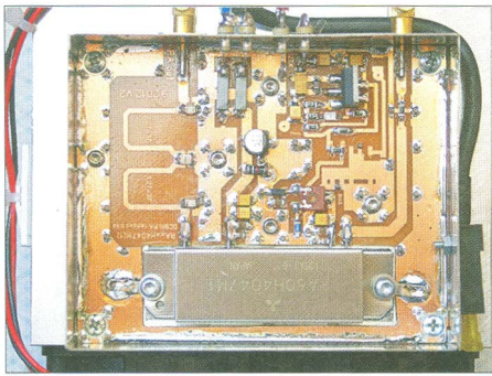
Bild 3: Das 60-W-Hybridmodul ermöglicht im Linearbetrieb etwa 40 W Ausgangsleistung bei einem IM3-Wert von 30 dBc.
