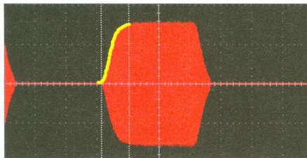
Bild 1: Typische Hüllkurve eines CW-Senders, aufgenommen mit einem digitalen Speicheroszilloskop; ein Kasten ist 10 ms breit. Gezeigt ist ein Dit bei Tempo 200 BpM. Der Anstieg dauert 9 ms (gelb nachgezeichnet). Screenshots: DM3DA
