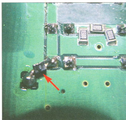
Nachgerüstete Schutzdiode am Empfänger-Eingang Foto: DL2EWN
