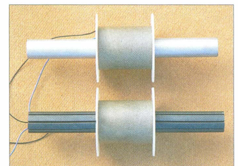
Bild 13: Induktionsspulen, oben mit Mu-Metall-Stabkern, unten mit K2006-Ferritstabkern ( d = 22 mm, l = 200 mm)
