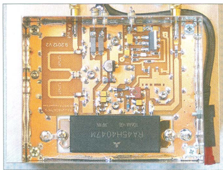
Bild 4: Endstufe mit 45-W-Modul; das Relais zur Zwangsabschaltung der Endstufe ist nicht aufgelötet. Fotos: DC8RI
