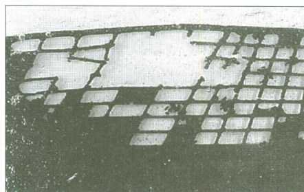
Bild 6: Nach fünf Jahren in einem PKW war der Stromableiter der positiven Elektrode durch Gitterkorrosion zerfressen. Quelle [12]
