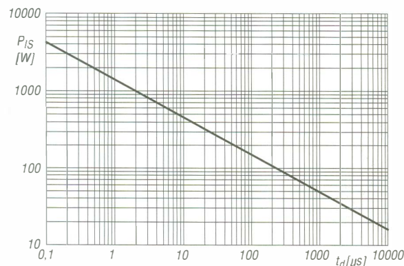
Bild 4: Abhängigkeit der Spitzenimpulsleistung P_{IS} von der Impulsdauer t_d bei einer Impulsform gemäß Bild 5
