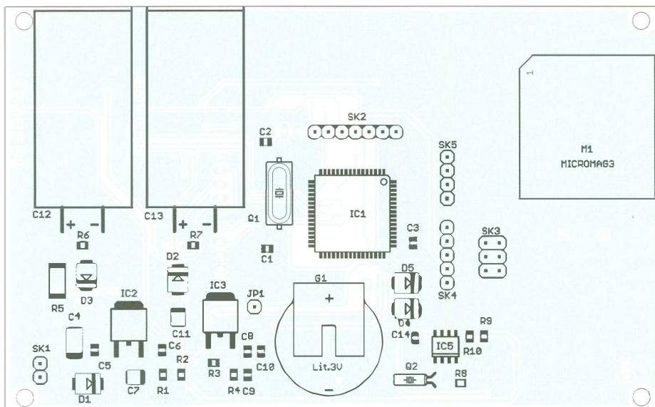
Bild 4: Bestückungsplan der Magnetometerplatine; die Bestückung erfolgt fast ausschließlich mit SMD-Bauelementen; Abmessungen 123 mm × 75 mm, M 1:1
