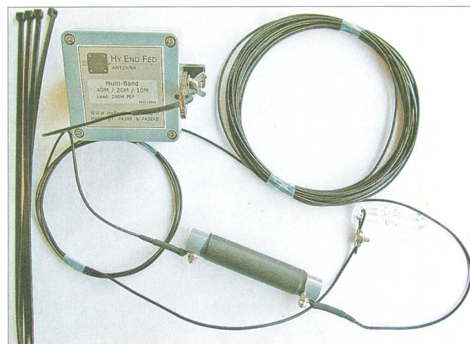
Bild 2: Packungsinhalt der Hy End Fed Antenna, Variante Multiband Tri Band
