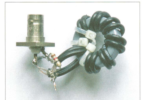
Bild 9: Dieser Transformator von 12 \Omega auf 50 \Omega passt ggf. sogar zwischen Autodach und Himmel. Fotos: DL4NO
