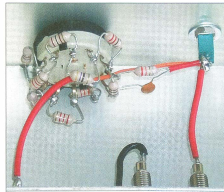
Bild 3: Beschaltung des Stufenschalters und des Kippschalters
