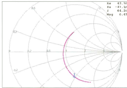
Bild 7: Ein 220-pF-Kondensator in Serie verschiebt den Resonanzpunkt, ohne den Realteil der Impedanz wesentlich zu ändern.
