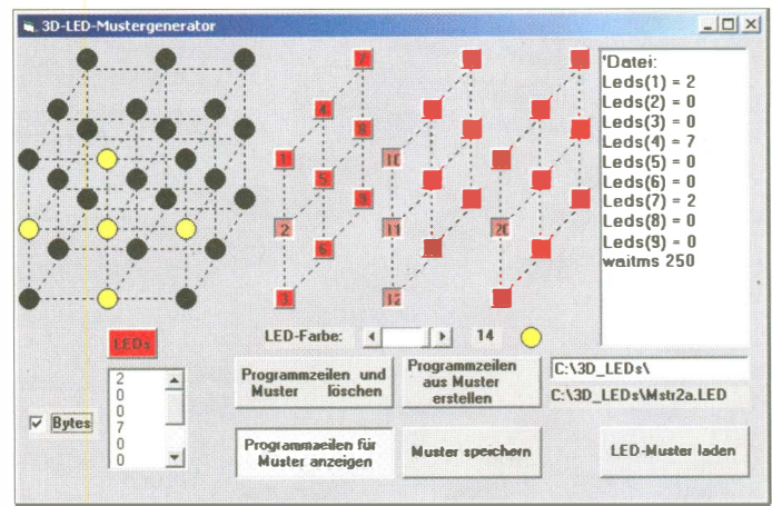
Bild 4: Screenshot des 3-D-LED-Muster- generators, der als Hilfsmittel für die Ermittlung der für die Darstellung der Muster/Figuren wichtigen Pro- grammzeilen der Ansteuer-Firmware des Mikrocontrollers dient
