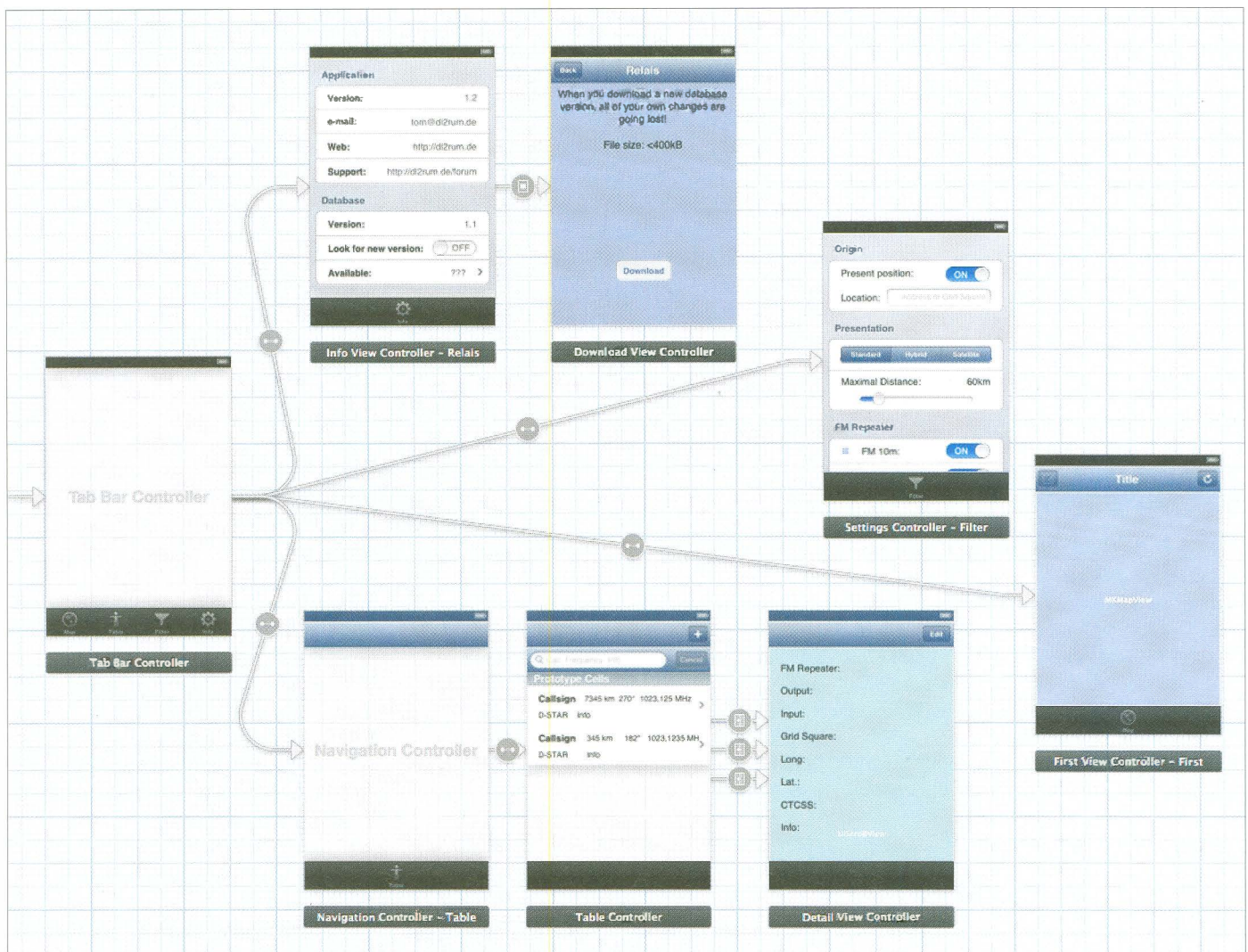
Bild 1: Storyboard der iOS-App „Relais“: Jede Ansicht der Benutzeroberfläche wird erst im Storyboard erstellt und dann untereinander verknüpft.
