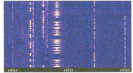
Bild 2: Das Wasserfallspektrum eines WebSDR-Empfängers zeigt die Tastklicks als Querlinien am Anfang und am Ende der Signale. Die meisten der gezeigten Stationen produzieren nur geringe Klicks, aber das Signal bei 14,014 MHz sind 1 kHz breit. Zum Vergleich: Der Bandplan sieht für Telegrafiesignale nur 200 Hz Signalbreite vor.
