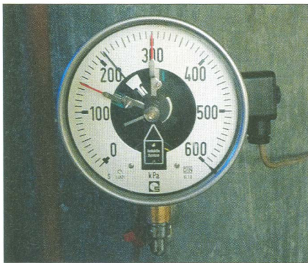
Bild 1: Kontaktmanometer mit den beiden auf beliebige Werte einstellbaren Schaltkontakten Foto: DM4TR
