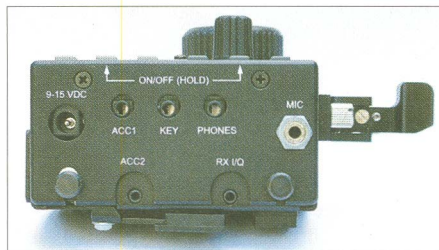
Bild 2: Außer der/den Antennenbuchse(n) befinden sich alle anderen an der linken Geräte-seite. Wer viel Peripherie anschließen möchte, sollte zum Zubehör-Kabelset KX-KCPT mit abgewinkelten Klinkensteckern greifen, das u. a. ein geteiltes Kabel für ACC2 enthält. Unten im Bild der linke der hereingeklappten Aufstellbügel.
