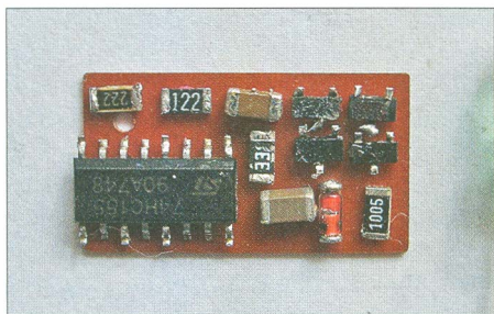
Bild 3: SMD-Bauteile werden auf der nicht kaschierten Seite einer einseitigen Platine an den Gehäusen aufgeklebt. Die Bauteile sind hier noch unverdrahtet.
