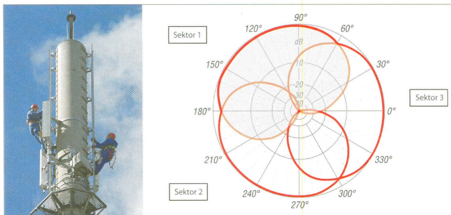
Bild 4: Je Zelle (Sektor) steht bei 20 MHz Bandbreite eine Ressource von bis zu 170 MBit/s zur Verfügung. Rechts im Bild ist das horizontale Strahlungsdiagramm der drei Sektorentennen zu sehen.
