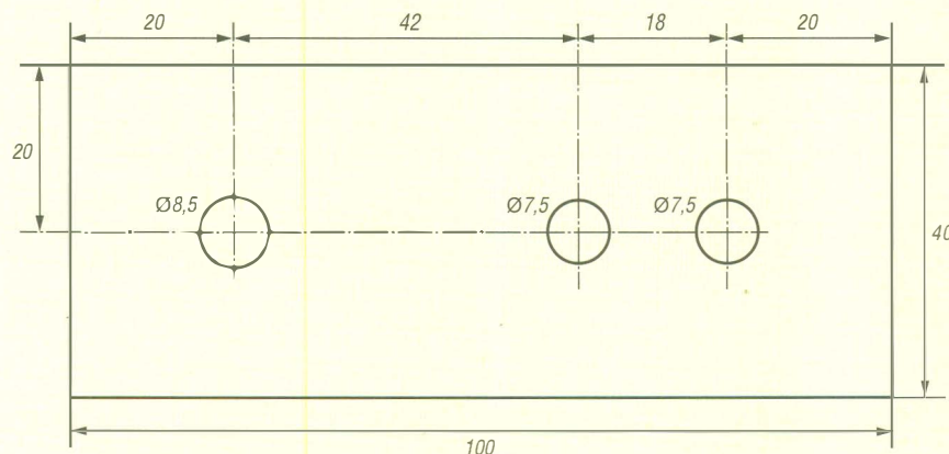
Bild 6: Bohrplan der Rückseite
