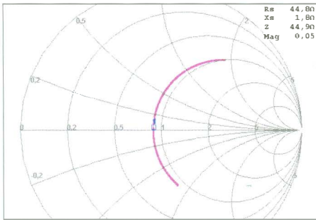
Bild 4: Gleiche Messung wie in Bild 3, jedoch mit kürzerem Kabel – der Kurvenzug hat nun überall annähernd gleichen Wirkwiderstand.
