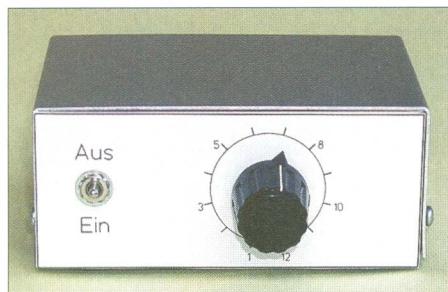
Bild 1: Musteraufbau des einfachen Anpassgeräts für Empfangsantennen
