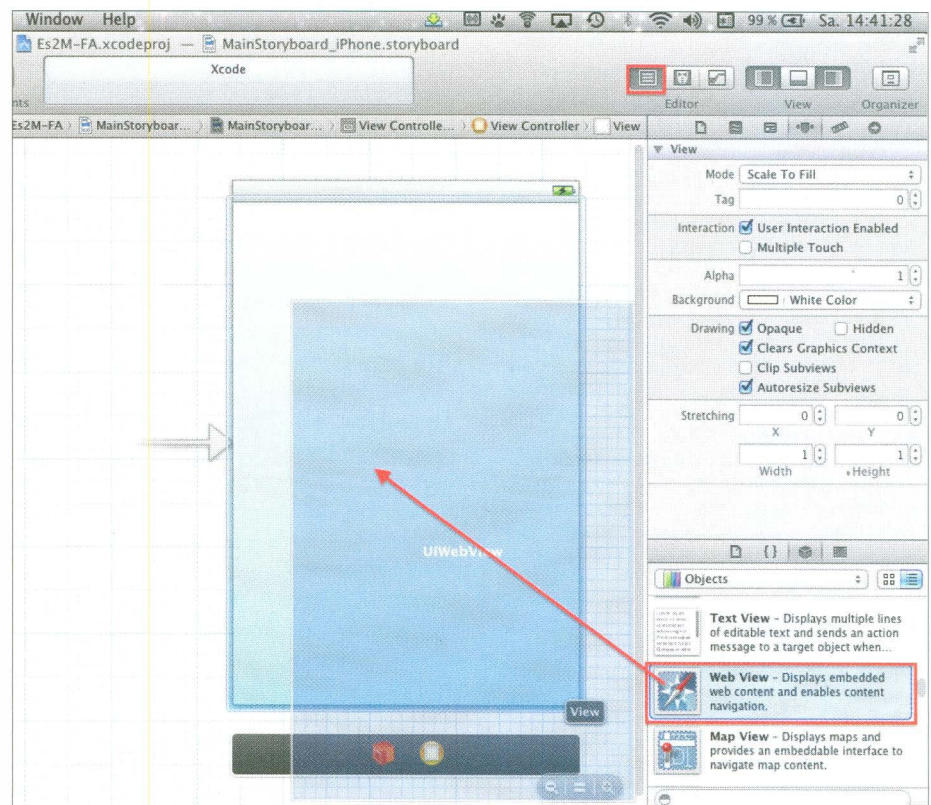
Bild 5: Erstellung der Benutzeroberfläche im iPhone-Storyboard
