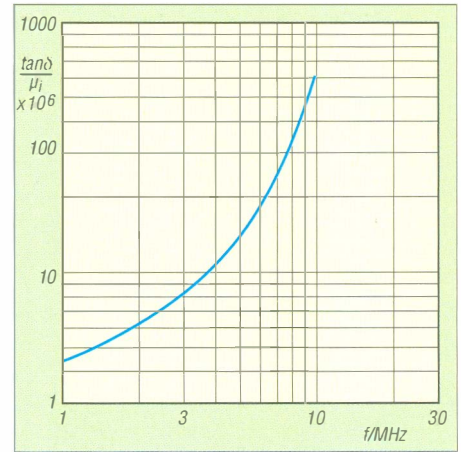
Bild 9: Der bezogene Verlustfaktor als Funktion der Frequenz
