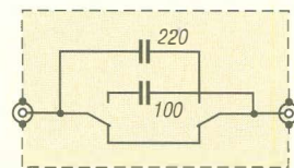
Bild 8: Schaltung des Anpassglieds; die Kondensatoren haben 50 \Omega bzw. 100 \Omega Impedanz (Beispiele für 14 MHz) und werden in Serie ins Koaxialkabel eingeschleift.
