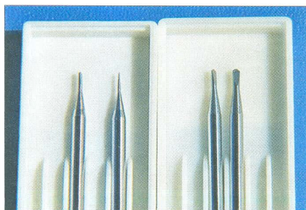
Bild 2: Speerbohrer in vier Größen für unterschiedlich breite Fräsbahnen Fotos: Heerde
