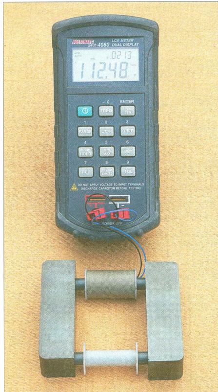
Bild 1: Versuchsanordnung zur Wirkung der Scherung. Erst im geschlossenen magnetischen Kreis zeigt die unterschiedliche Permeabilität der Zylinderkerne Wirkung.
