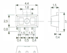
Bild 2: Pinbelegung (SOT-89) und Abmessungen
