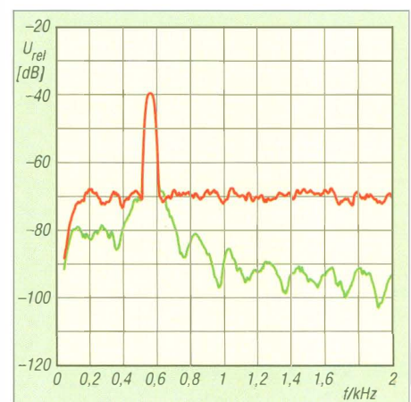
Bild 8: Wirkung der Geräuschunterdrückung, NR (rot ohne, grün mit) in Maximalstellung, bei schwachen CW-Signalen sehr nützlich
