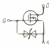
Bild 1: Innenschaltung des RD01MUS2
