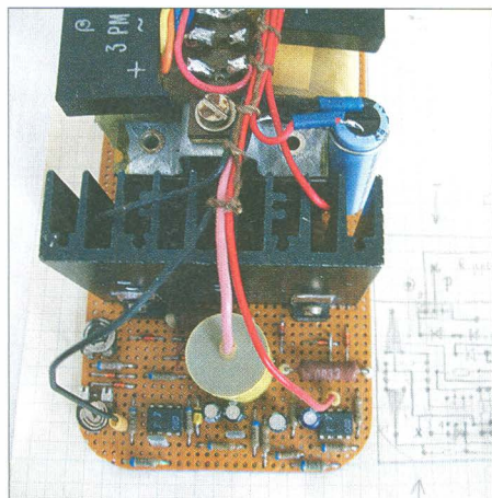
Bild 4: Auf der Oberseite sind die Bauteile dicht gepackt angeordnet. Fotos: Quietzschn
