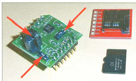
Bild 5: Das Modul Micromag 3 hat für die x-, y- und z-Richtung je einen Sensor. Daneben liegt das Modul BOB-00544 für den Anschluss der microSD-Karte.
