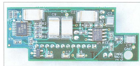
Bild 9: Das optionale Modul für zwei Roofing-Filter sieht etwas ungewöhnlich aus, enthält aber statt passiver Filter DSP-Filter mit ICs.
