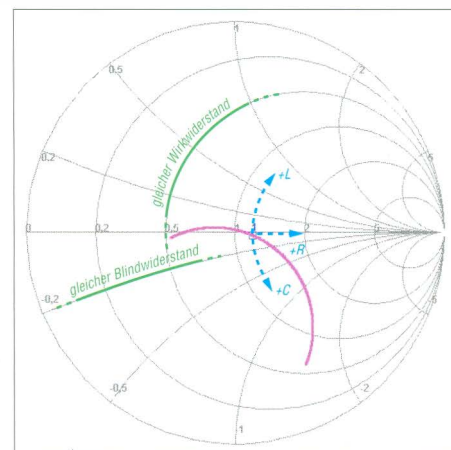
Bild 3: Smith-Diagramm einer 20-m-Mobilantenne, das linke Ende der violetten Kurve liegt bei 14,0 MHz, das untere bei 14,35 MHz.
