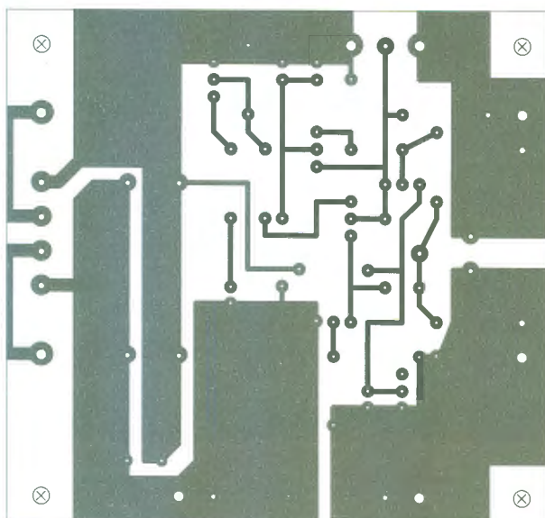
Bild 3: Layout der einseitig kaschierten Platine; Abmessungen 80 mm \times 75 mm, M 1:1
