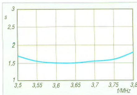
Bild 8: Gemessener SWV-Verlauf der stark verkürzten Vertikalantenne im 80-m-Band
