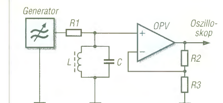
Bild 3: Bei der gepufferten Schaltungsvariante erfolgt die Dämpfung hauptsächlich durch die Reihenschaltung aus R1 und Generatorinnenwiderstand.
