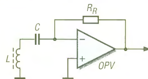
Bild 10: Beim Einsatz der Induktionsspule im Reihenschwingkreis wird der Verstärkungsfaktor vom Scheinwiderstand Z bestimmt, bei Resonanz gilt Z_0 = R_v .
