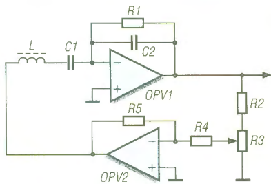
Bild 15: Schaltung zur Entdämpfung von Serienresonanzkreisen
