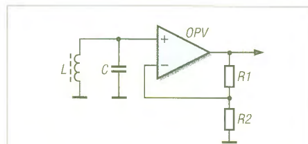
Bild 7: Hochohmige Ankopplung des Parallelschwingkreises an den OPV
