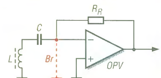
Bild 12: Der OPV hat für den Reihenschwingkreis aus L und C fast die gleiche Wirkung wie die gestrichelt eingezeichnete Brücke Br.
