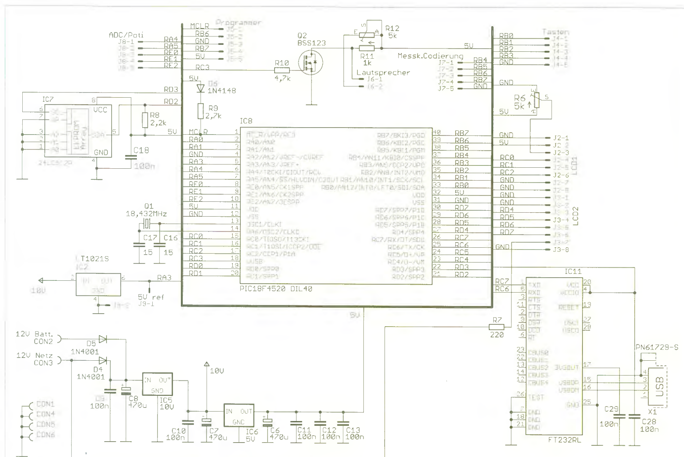
Bild 3: Schaltplan der Hauptplatine (Teil 1), Digitalteil
