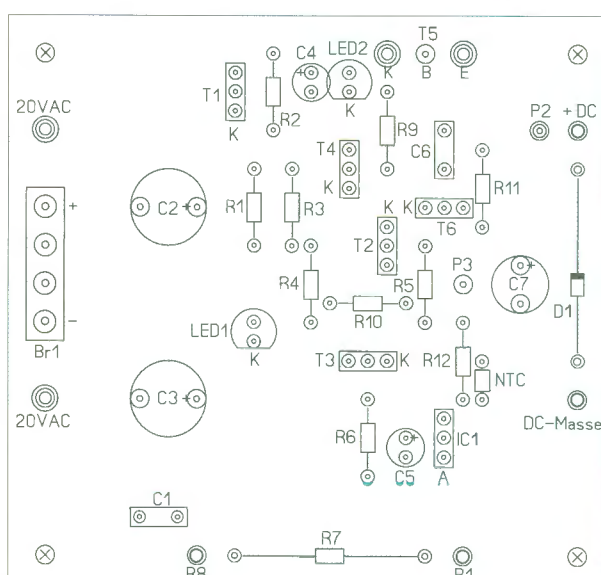
Bild 4: Bestückungsplan der Leiterplatte
