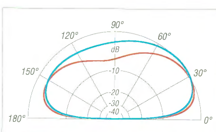
Bild 6: Simuliertes Strahlungsdiagramm der Antenne mit Sperrkreisresonanz bei 2,6 MHz über realem Grund ( \sigma = 0,005 \text{ S/m} , \epsilon_r = 13 ) bei f_{\text{Res}} = 3,65 \text{ MHz} (blau) und f_{\text{Res}} = 1,85 \text{ MHz} (rot)
