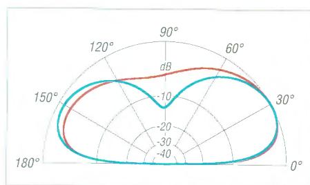
Bild 4: Simuliertes Strahlungsdiagramm der Antenne mit Sperrkreisresonanz bei 3,4 MHz über realem Grund ( \sigma = 0,005 \text{ S/m} , \epsilon_r = 13 ) bei f_{\text{Res}} = 3,65 \text{ MHz} (blau) und f_{\text{Res}} = 1,85 \text{ MHz} (rot)
