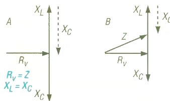
Bild 11: Zeigerdiagramm der Widerstände der Reihenschaltung aus L , C und R_v im Resonanzfall (A); die Beträge von X_L und X_C sind identisch. Sie heben sich auf, der Scheinwiderstand Z entspricht R_v . Für alle anderen Fälle sind die Beträge von X_L und X_C unterschiedlich (B).
