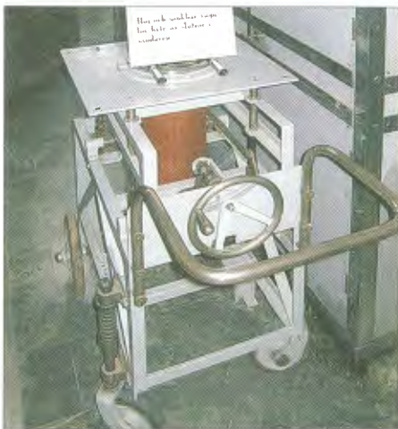
Höhenverstellbarer Wagen zum Austausch der Senderöhre CAT14
