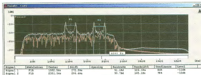
Bild 4: Der Wavecom-Classifier hat zwei F1B-Signale bei 28 100 kHz klassifiziert. Bilder 1 bis 4: DK2OM mit Wavecom W61, W-Code und Perseus
