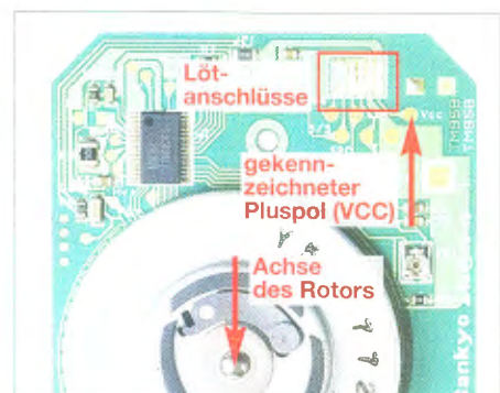
Bild 1: An die zur Ansteuerung genutzten Lötanschlüsse war im Originalzustand ein Flachbandkabel angelötet. Bei einigen Diskettenlaufwerken ist die Rotorachse festgeschraubt, bei anderen lässt sich der Rotor einfach abziehen. Foto: Red. FA
