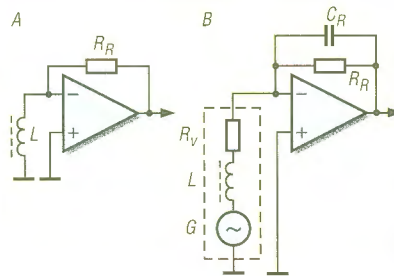
Bild 17: So wird die Induktionsspule stromgekoppelt an den OPV geschaltet. Die Schaltungsfunktion wird anhand des Ersatzschaltbildes deutlich. Durch C_R bekommt die Schaltung ein ausgeprägteres Tiefpassverhalten.
