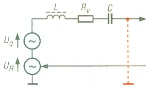
Bild 16: Wirkungsprinzip der Schaltung in Bild 15; die Spannungs- und Strompeile von U_q und U_R sind phasengleich. Die bedämpfende Wirkung von R_v wird minimiert.
