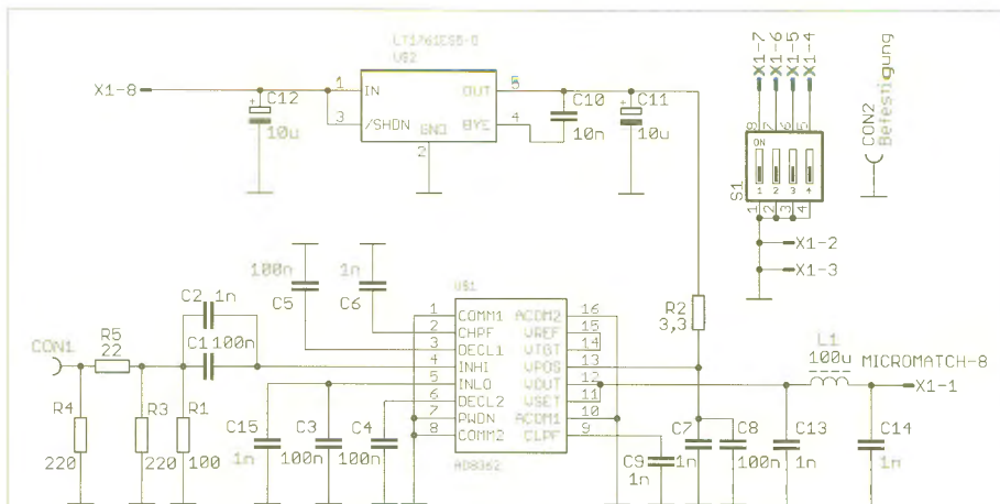
Bild 5: Schaltplan des Messkopfs mit dem AD8362
