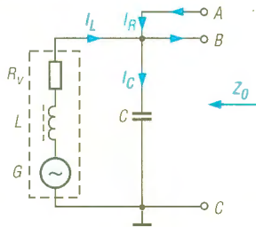
Bild 9: Die phasenrichtige Spannungs-rückführung bewirkt einen Rückgang des Spulenstroms. Z_0 vergrößert sich und R_v verringert sich scheinbar.
