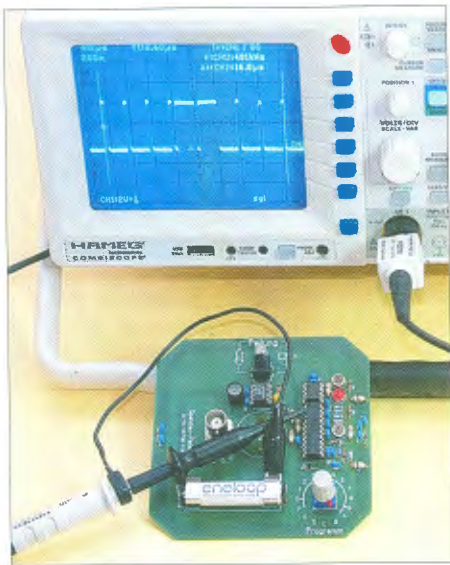
Bild 1: Messung der Debug-Information beim Spandau-Peiler V6.3 am Pin 2 von IC1 in Stellung „B“ des HEX-Schalters S2
