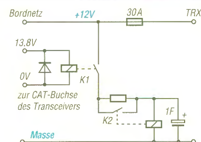
Bild 2: Diese einfache Schaltung verhindert den ersten Ladestromstoß durch den Powercap. Die Ansteuerung erfolgt über die CAT-Buchse des Transceivers.
