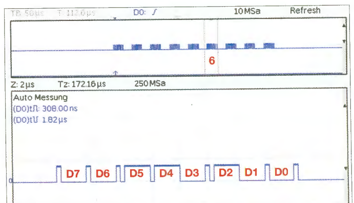
Bild 2: Ausgabe der neunmal aufgerufenen Debug-Routine beim Spandau-Peiler, im sechsten Datenpaket steht der aktuell gemessene HF-Wert: 0b00110100 = 0x34 des logarithmischen Verstärkers IC2. Die Daten werden mit dem MSB zuerst (D7) übertragen. Foto und Screenshot: DC7GB
