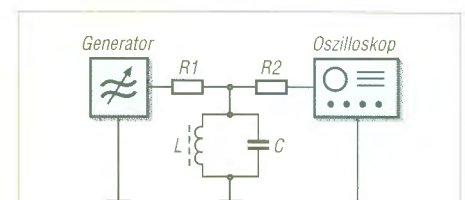
Bild 2: Schaltung zur Ermittlung der Resonanzfrequenz des Schwingkreises; der Wert von R1 und R2 sollte einige zehn Kilohm bis einige 100 Kilohm betragen.
