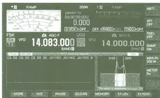
RTTY-Decoder
