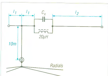
Bild 5: Abmessungen der Antenne bei Variation des Sperrkreises
