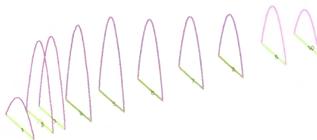
Bild 3: Stromprofil der 10-Element-28- \Omega - Yagi nach DK7ZB
