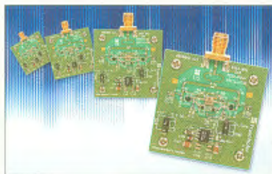
Prototypen eines SAW-Oszillators mit einer Ausgangsfrequenz von 4,884 GHz
