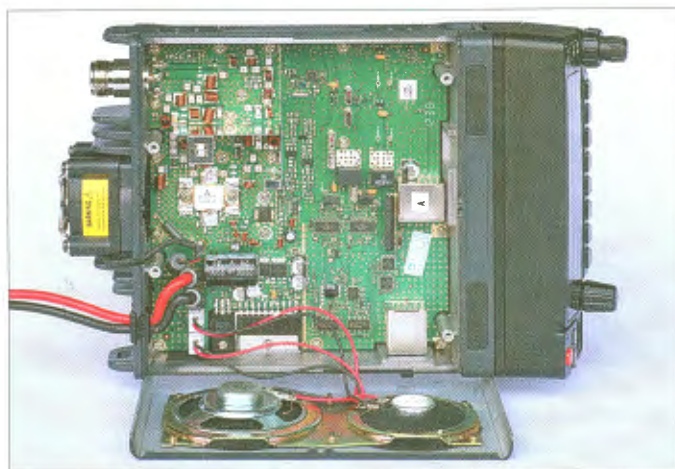
Bild 4: Blick auf die Platine des AMT-920-UV; das Gerät hat zwei eingebaute Lautsprecher und einen dritten im Handmikrofon.
