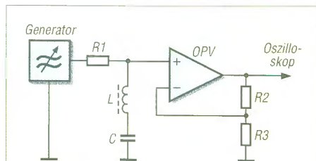
Bild 5: Die Reihenschaltung einer Spule mit sehr hoher Induktivität und einem Messkondensator bietet sich zur Ermittlung der Resonanzfrequenz an.
