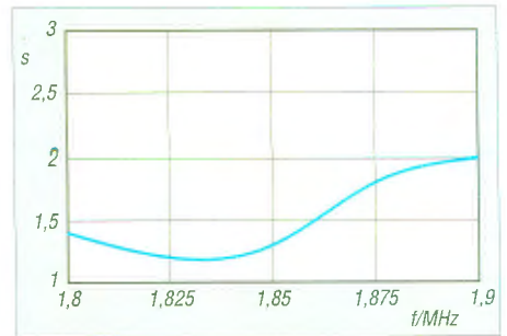
Bild 9: Gemessener SWV-Verlauf der stark verkürzten Vertikalantenne im 160-m-Band
