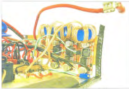
Bild 7: Gleichspannungswandler
