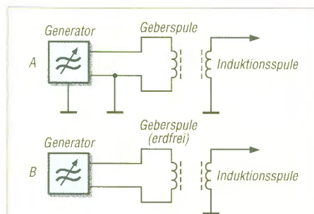
Bild 6: Vorteilhafte Signaleinspeisung durch induktive Kopplung
