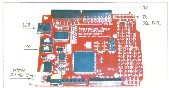
Bild 4: Das Seeeduino Mega Modul basiert auf dem ATmega1280 . Der Schalter für die Höhe der Betriebsspannung ist auf 5 V einzustellen.
