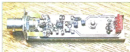
Bild 7: Messkopf mit dem AD8307; der DIP-Schalter wurde weggelassen, stattdessen dienen kleine Zinnbrücken zur Codierung.
