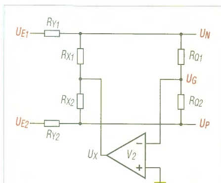
Bild 2: Eingangsstufe des Differenzverstärkers aus Bild 1
