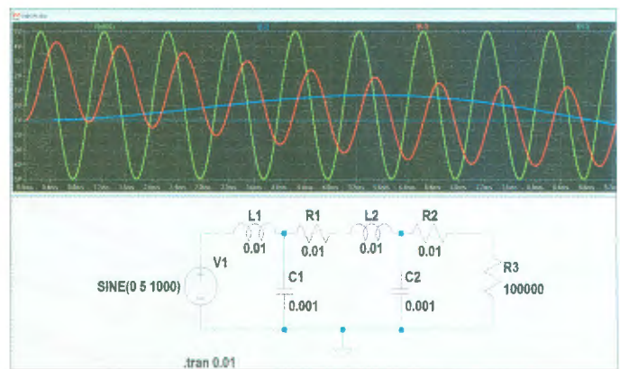
Bild 7: Mit Programmen wie LTSpice lassen sich elektronische Schaltungen direkt am PC analysieren. So kann man sich auch das Verhalten von Übertragungsleitungen veranschaulichen – ganz ohne komplizierte Formeln!
