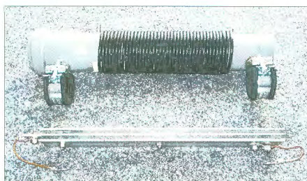
Bild 2: Aufbau eines Sperrkreises mit vergrößertem Kondensator
