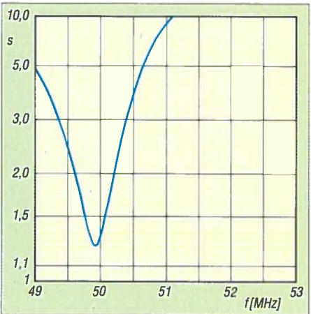
Bild 11: Simuliertes SWV einer 3-Element-NBS-Yagi mit Z = 12 \Omega
