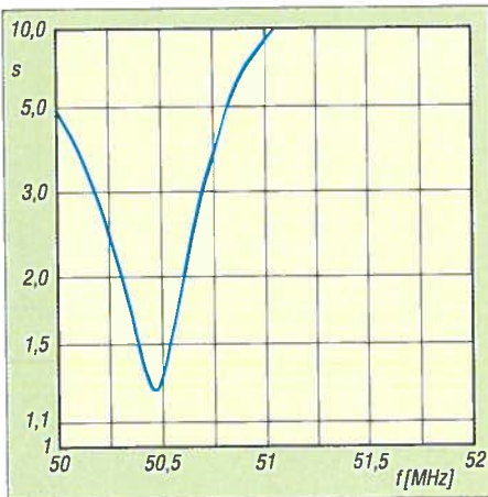
Bild 13: Simuliertes SWV einer 4-Element-Ban(d)tenna mit Z = 12 \Omega
