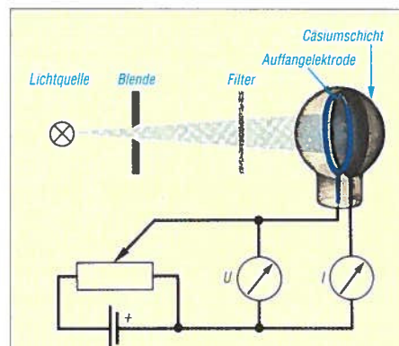
Bild 2: Der Versuchsaufbau zum fotoelektrischen Effekt [2]
