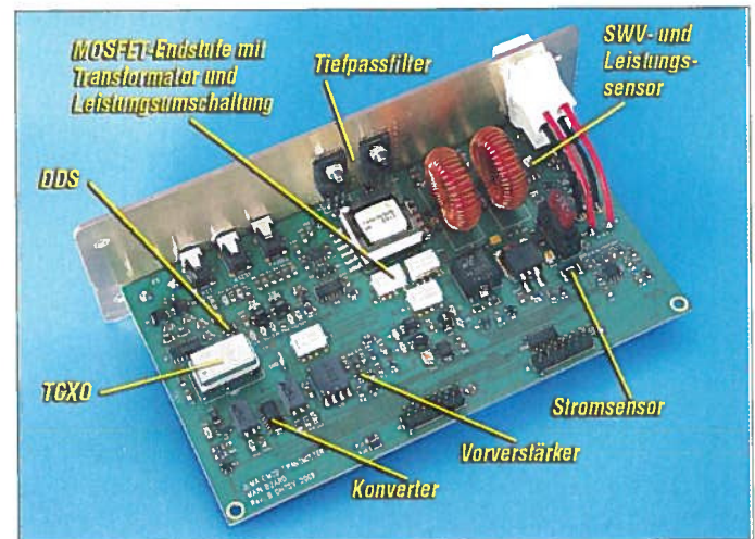
Bild 2: Hauptmodul mit Endstufe und Tiefpassfilter
