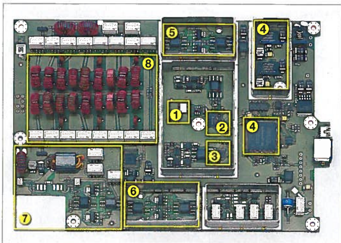
Bild 7: Innenleben des ZS-1; 1 Taktfrequenz- generator 2 A/D-Umsetzer 3 D/A-Umsetzer 4 FPGA und Spannungsquelle 5 Eingangsvor- verstärker (LNA) 6 Ausgangs-LNA 7 Vortreiber/Endstufe 8 Filter
