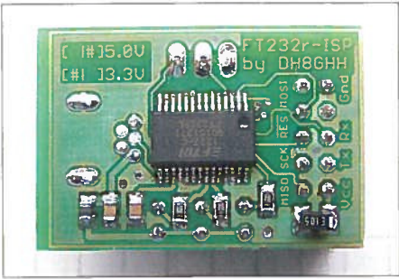
Bild 7: Unterseite des Programmieradapters mit den aufgelöteten SMD-Bauteilen
