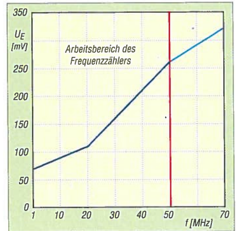
Bild 4: Eingangsempfindlichkeit des Frequenzzählers
