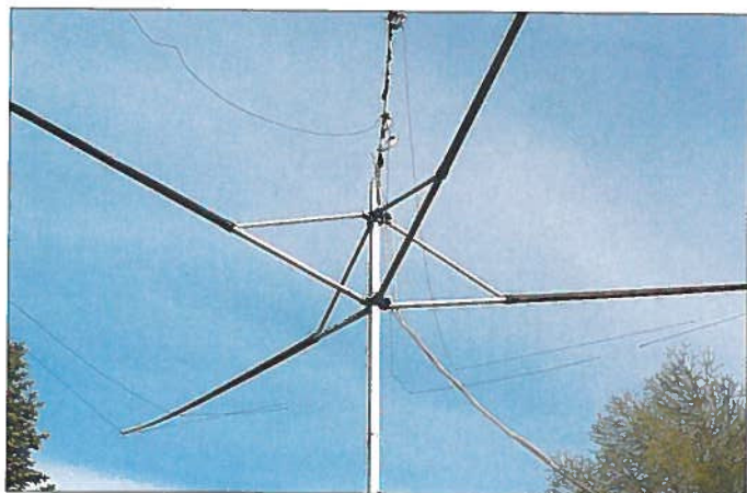
Bild 1: Zwei 3-Element- Antennen für 14 MHz und 21 MHz mit einer Wäschespinne als zentraler Stütze
