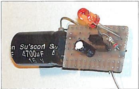
Bild 1: Aufbau des LED-Blitzers der Version 2 auf einer Universalplatte Foto: Urbanneck
