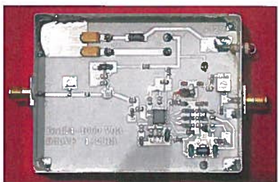
25-GHz-Frequenzteiler im Weißblechgehäuse
