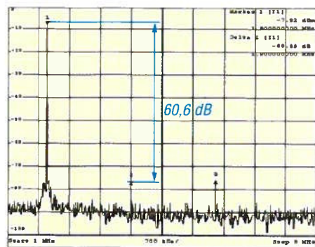
Bild 9: Oberwellenspektrum auf 160 m
