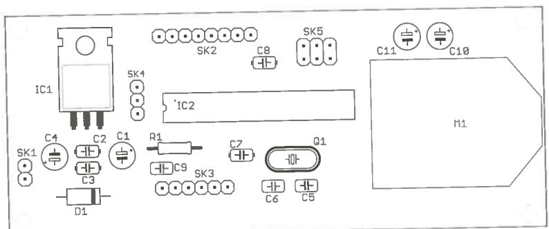
Bild 8: Bestückungsplan der Controllerbaugruppe für die Sensoren; Abmessungen 104 mm × 42 mm, M 1:1; die Platinen sind bei [4] erhältlich.
