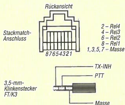
Bild 11: Belegung der Steckverbinder; bei den nicht dargestellten Cinch- und Hohlsteckerbuchsen liegt der Massekontakt außen.
