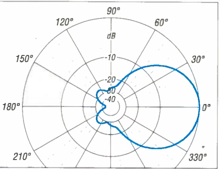
Bild 19: Simuliertes Horizontales Freiraum-Richtdiagramm einer 5-Element-Ban(d)tenna nach Bild 4; äußerer Ring 7,1 dBd
