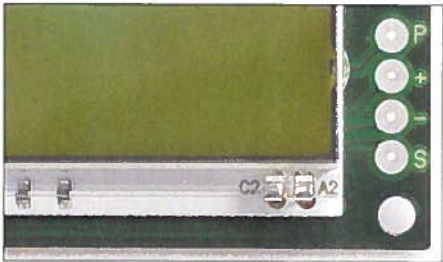
Bild 5: Die Kontaktflächen zum Programmieren sind auch auf der Vorderseite der Platine zugänglich und hier entsprechend ihrer Funktion beschriftet.
