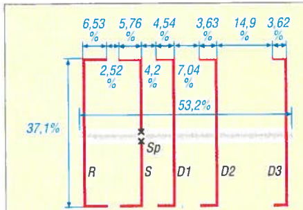
Bild 4: Aufbau einer 5-Element-Ban(d)tenna; die Prozentangaben unter den Maßzahlen sind auf die mittlere Betriebswellenlänge \lambda bezogen; Elementdurchmesser ist hier 0,1 % \lambda !
