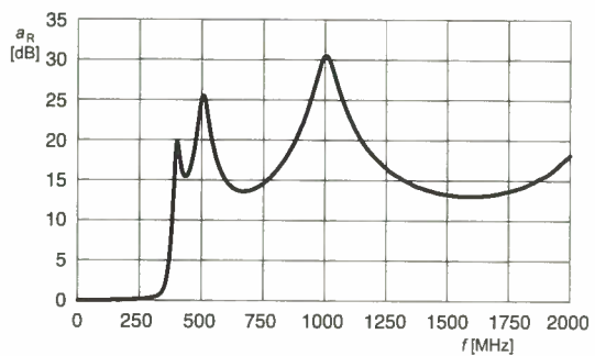
Bild 8: Abhängigkeit der Reflexion a_R eines PHP-400 von der Frequenz f bei P_E = 0 dBm
