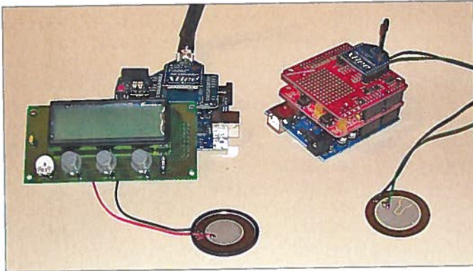
Bild 1: In der Alarmanlage kommen verschiedene Sensoren und ein Arduino-Board als Zentrale zum Einsatz.
