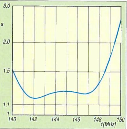
Bild 18: Simuliertes SWV einer 5-Element-Ban(d)tenna nach Bild 4
