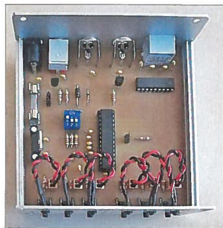
Bild 8: Prototyp der Stackmatch-Steuerung im geöffneten Gehäuse; die LEDs sind hier mittels Stifteisen und -buchsen angeschlossen.
