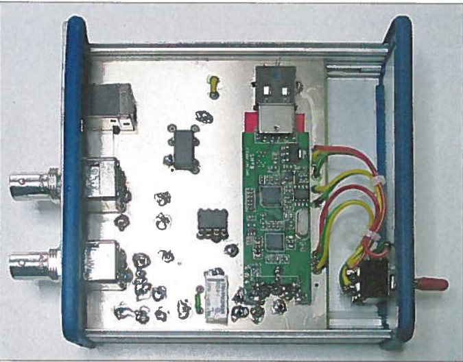
Bild 1: Geöffneter softwaredefinierter Empfänger mit dem DVB-T-Stick rechts
