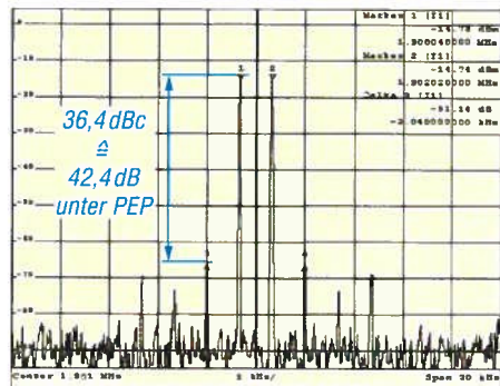
Bild 10: 160-m-Sendespektrum bei Zweitonaussteuerung, 2 kHz Trägerabstand
