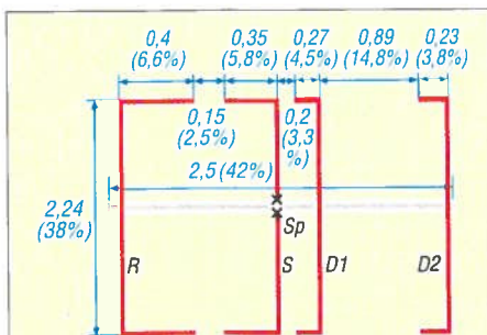
Bild 3: Aufbau einer Ban(d)tenna für das 6-m-Band; die Prozentangaben unter den Maßzahlen sind auf die mittlere Betriebswellenlänge \lambda bezogen; Elementdurchmesser ist hier 0,1 % \lambda !
