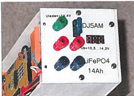
Bild 3: Frontplatte des Akkupacks mit Anschlussbuchsen, Sicherung und Anzeige
