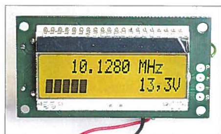
Bild 1: Das zweizeilige LC-Display des Moduls zeigt in der oberen Zeile die Frequenz und optional in der unteren Zeile zwei Gleichspannungswerte an, links als Balken, rechts als Ziffernfolge mit Maßeinheit.
