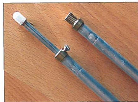
Die drei Segmente des Viertelwellenstrahlers sind jeweils etwa 1 m lang und lassen sich gut im Kofferraum transportieren. Zur Abstimmung dient das verschiebbare oberste Antennensegment.
