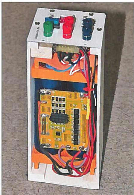
Bild 1: Blick in das geöffnete Gehäuse des Akkupacks mit der BMS-Platine vorn
