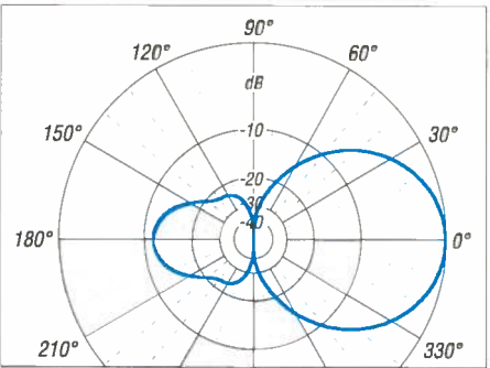
Bild 12: Simuliertes Horizontales Freiraum-Richtdiagramm einer 3-Element-NBS-Yagi mit Z = 16 \Omega ; äußerer Ring 6,8 dBd
