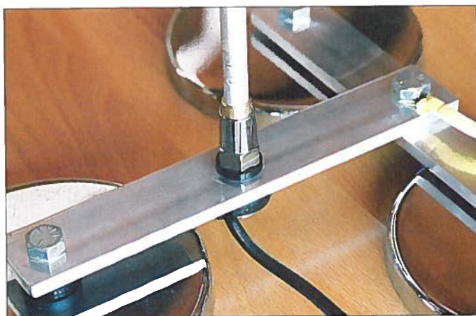
Dank 3/8-Zoll-Gewinde lässt sich der Mobilstrahler von Winkler mit einem großen Magnetfuß verwenden.
