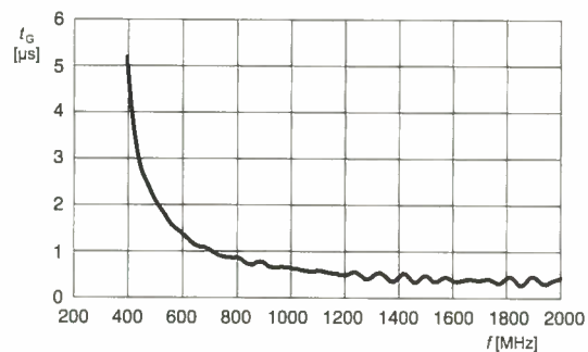
Bild 9: Abhängigkeit der Gruppenlaufzeit t_G eines PHP-400 von der Frequenz f bei P_E = 0 dBm
