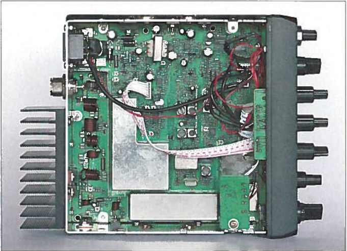
Das Funkgerät hat etwa Autoradioformat; am linken Bildrand sind die auf der Rückseite montierten Kühlrippen zu sehen.
