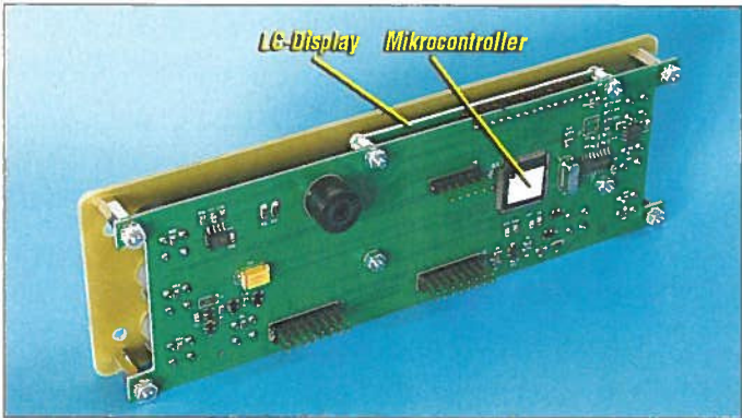
Bild 3: Rückseite der Frontplatte mit dem Mikrocontroller Werkfotos
