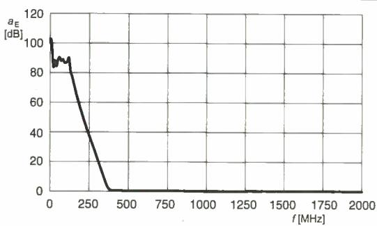
Bild 7: Abhängigkeit der Einfügedämpfung a_E eines PHP-400 von der Frequenz f bei P_E = 0 dBm
