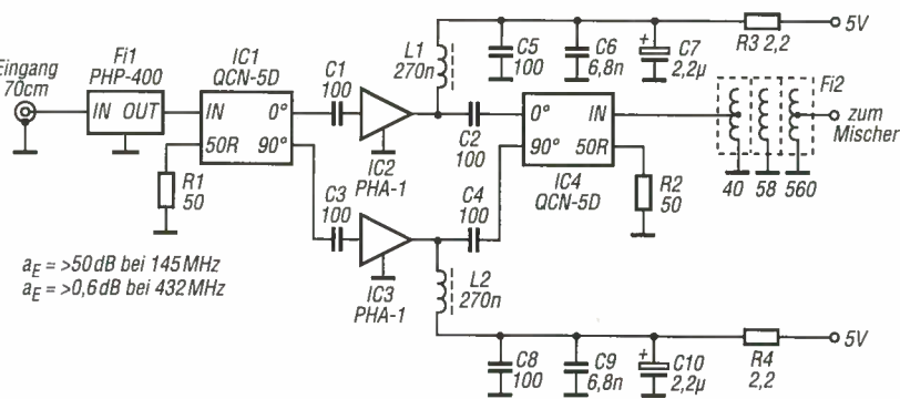
Bild 10: Eingangsverstärker des Empfangsteils für den 70-cm-Transverter IRHX4011 nach [1], hier mit einem PHP-400 als Fi1
