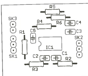
Bild 7: Bestückungsplan des Ladungsverstärkers; Abmessungen 39 mm × 32 mm, M 1:1
