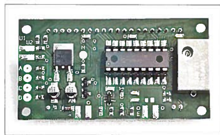
Bild 2: Bis auf das Display befinden sich alle Bauelemente des Frequenzzählers auf der Rückseite des Moduls. Dort sind auch sämtliche Anschlüsse zugänglich.
