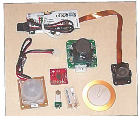
Bild 2: Auswahl geeigneter Sensoren für Alarmanlagen Fotos: Sander
