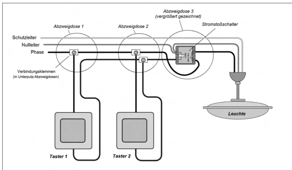
Abb. 52: Bildlich dargestelltes Beispiel der Anschlüsse eines Stromstoßschalters
