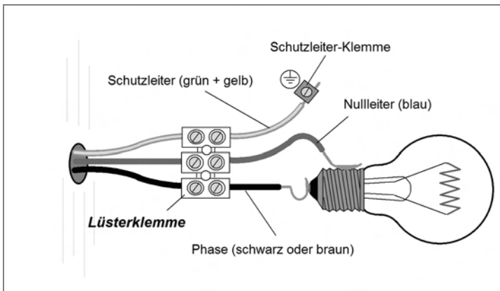
Abb. 12: Prinzip des Netzanschlusses einer Lampe
