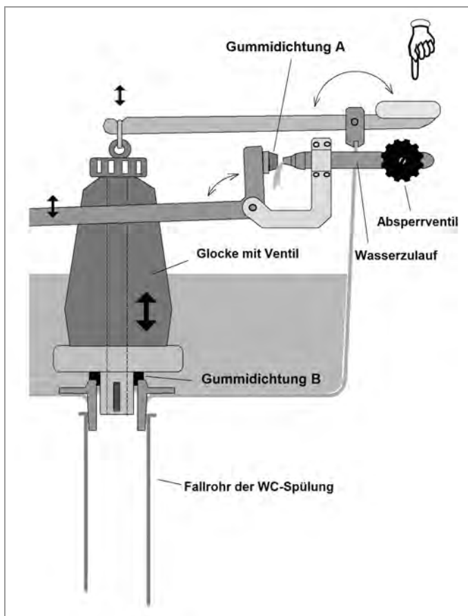
Abb. 25: Wenn eine WC-Spülung undicht wird, liegt die Ursache darin, dass entweder die Gummidichtung A oder die Gummidichtung B verschmutzt, verkalkt oder verschlissen sind.
