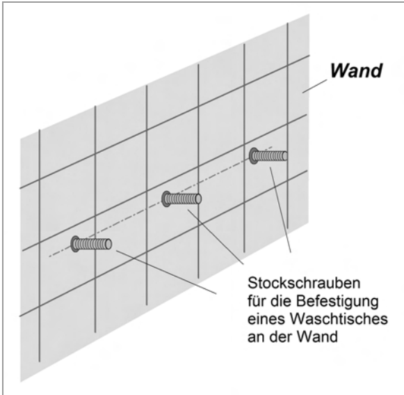
Abb. 96c: Größere Porzellan-Waschtische müssen mit drei Stockschrauben (in Wanddübel) an der Wand befestigt werden.
