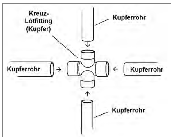
Abb. 82: Kreuzförmiges Lötfitting
