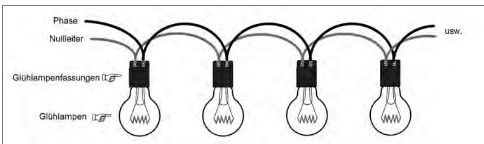
Abb. 13: Lampenkette im Parallelbetrieb
