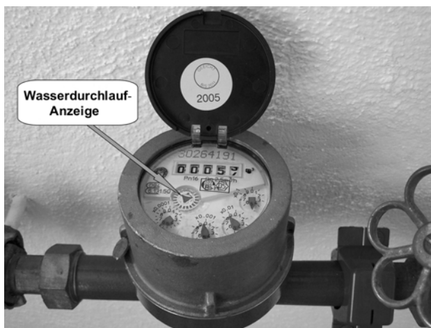
Abb. 3: Am Wasserzähler können Sie kontrollieren, ob Ihr Wasserleitungs-Hausnetz perfekt dicht ist.
