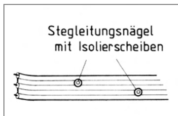
Abb. 73: Bevor eine Unterputz-Stegleitung (Flachleitung) definitiv eingeputzt wird, muss sie an einigen Stellen z. B. mittels speziellen Stegleitungsnägeln befestigt werden.
