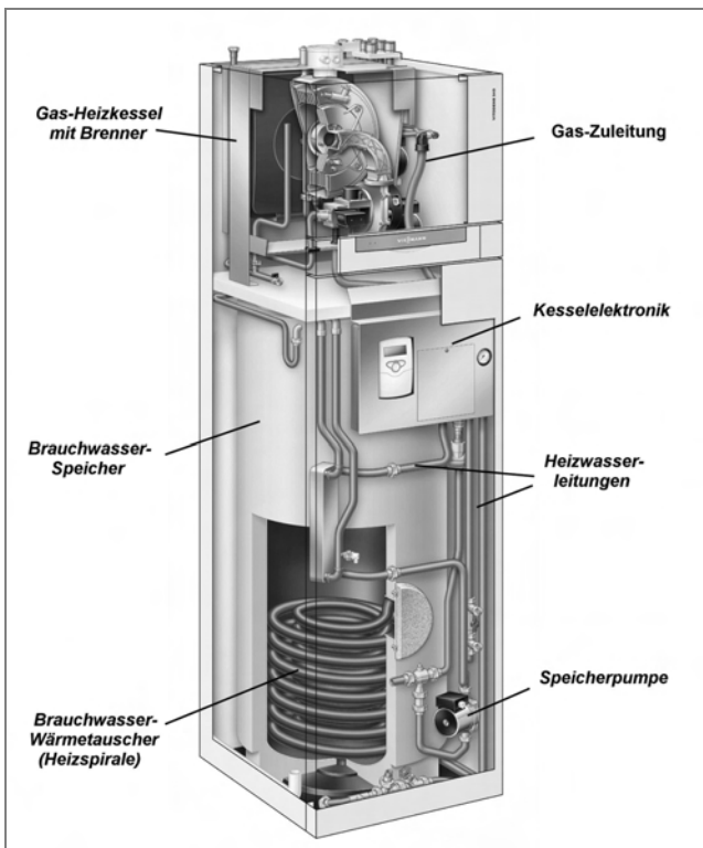
Abb. 10: Einsicht in das Innere des Heizkessels
