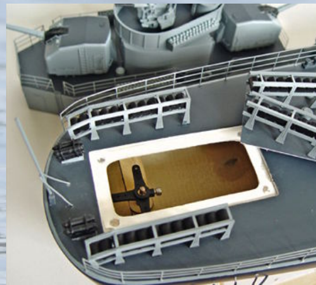
Die Anlenkung des Ruders verbirgt sich unter einem Deckel im Heck
