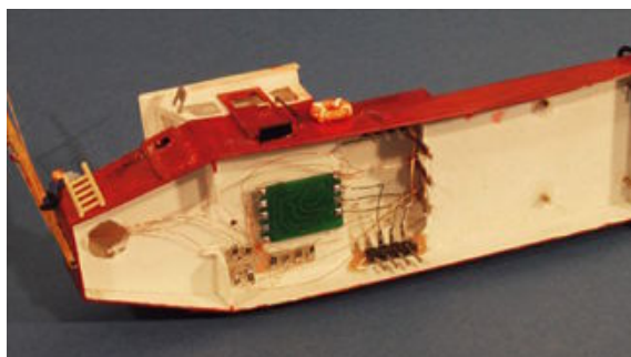
Der Aufbau wird elektrisch und mechanisch durch Stecker mit dem Rumpf verbunden. Ein kleiner 5-Kanal-Schalter und die Vorwiderstände der LEDs finden auch noch Platz
