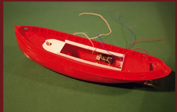
Mit 1-mm-Pastikplatten wird die Decksöffnung angepasst und das Süllbord aufgebaut
