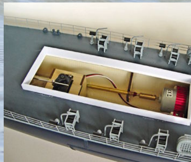
Motoren und Ruderservo befinden sich unter dem hinteren Aufbau
