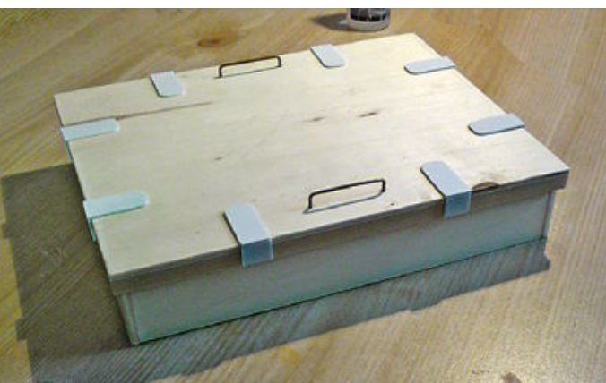
Die neue vordere Ladeluke
