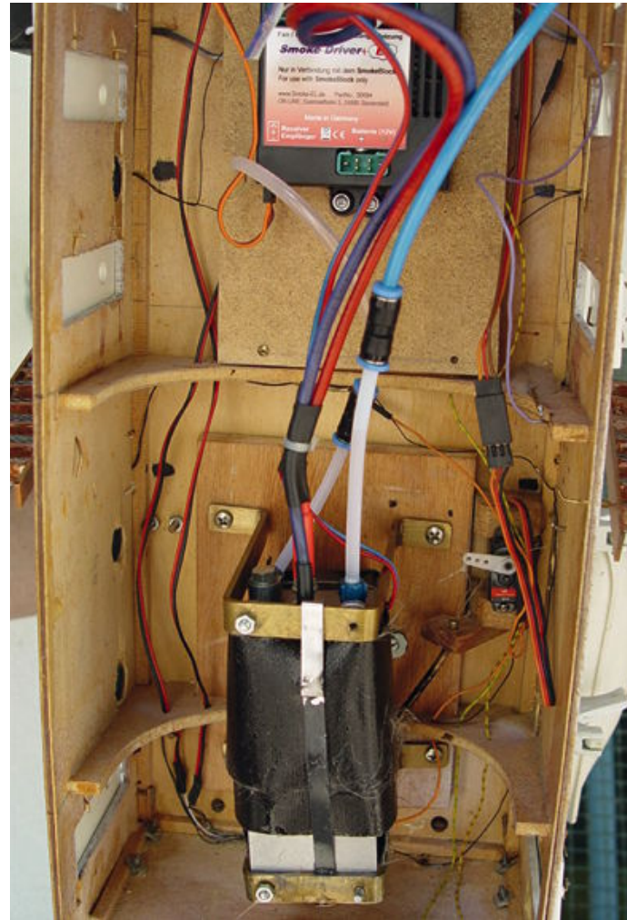
Steuerelektronik und Rauchgenerator sind am Dach des Aufbaus montiert
