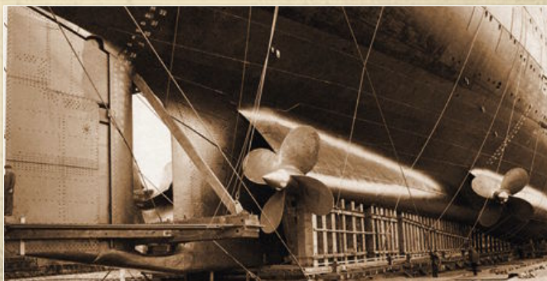
Ebenfalls eine Neuerung war die Ausführung des Ruders der Bremen
