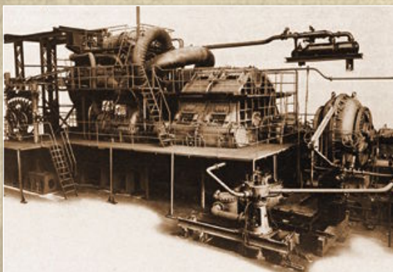
Ein Turbinensatz der Bremen auf dem Prüfstand
