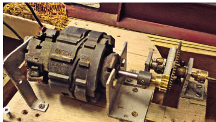
Musste weichen: der eingebaute Antrieb hatte seine besten Jahre schon hinter sich
