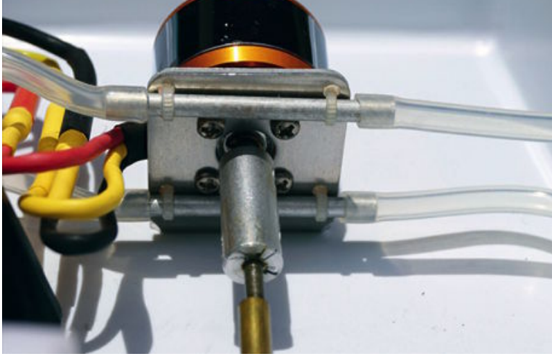
Der Außenläufer wird über den Motorspant gekühlt, eine Klemmkupplung nimmt die 3-mm-Flexwelle auf
