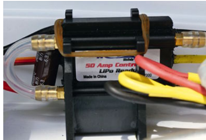
Der 50-A-Regler ist ebenfalls wassergekühlt
