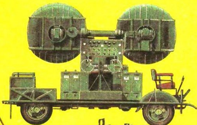
Fla- Geschützrichtstation B-2 (1939)
