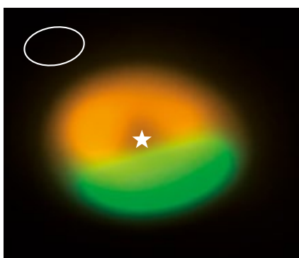
Der Stern Oph IRS 48 (weißer Asterisk) ist von einer asymmetrischen Staubscheibe umgeben: Die größeren Körnchen sammeln sich in einem Sektor (grün). Oben links ist zum Vergleich der Durchmesser der Neptunbahn gezeigt.
