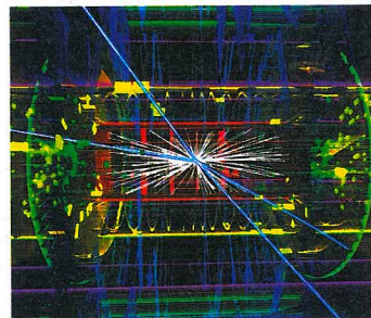
Small Bang: Das vom Computer erzeugte Bild basiert auf den Daten einer Teilchenkollision beim Cern
