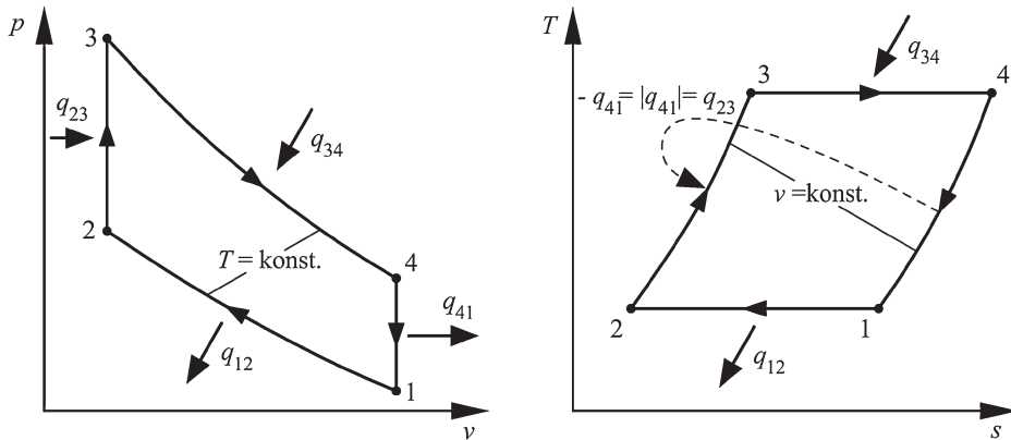
Abb. 7.7 Zustandsänderungen des Stirling-Prozesses
