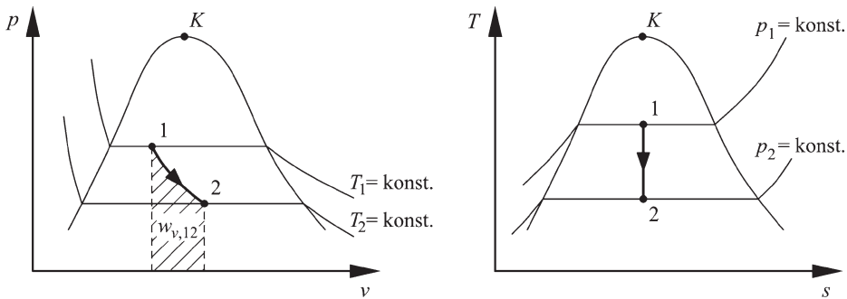
Abb. 5.12 Reversibel adiabate Zustandsänderungen im Nassdampfgebiet, dargestellt im p,v -Diagramm und im T,s -Diagramm
