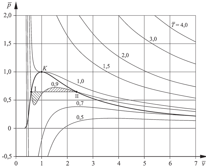
Abb. 4.6 Verlauf der Isothermen nach der van-der-Waals-Gleichung in einem \bar{p}, \bar{v} -Diagramm
