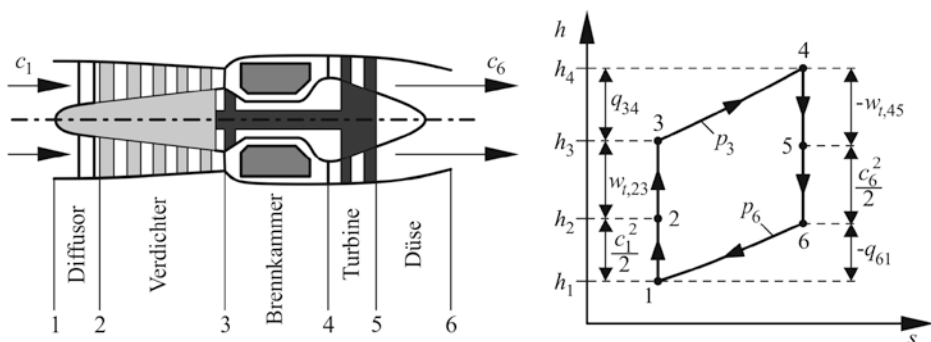
Abb. 7.9 Schematische Darstellung eines Gasturbinen-Strahltriebwerkes und des zugehörigen Vergleichsprozesses im h,s -Diagramm
