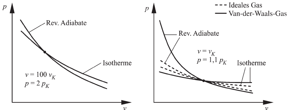
Abb. 5.8 Zustandsänderungen im p , v -Diagramm für ein reales und ideales Gasverhalten
