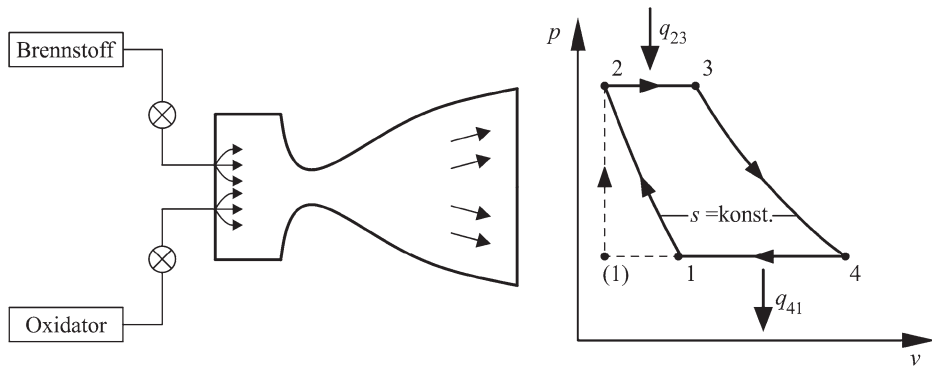
Abb. 7.10 Schematische Darstellung eines Raketentriebwerkes und Vergleichsprozess im p, v -Diagramm
