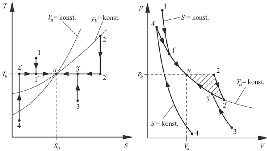
Abb. 6.2 Beispiele für reversible Zustandsänderungen geschlossener Systeme mit verschiedenen Anfangszuständen unter Energieaustausch mit der Umgebung. Der Systemendzustand ist immer der Umgebungszustand (Zustand u )
