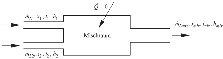
Abb. 7.31 Die Mischung von zwei feuchten Luftströmen
