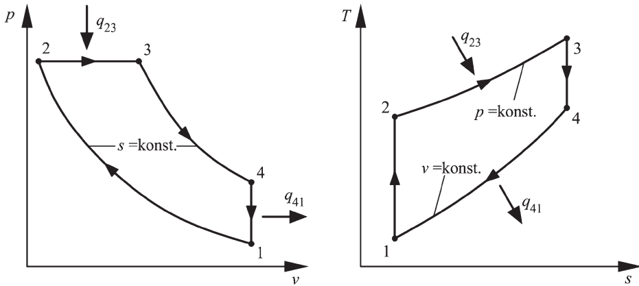
Abb. 7.6 Zustandsänderungen des Diesel-Prozesses
