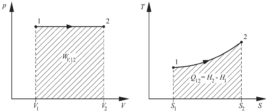
Abb. 5.2 Isobare Zustandsänderungen im p,V -Diagramm und im T,S -Diagramm
