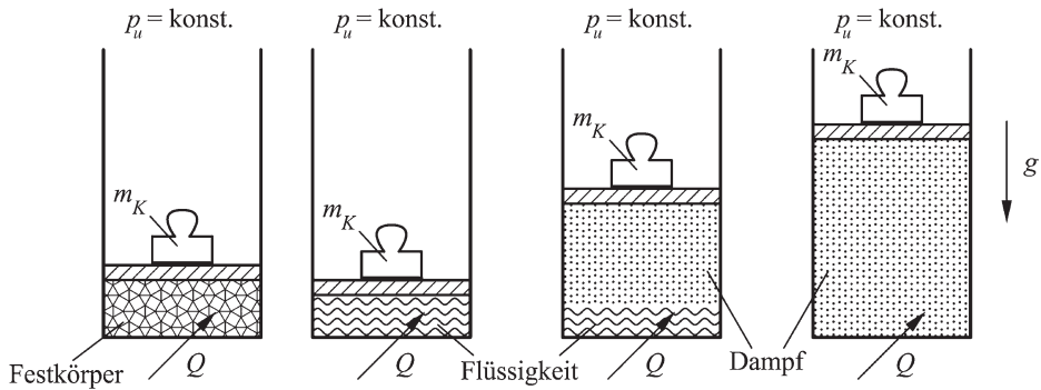
Abb. 4.1 Erhitzen eines Stoffes bei konstantem Druck
