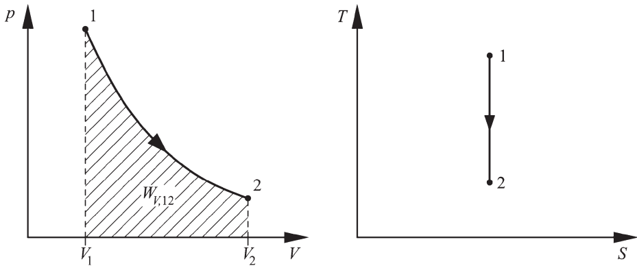
Abb. 5.5 Reversibel adiabate Zustandsänderung im p, V -Diagramm und im T, S -Diagramm
