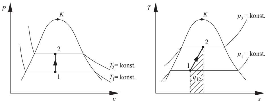
Abb. 5.11 Isochore Zustandsänderungen im Nassdampfgebiet, dargestellt im p,v -Diagramm und im T,s -Diagramm
