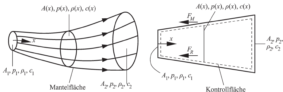
Abb. 7.22 Stromröhre bei stationärer Strömung und differenzielles Kontrollvolumen in einer Kanalströmung
