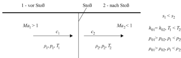
Abb. 7.26 Zustandsänderungen über den senkrechten Verdichtungsstoß
