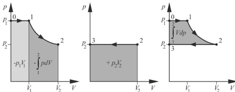
Abb. 3.5 Expansionsprozess einer kontinuierlich arbeitenden Kolbenmaschine
