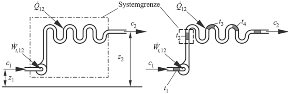
Abb. 3.4 Links: Darstellung einer Anlage als offenes, stationäres thermodynamisches System, das mit seiner Umgebung sowohl technische Arbeit als auch Wärme austauscht. Rechts: Betrachtung eines geschlossenen, instationären Systems einer konstanten Masse, die durch die Anlage strömt (Darstellung zu verschiedenen Zeiten t_1 bis t_4 )
