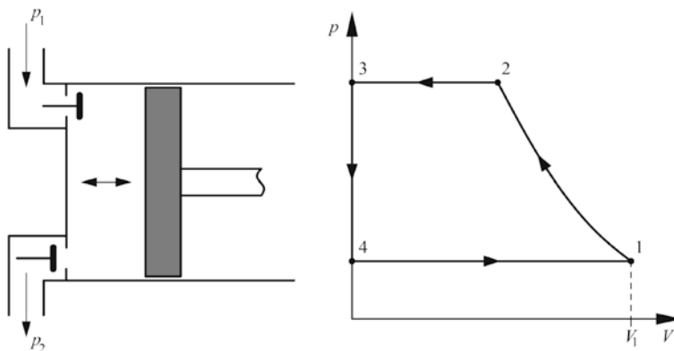
Abb. 7.1 Schematische Darstellung eines Kolbenverdichters und Darstellung der Arbeitsweise im p, V -Indikatordiagramm
