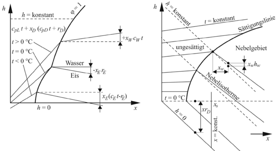
Abb. 7.29 Grundsätzlicher Aufbau eines geradwinkligen (links) und eines schiefwinkligen (rechts) h,x -Diagramms nach Mollier
