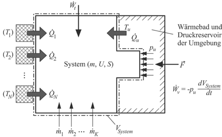
Abb. 6.1 Ein offenes, instationäres System, das mit mehreren Wärmebehältern und mit seiner Umgebung in Wechselwirkung steht
