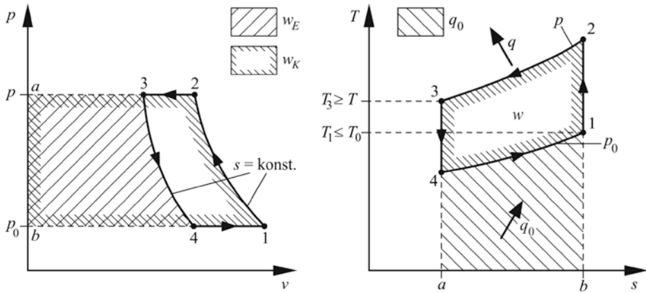
Abb. 7.16 Die Zustandsänderungen eines Kaltluftprozesses in einem p,v - und einem T,s -Diagramm
