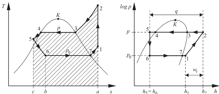
Abb. 7.20 Die Zustandsänderungen eines Wärmepumpe-Kaltdampfprozesses in einem T,s - und einem \log p,h -Diagramm
