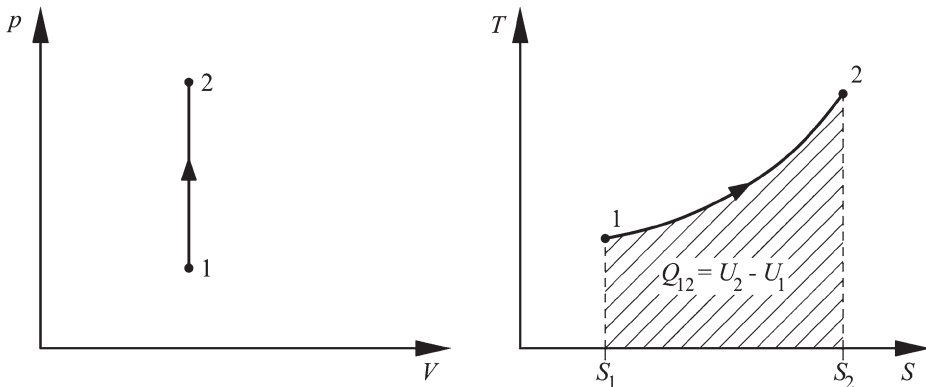
Abb. 5.3 Isochore Zustandsänderungen im p,V -Diagramm und im T,S -Diagramm
