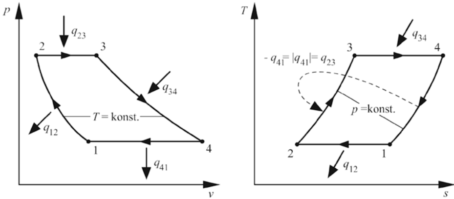
Abb. 7.11 Zustandsänderungen des Ericsson-Prozesses
