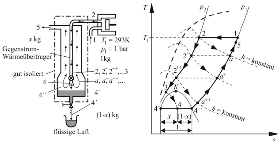
Abb. 7.21 Prinzipische Skizze und Prozessführung im T,s-Diagramm der Luftverflüssigung nach Linde
