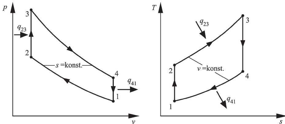
Abb. 7.5 Zustandsänderungen des Otto-Prozesses
