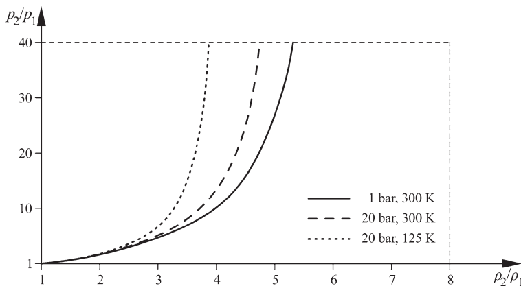
Abb. 7.27 Hugoniotkurve für ein van-der-Waals-Gas bei verschiedenen Zustandsbedingungen ( p_1, T_1 )
