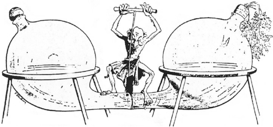
Abb. 3.7 Der Maxwellsche Dämon bei der Arbeit (nach einer Abbildung von Darling und Hultburt aus dem Jahr 1955)
