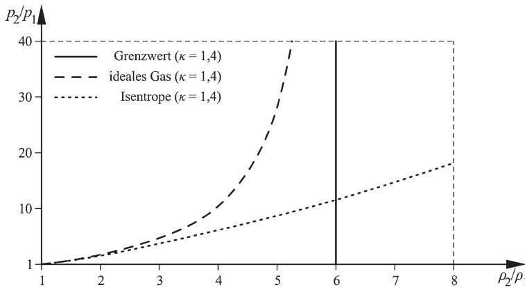
Abb. 7.28 Hugoniotkurve und Isentrope für ein zweiatomiges ideales Gas
