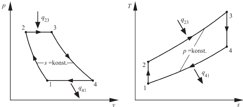
Abb. 7.8 Zustandsänderungen des Joule-Prozesses
