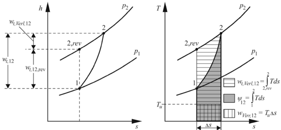
Abb. 7.3 Veranschaulichung zur Definition des isentropen Verdichterwirkungsgrades
