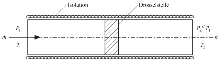
Abb. 5.7 Adiabate Drosselung eines kontinuierlich fließenden Gasstroms in einem Rohr
