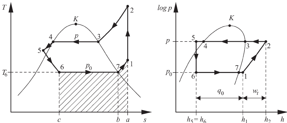
Abb. 7.18 Die Zustandsänderungen eines Kaltdampfprozesses in einem T,s - und einem \log p, h -Diagramm
