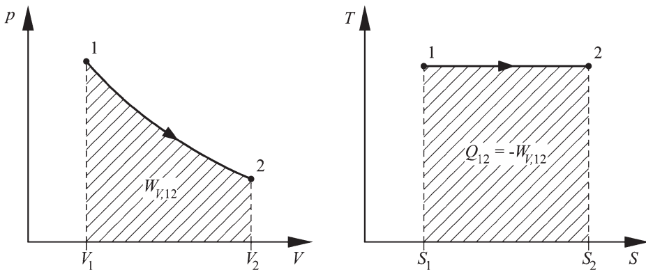
Abb. 5.4 Isotherme Zustandsänderungen im p, V -Diagramm und im T, S -Diagramm
