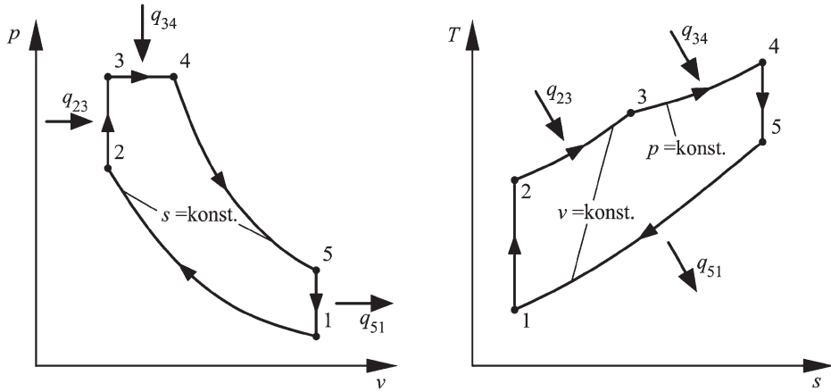
Abb. 7.4 Zustandsänderungen des Seiliger-Prozesses
