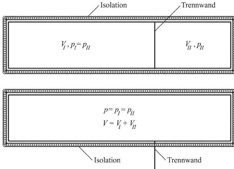
Abb. 5.6 Irreversible Vermischung zweier Gase
