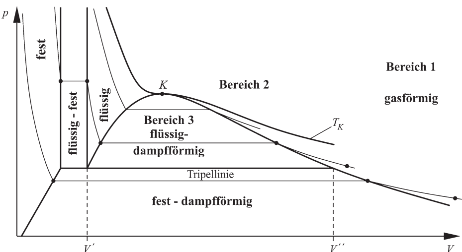
Abb. 4.3 Schematisches p,V -Diagramm für Kohlendioxid
