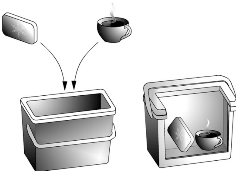
Abb. 3.2 Ein ursprünglich kalter Kühlakku und eine ursprünglich heiße Tasse Kaffee befinden sich im thermischen Kontakt und nehmen als Teilsysteme eines abgeschlossenen Gesamtsystems nach ausreichend langer Zeit die gleiche Temperatur an
