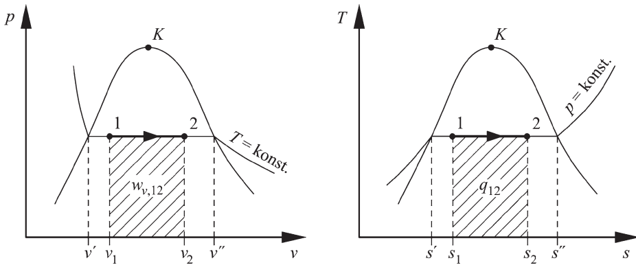
Abb. 5.10 Isobare Zustandsänderungen im Nassdampfgebiet dargestellt im p,v -Diagramm und im T,s -Diagramm
