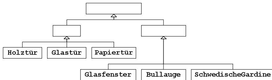
Abbildung 9.7: Übungsaufgabe: Generalisierung (2)
