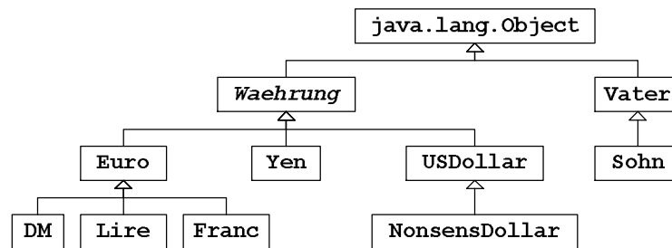
Abbildung 11.3: Klassenstammbaum
