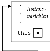
Abbildung 10.4: Die this-Referenz
