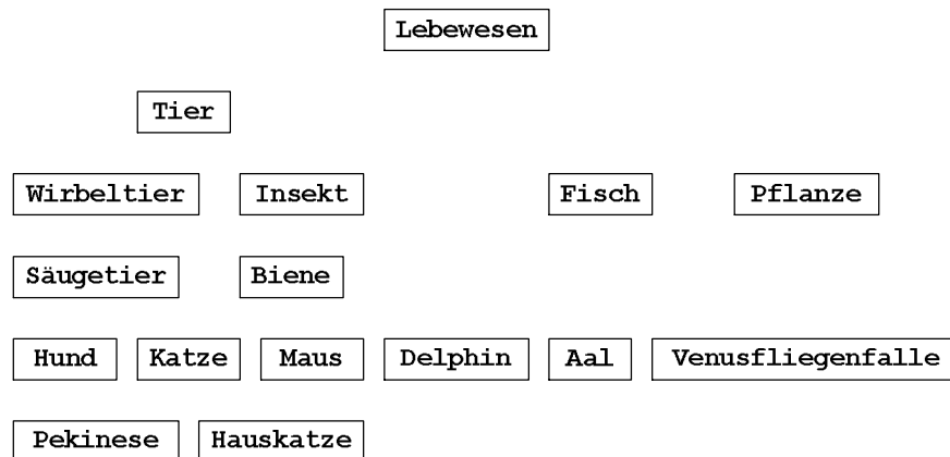
Abbildung 9.6: Übungsaufgabe: Generalisierung (1)
