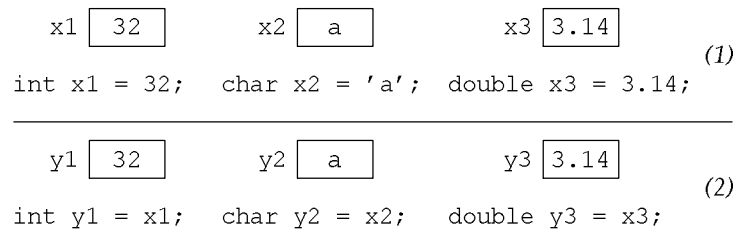
Abbildung 6.8: Einfache Datentypen
