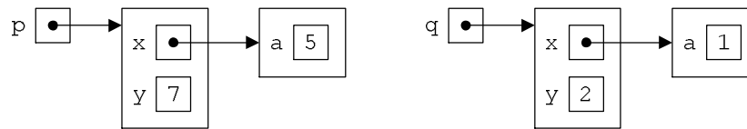
Abbildung 10.9: Ausgangsbild Aufgabe 10.15
