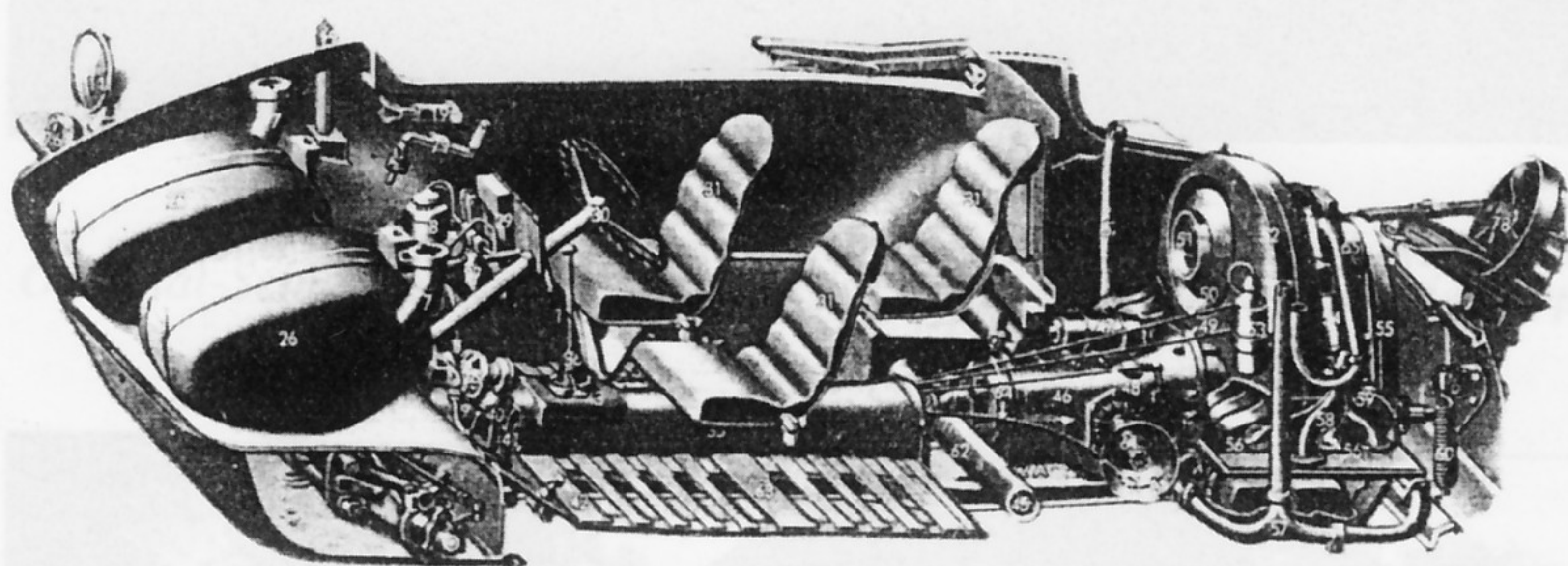
Schnitt durch den VW-Schwimmkübel Typ 166.
