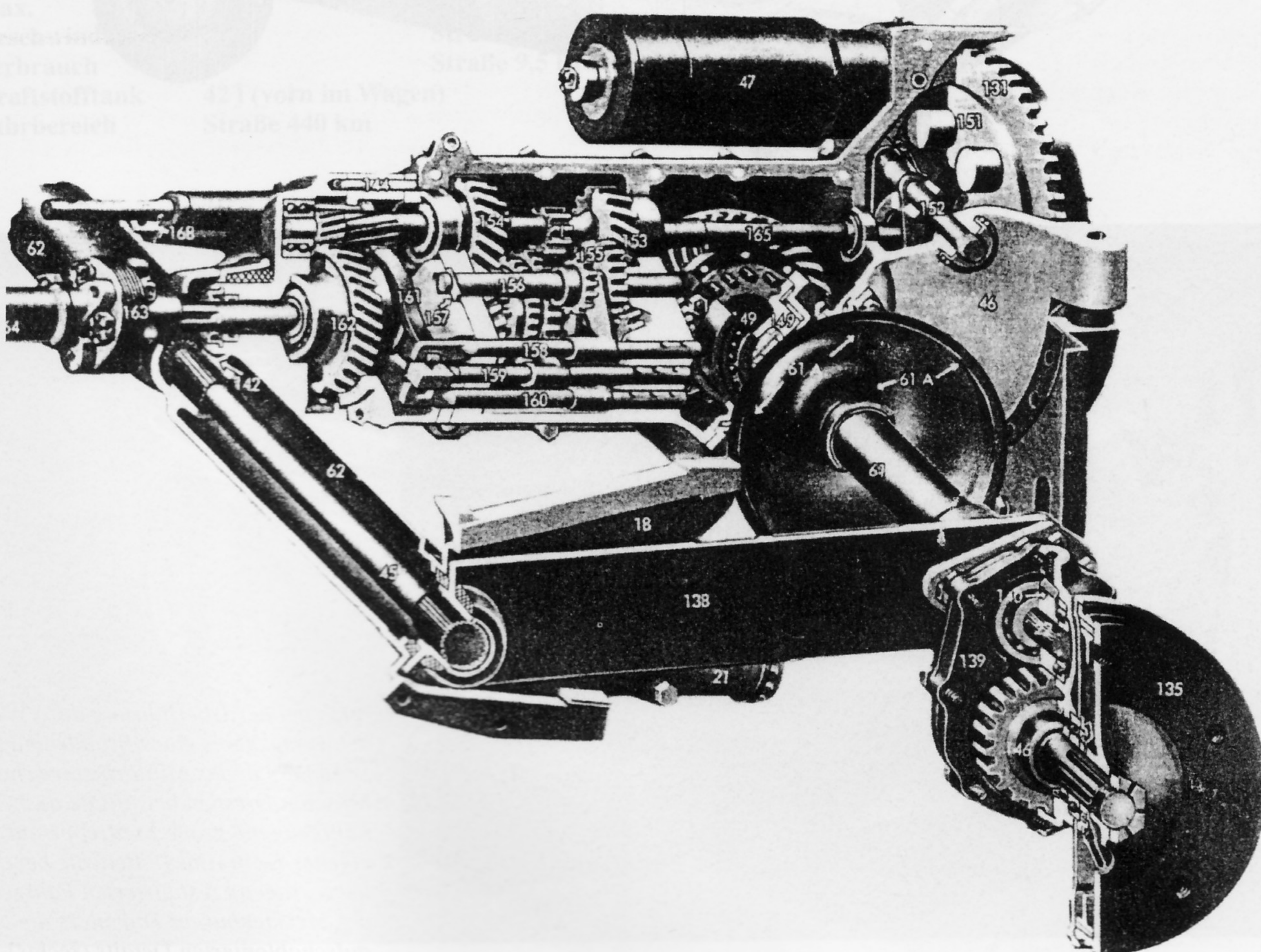
Schnittbild der Vorderachse (oben) sowie des Wechselgetriebes und der Hinterachse (unten). Der Radstand betrug 1220/1230 mm.
