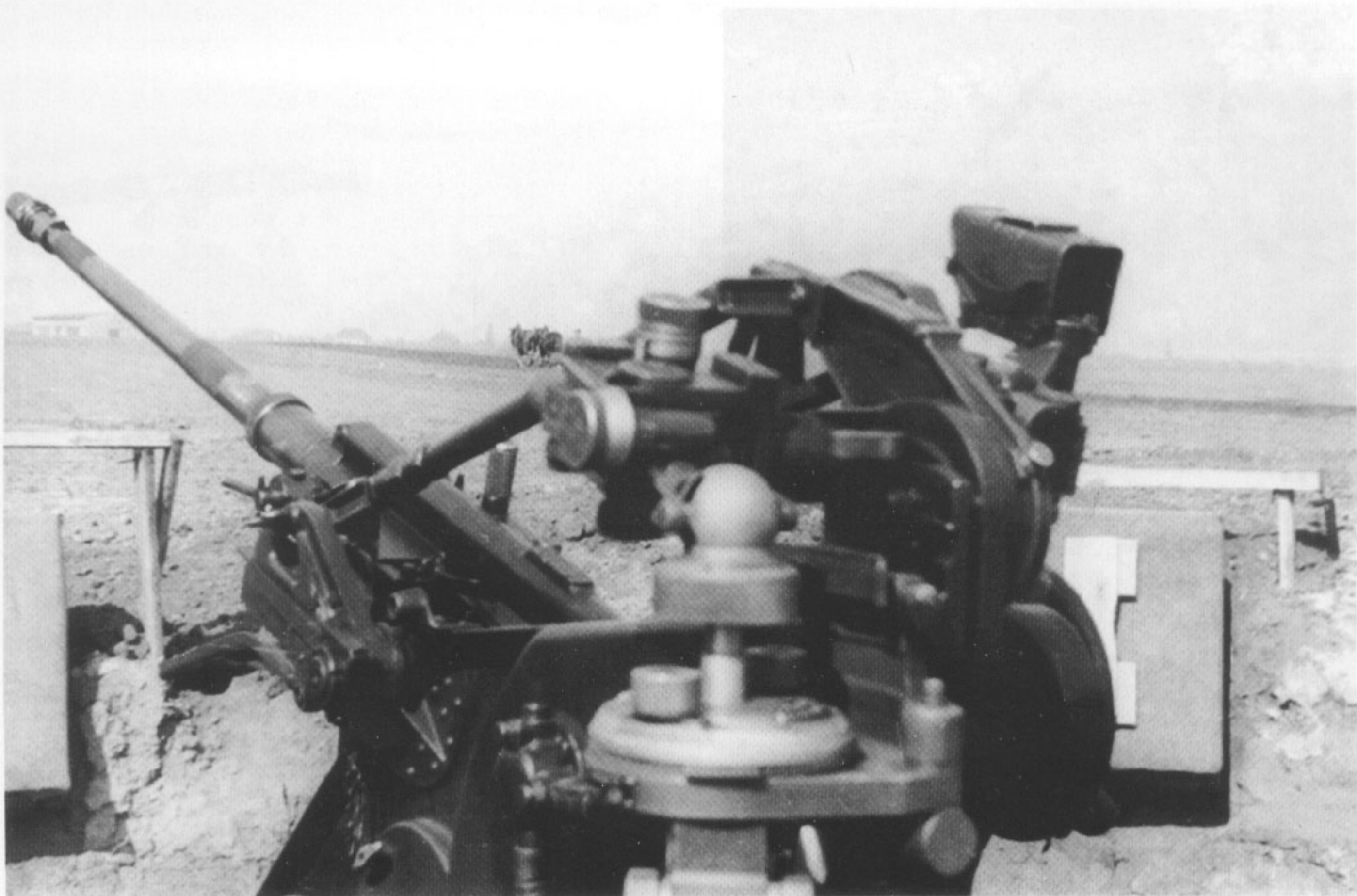
Detailaufnahme des Flakvisier 35. Es handelt sich dabei um ein Spiegelreflexvisier mit automatischer Rechendose. Außerdem stand ein mechanisches Visier, das Liniealvisier zur Verfügung. Erdziele wurden mit dem Erdzielfernrohr 3x8° anvisiert.
