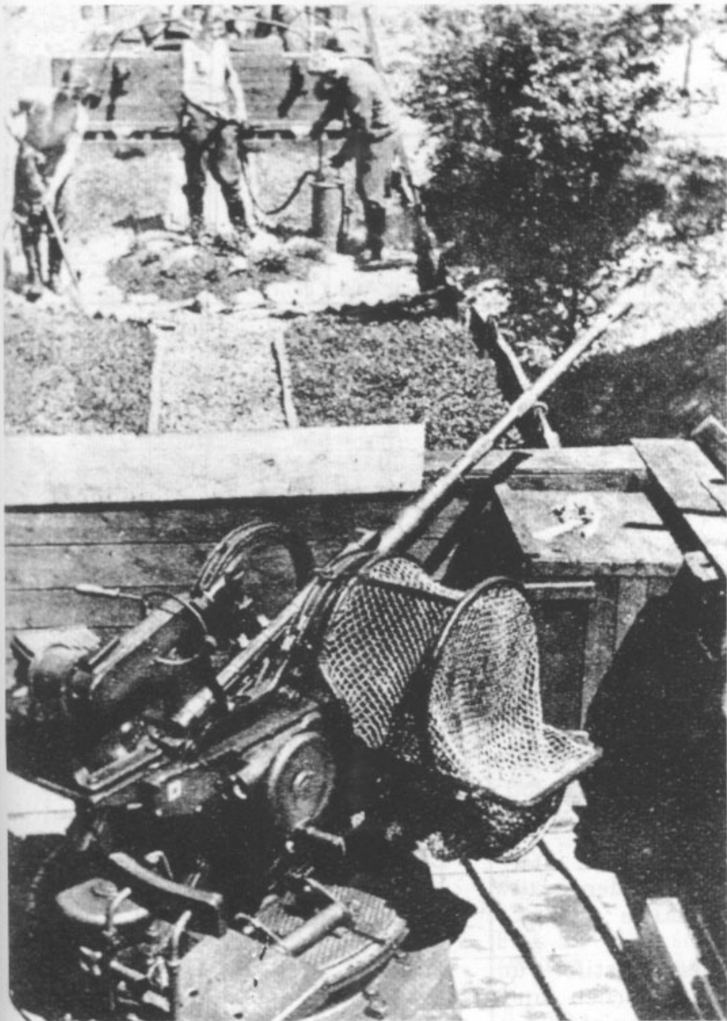
Eine 2-cm-Fliegerabwehrkanone 38 auf einem behelfsmäßig hergestellten Eisenbahn-Flak-Schutzwagen.
