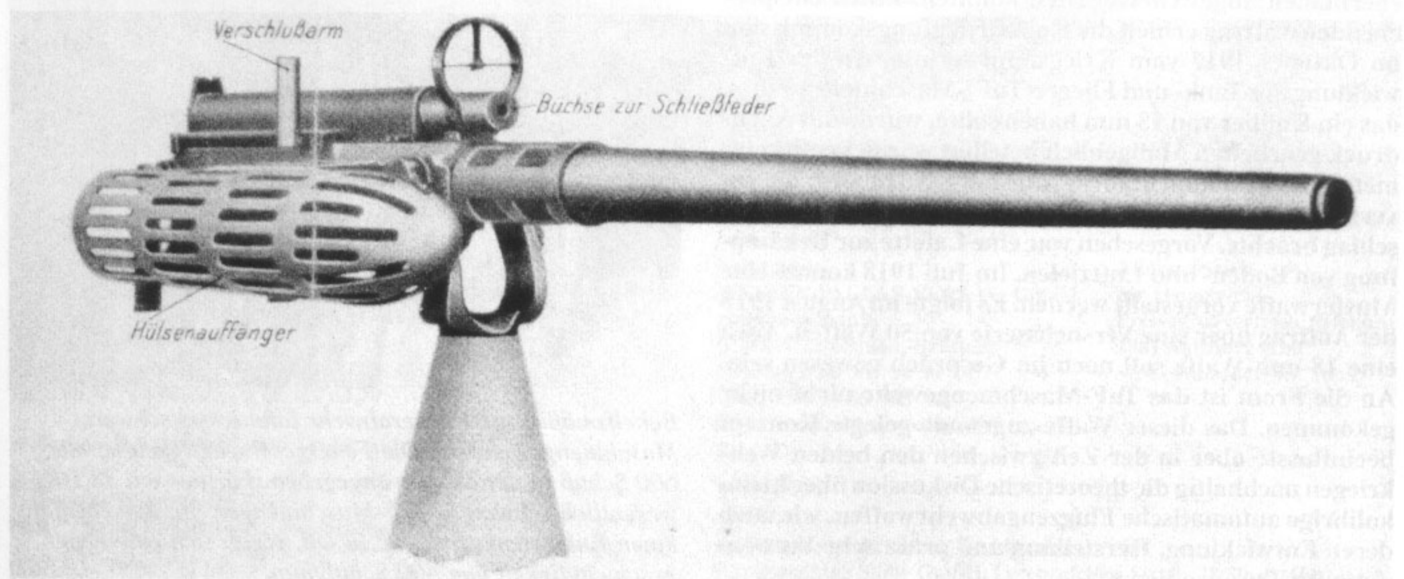
Die 2-cm-Kanone (Ehrhardt). Eine vorläufige Vorschrift für diese Waffe erschien im Februar 1918. Der Rückstoßlader besaß einen Verschluß mit starrer Verriegelung und wog 35 Kg. In der Sekunde konnten drei Schuß abgegeben werden. Die leeren Hülsen wurden in dem rechts angebrachten Hülsenfänger gesammelt.
