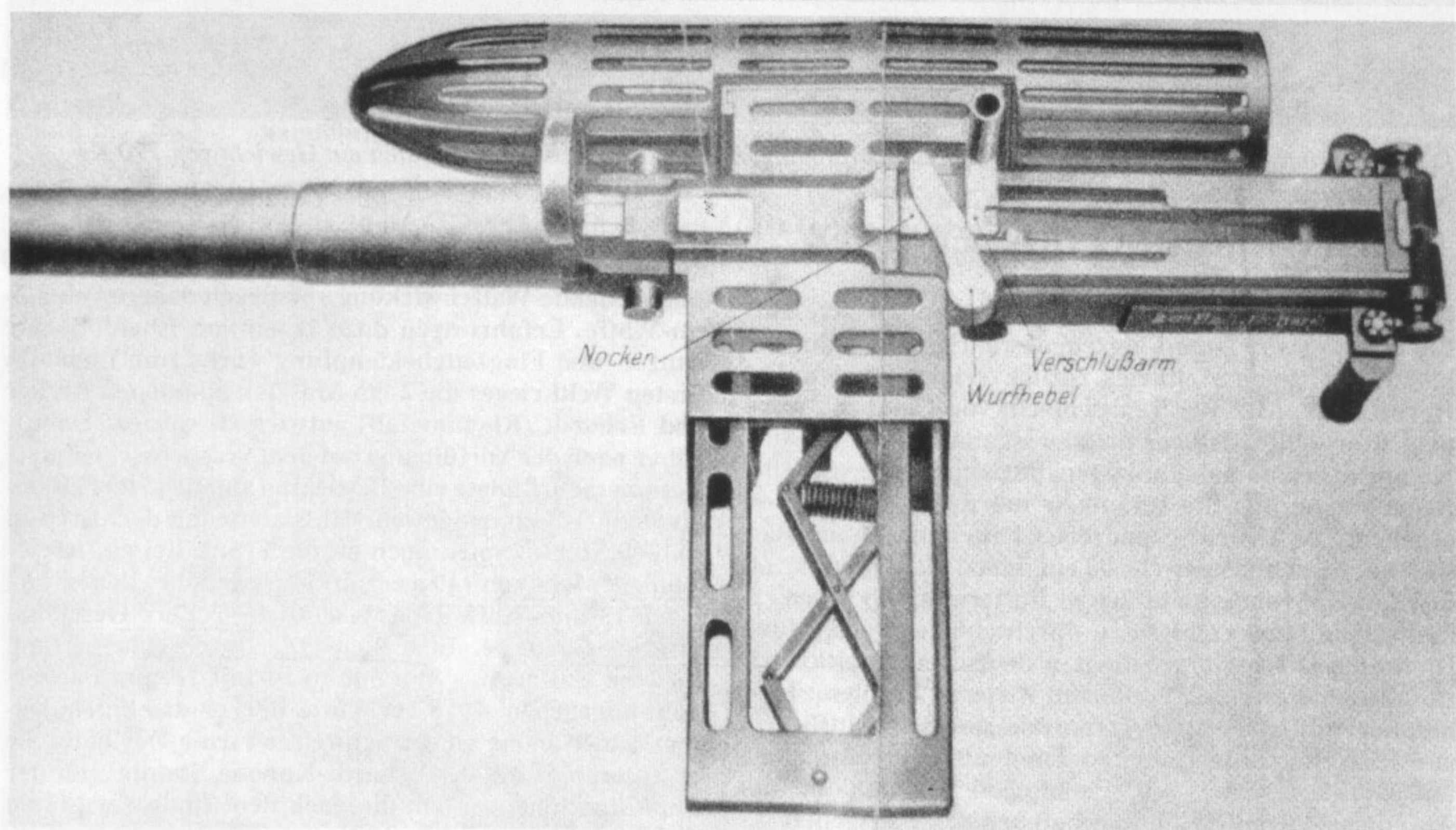
Die 2-cm-Kanone (Ehrhardt). Eine vorläufige Vorschrift für diese Waffe erschien im Februar 1918. Der Rückstoßlader besaß einen Verschluß mit starrer Verriegelung und wog 35 Kg. In der Sekunde konnten drei Schuß abgegeben werden. Die leeren Hülsen wurden in dem rechts angebrachten Hülsenfänger gesammelt.
