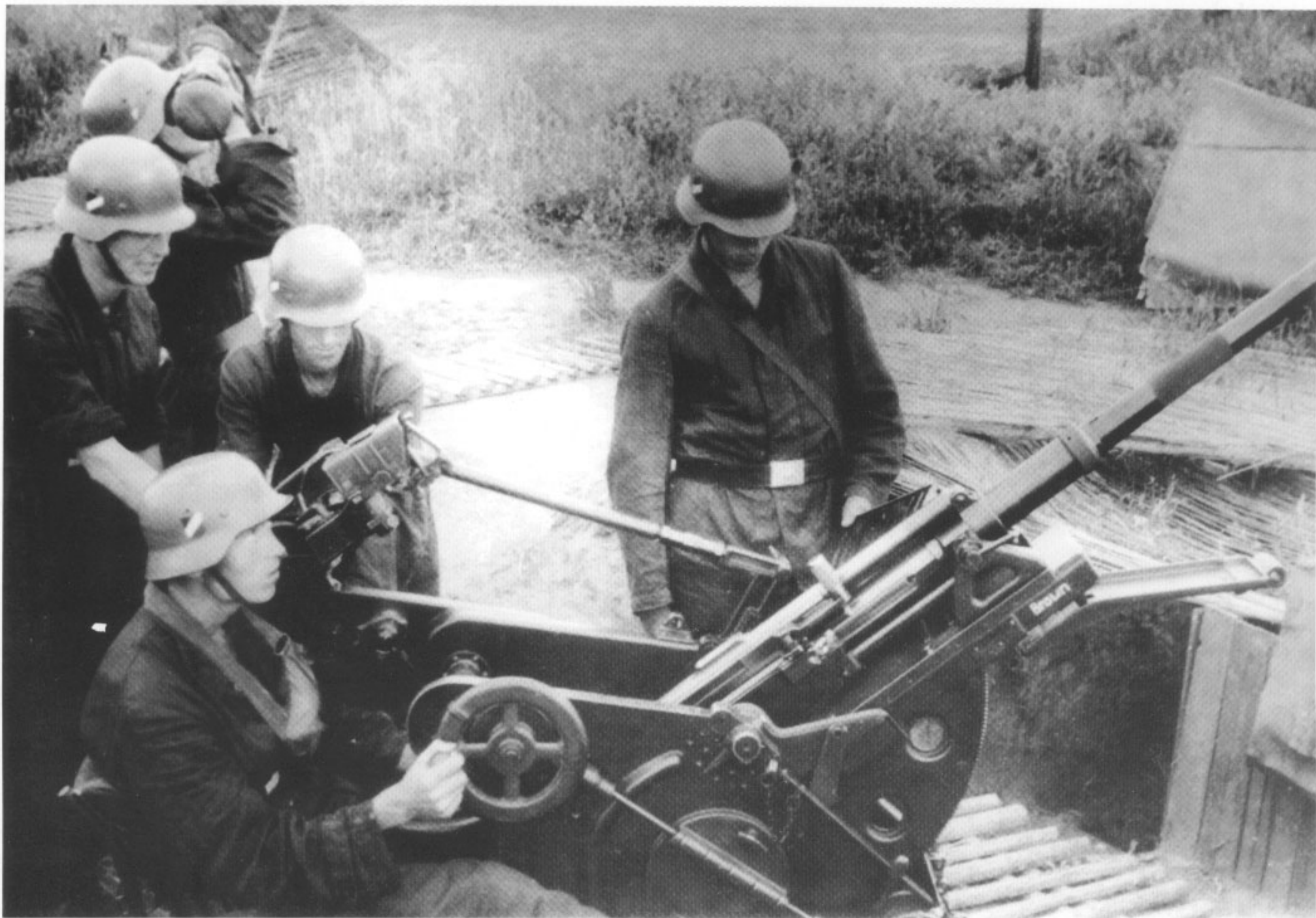
Zum Schutz der Flakstellungen im Heimatskriegsgebiet wurden während des Krieges die leichte Flaktrupps mit 2-cm-Fliegerabwehrkanonen 30 (im Bild) und 38 abgestellt. Mit ihrer Hilfe sollten die schweren Fliegerabwehrkanonen (8,8 cm, 10,5 cm und 12,8 cm) vor den Angriffen von Tieffliegern gesichert werden.
