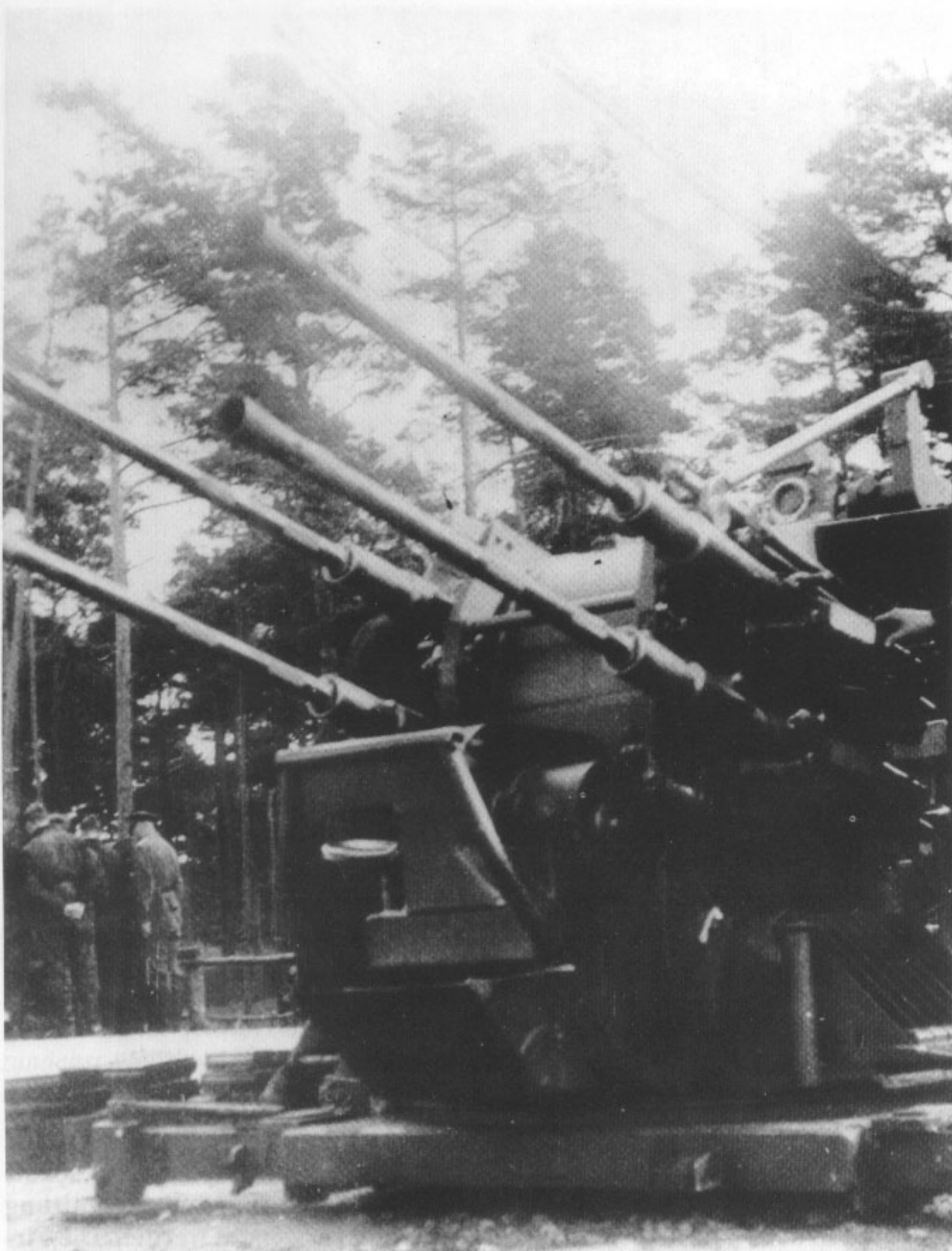
Die 2-cm-Vierlings-Fliegerabwehrkanone 38 auf Dreiecksbettung ließ sich auf dem Sonderanhänger 52 fahren. Außerdem trat sie auf dem mittleren Zugkraftwagen 8 t (Sd.Kfz. 7/1) und im Flak-Panzer IV "Wirbelwind" in Erscheinung. Häufig war der Vierling auch auf den Geschütz- bzw. Flak-Schutzwagen der Deutschen Reichsbahn anzutreffen.
