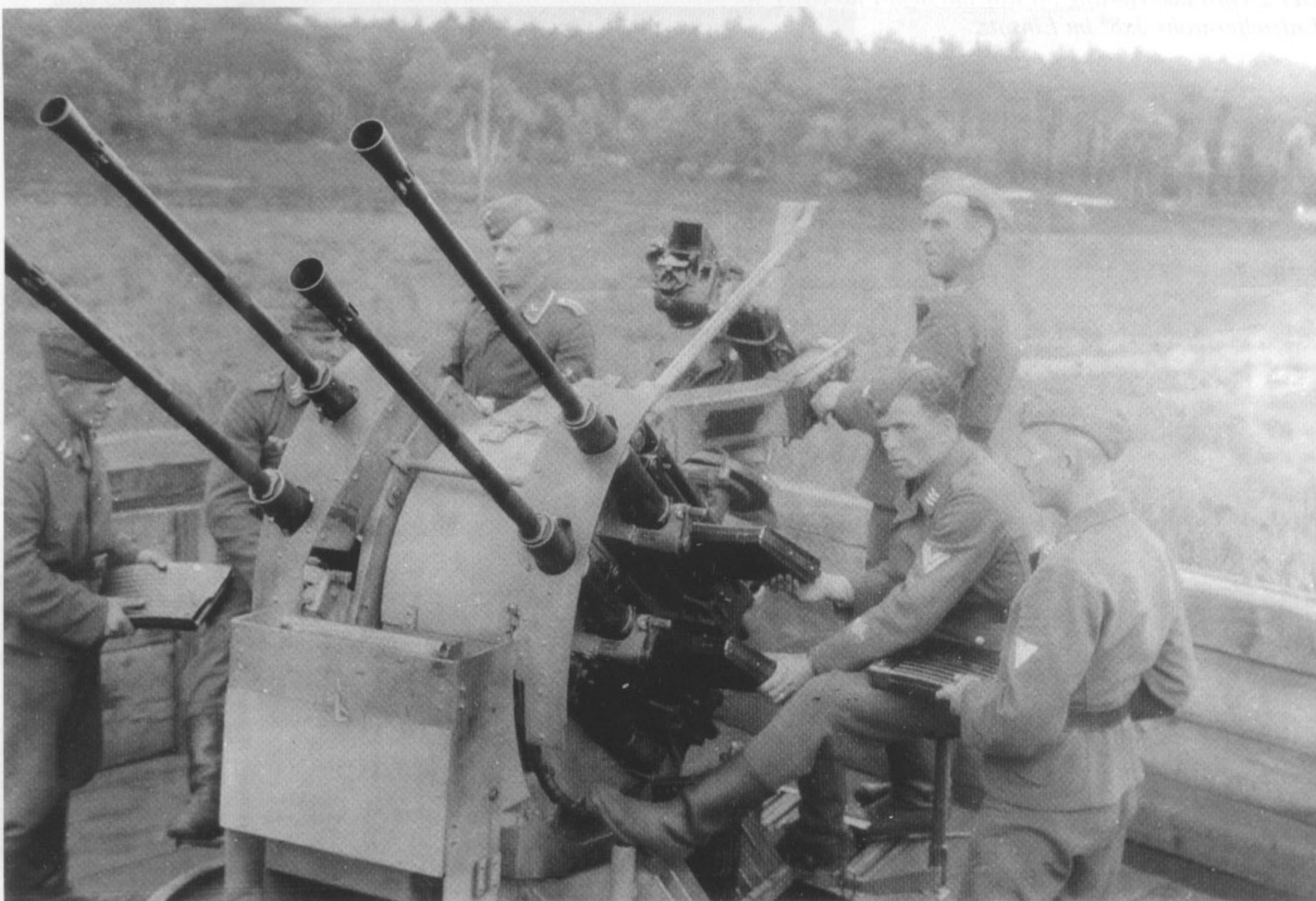
Die Munition für den 2-cm-Flak-Vierling wurde in 20-Schuß-Ansteckmagazinen zugeführt. Ihr Gewicht ist, mit 20 Granatpatronen gefüllt, mit 9,5 Kg angegeben. Eine 2-cm-Sprenggranatpatrone L'Spur wog etwa 0,3 Kg, eine 2-cm-Panzergranatpatrone 0,33 Kg.
