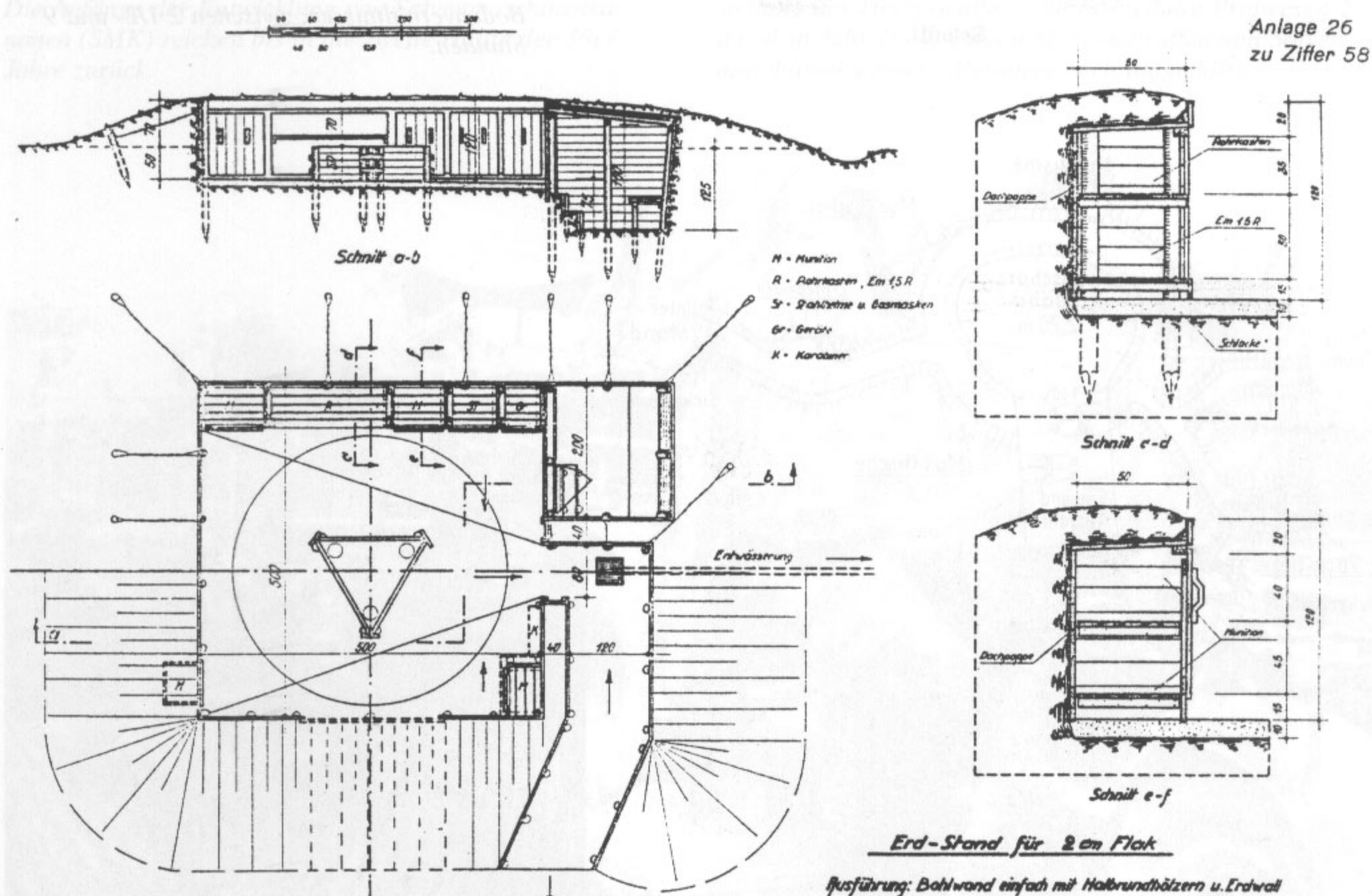
Der Erdstand für 2-cm-Fliegerabwehrkanonen 30 und 38 mit einer einfachen Bohlenwand aus Halbrundhölzern und Erdwall. Die Feuerstellung ist mit einer 2-cm-Fliegerabwehrkanone 38 besetzt.
