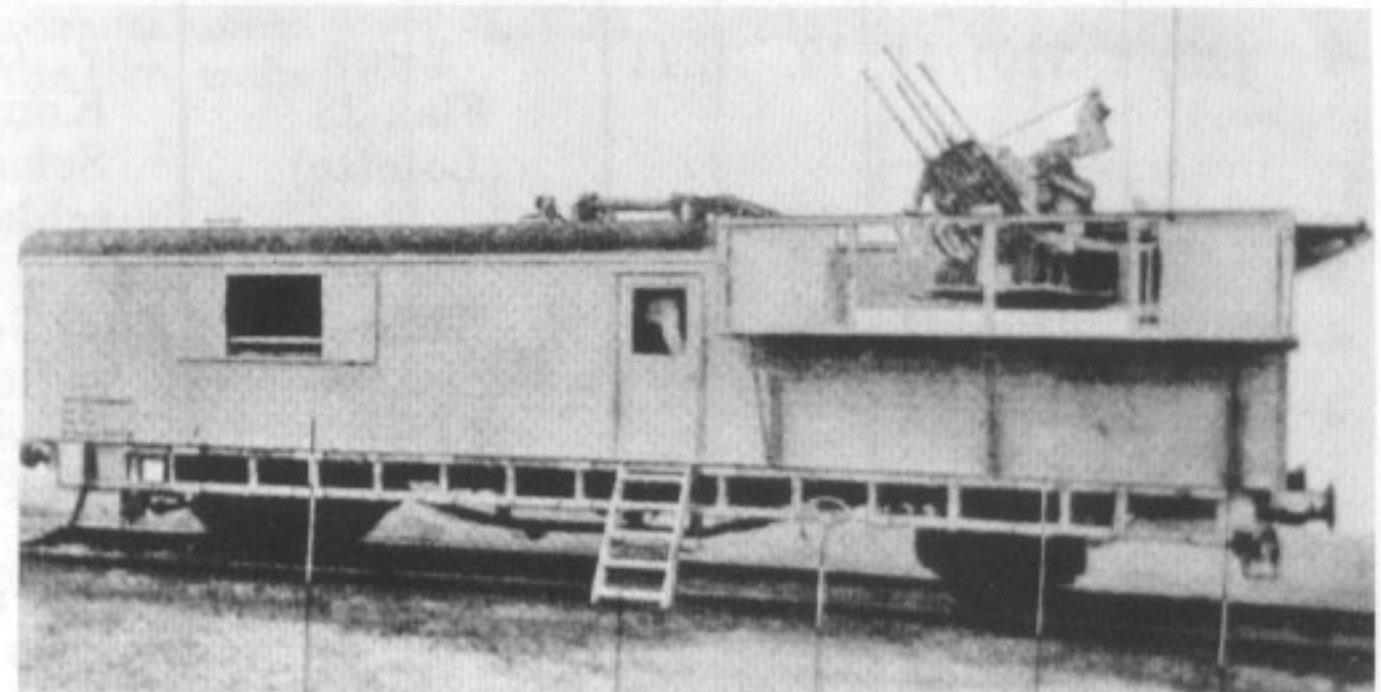
Der Geschützwagen II (E) leichte Flak mit dem 2-cm-Falk-Vierling in Feuerstellung.
