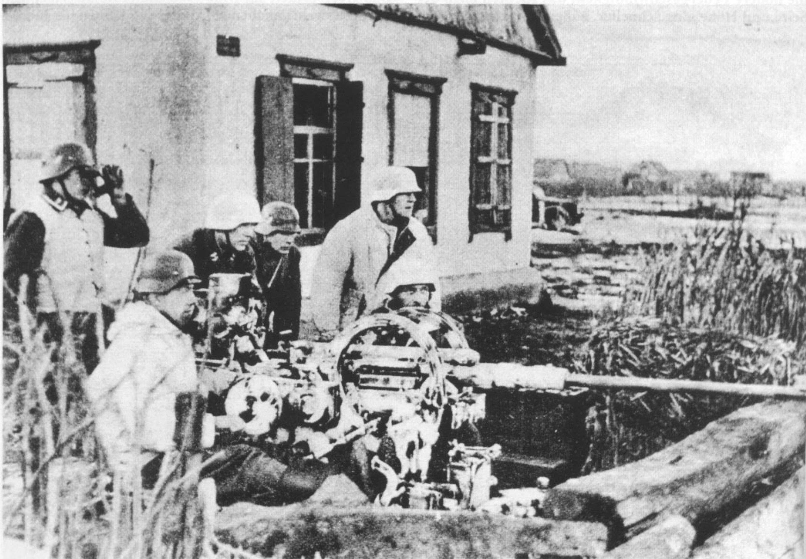
Feuerbereit zum Erdzielbeschuß - eine 2-cm-Fliegerabwehrkanone während der Abwehrkämpfe an der Ostfront im Winter 1942/43. Der Bedienung dieses Geschützes war es gelungen, einen russischen T-34 außer Gefecht zu setzen, nachdem sie dessen Zusatztanks zerschossen hatte.
