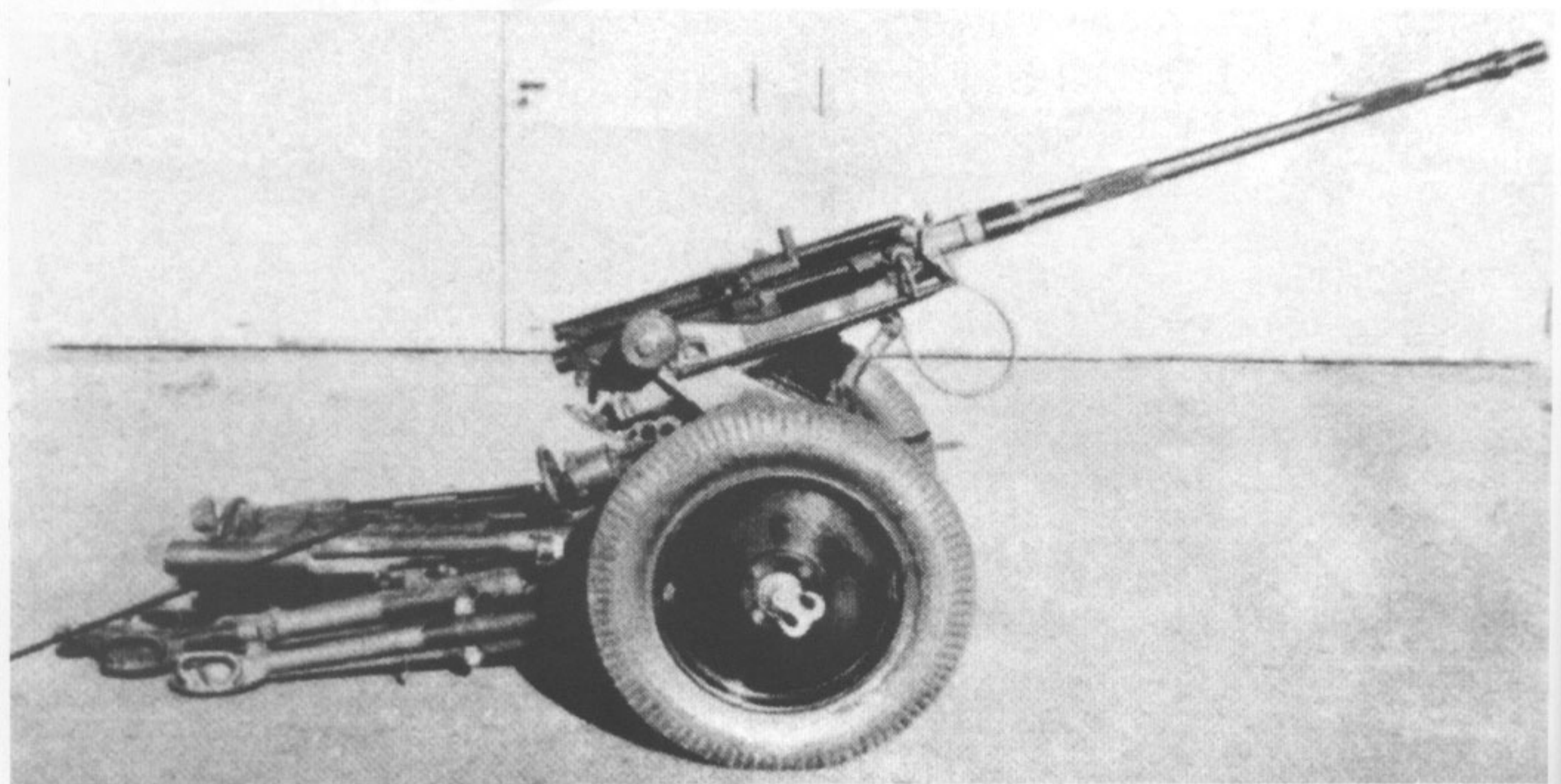
Eine lufttransportfähige 2-cm-Fliegerabwehrkanone 30 in Fahrstellung.
