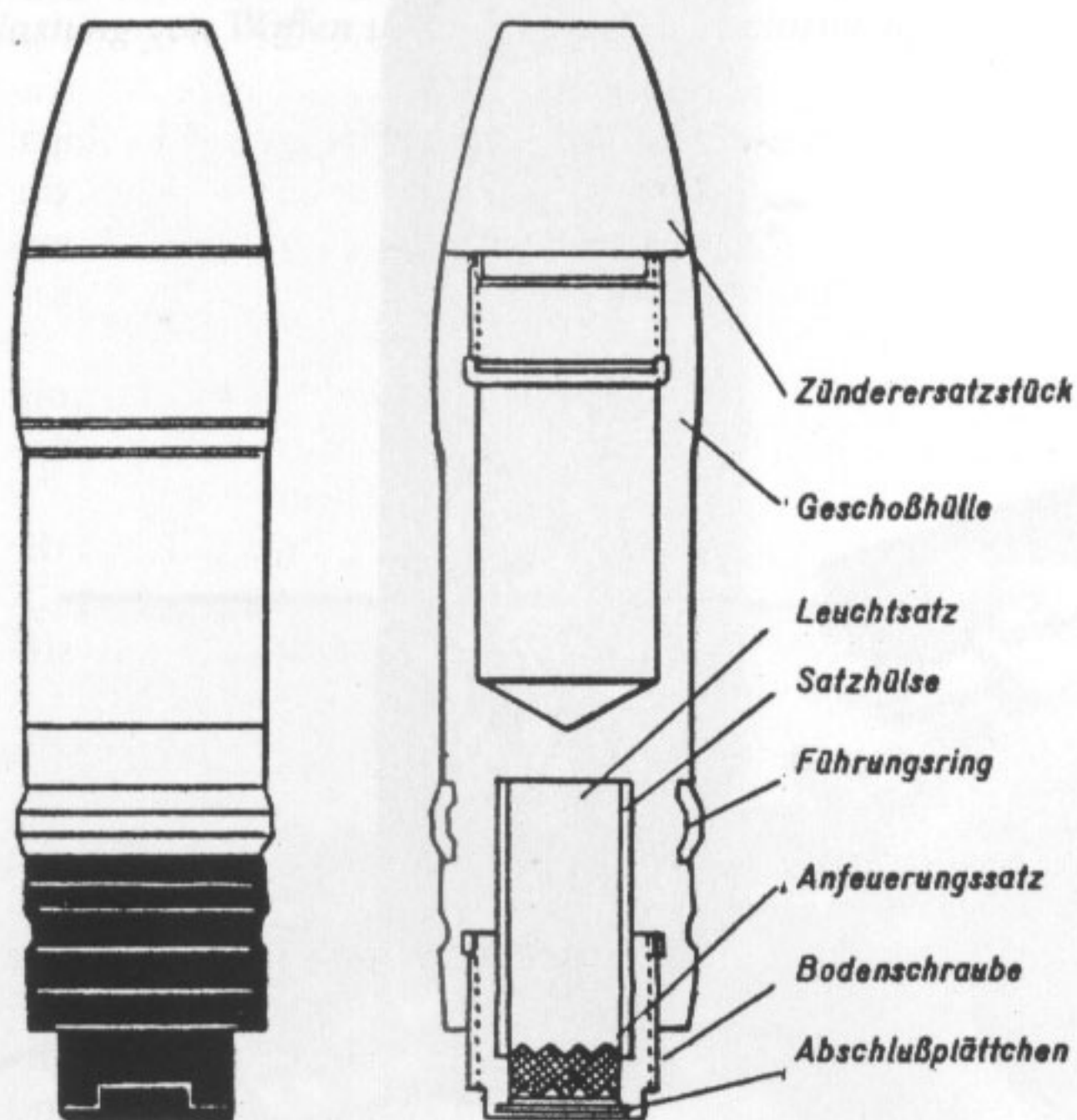
2-cm-Sprenggranate L'spur (Üb)
