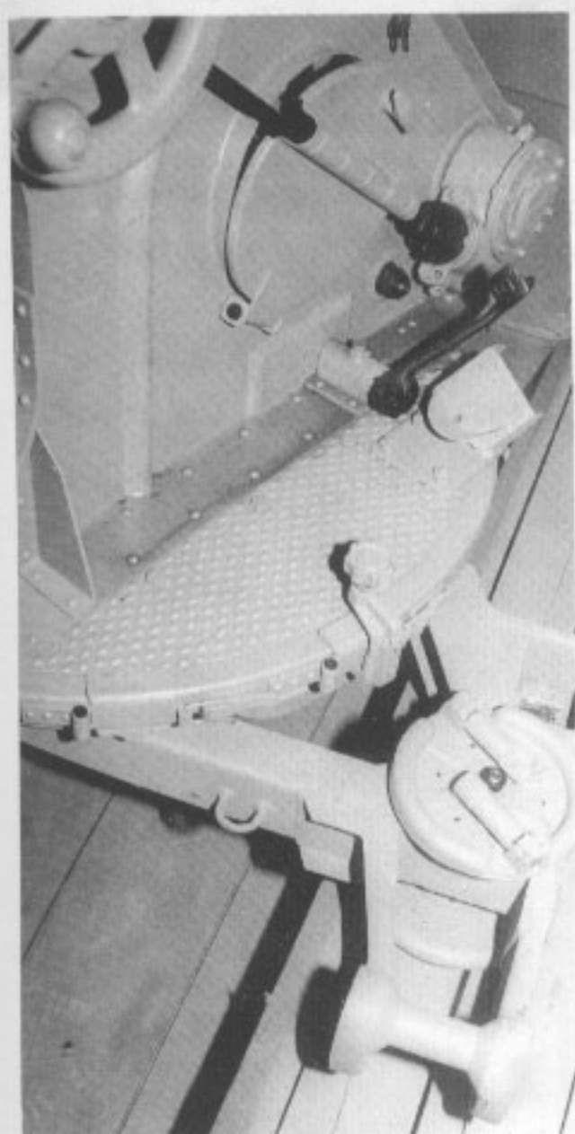
Detailbilder des Visiertragearms und des Richtmechanismus. Der Höhenrichtbereich ist mit -10 Grad bis +90 Grad angegeben, die Seitenrichtung mit 360 Grad. Die komplette Oberlafette wog 196 Kg.
