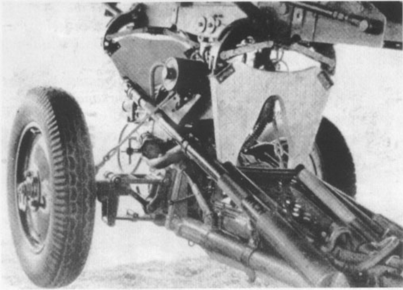
Um die 2-cm-Fliegerabwehrkanonen 30 für den Lufttransport verlasten zu können, wurden insgesamt 14 zusätzliche Teile benötigt, darunter eine 0,7 m lange Notwurfleine mit einer Bruchlast zwischen 15- und 50 Kg. Das Bild zeigt die Aufhängung des Geschützes mit eingesetzten Holzbrettern.
