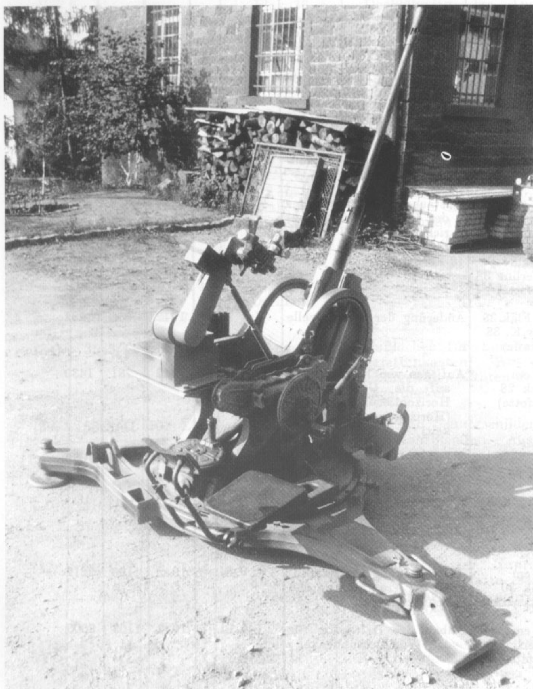
Die 2-cm-Fliegerabwehrkanone 38 in Feuerstellung.
