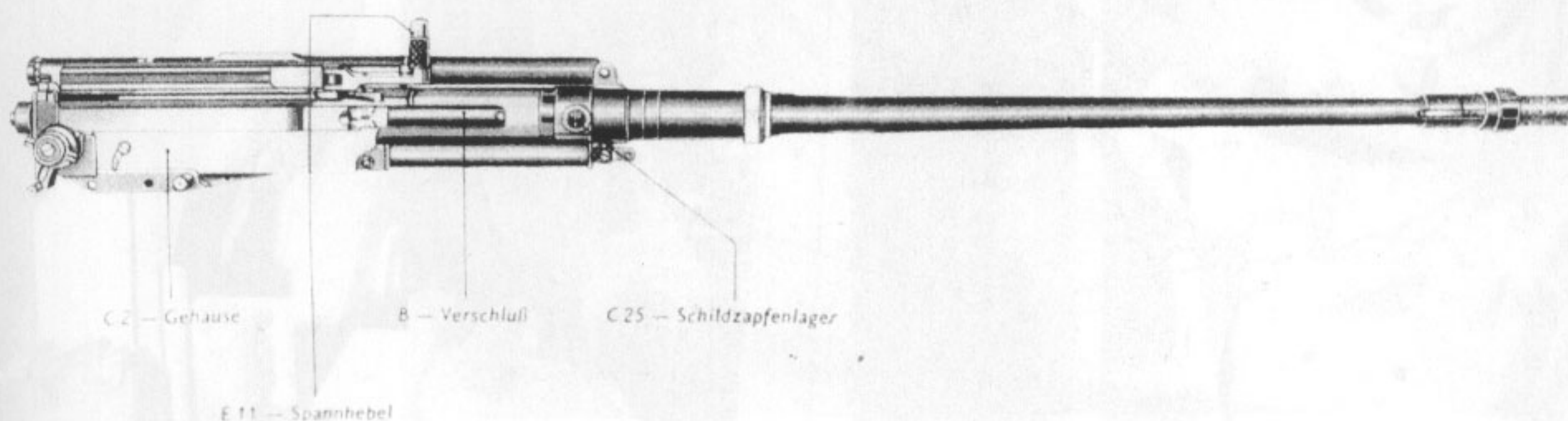
Bild 5 Gesamtansicht der Waffe von rechts (Hülseauswurfseite)
