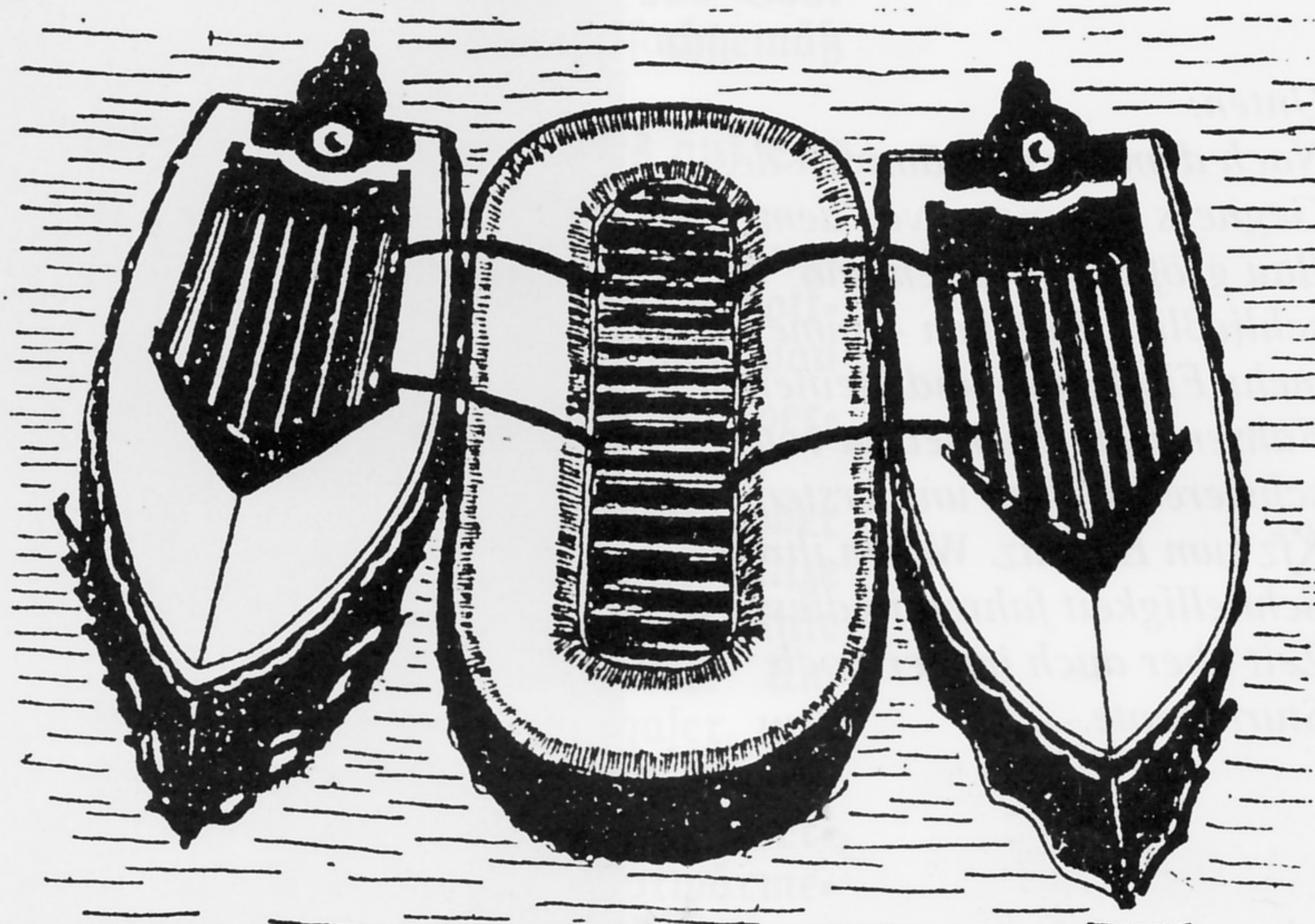
Beim Fahren ist es zweckmäßig, den besten Pi.-Steuermann auf das Steuerbord-Pi.-Sturmboot einzusetzen.
