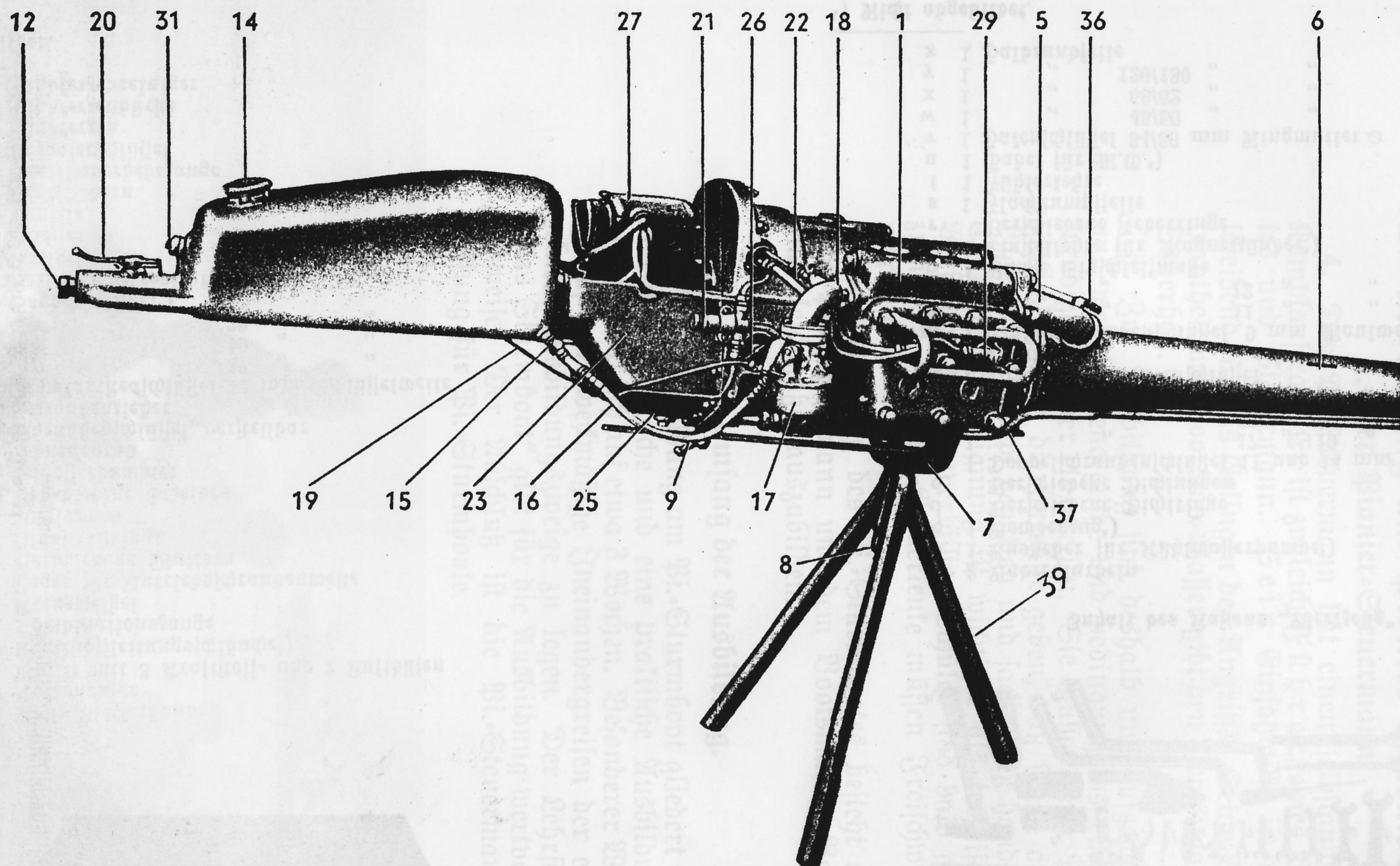
Motorblock von der Seite des Öldruckmessers aus gesehen, mit abgenommenem Schutzdeckel zum Magnetzündler
