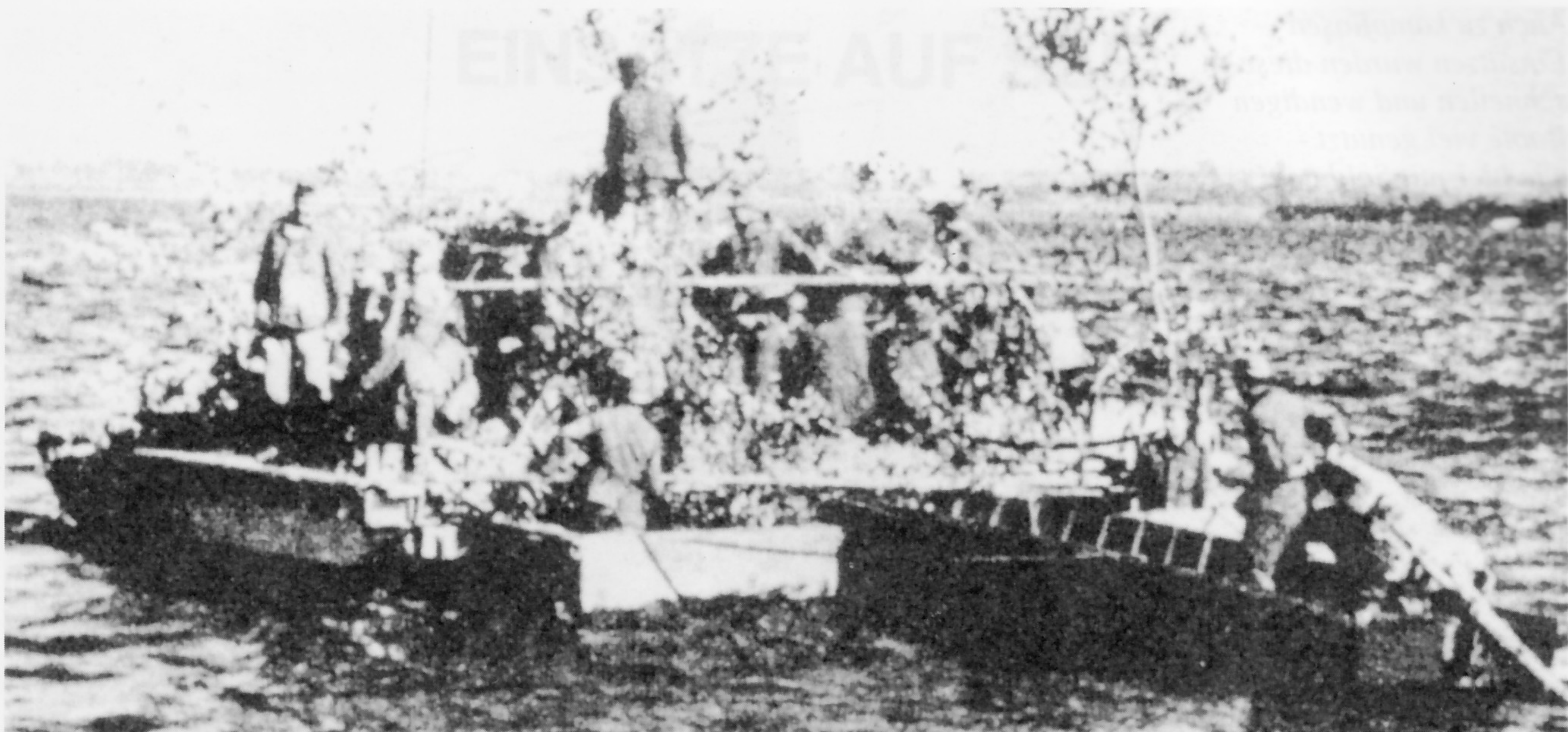
Bild 5. Großer Floßsack zwischen 2 Pi.-Sturmbooten.
