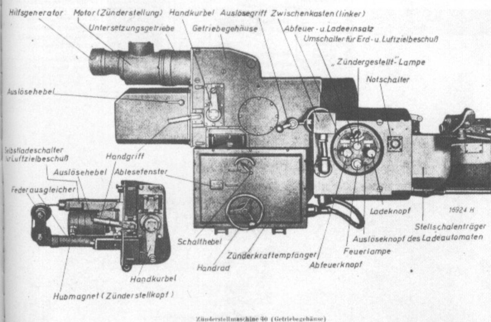
Zünderstellmaschine 40 (Getriebegehäuse)
