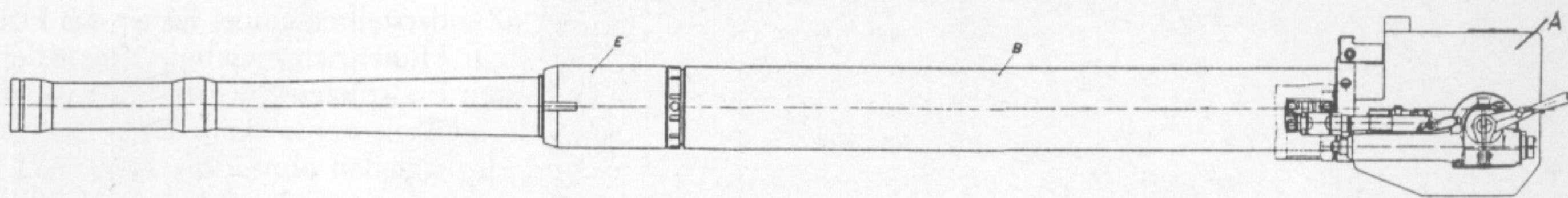
Abb. 3. Längsschnitt.
