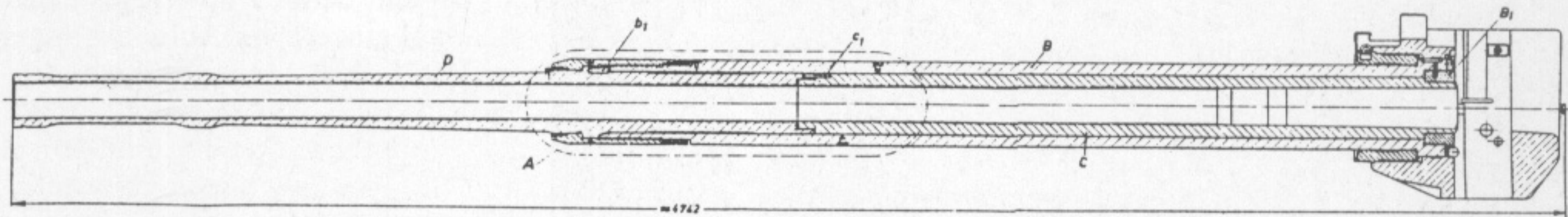
Abb. 3. Längsschnitt.
