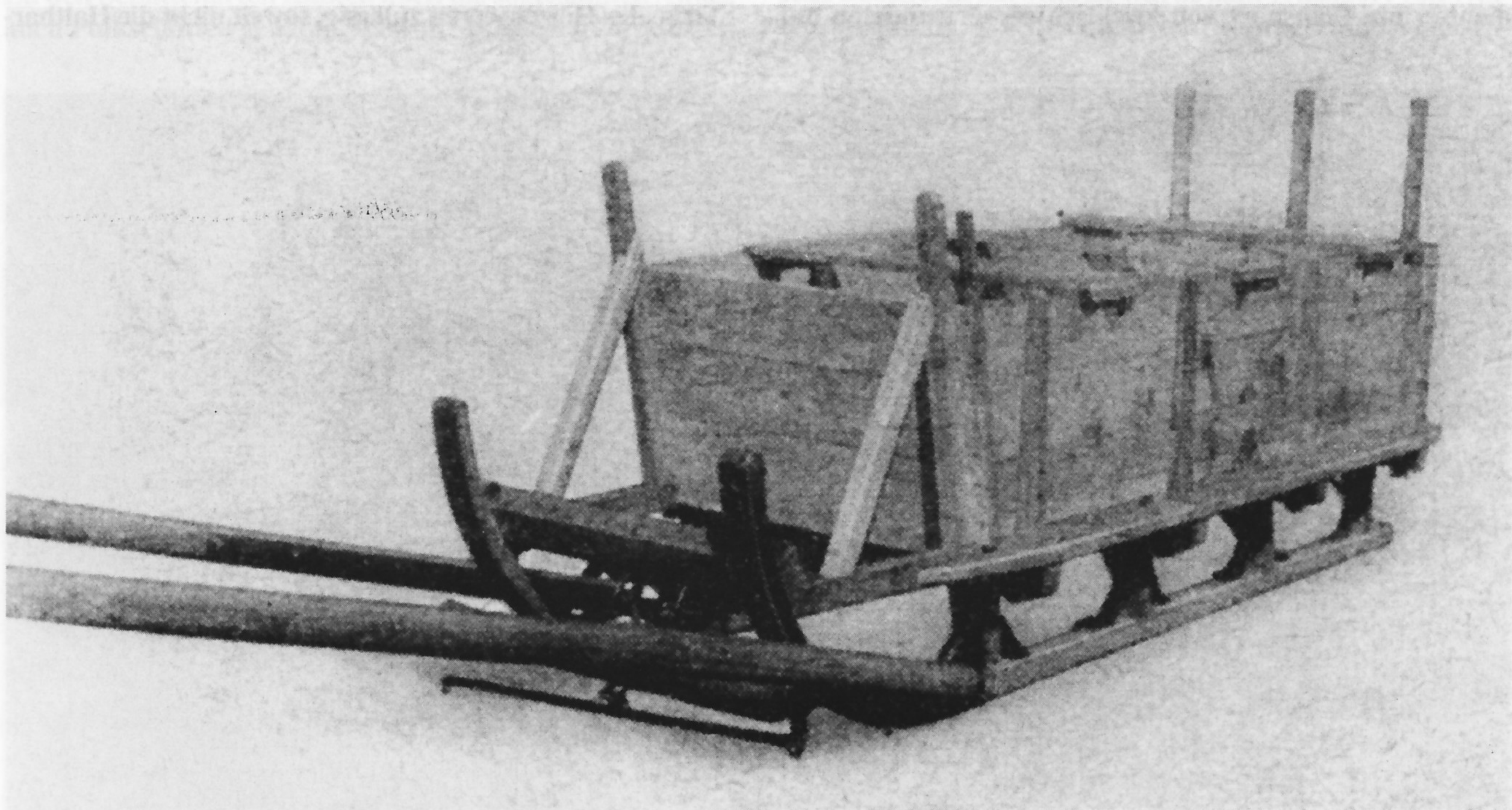
Der Schlitten 300 kg (Hs 1) mit Aufbau; hier als Transportschlitten für die Beförderung von Mannschaften. Die beiden hinteren Sitzbretter wurden von der Rückwand abgenommen und als Sitze quer über die Seitenwände gelegt. Das vordere Sitzbrett diente als Fahrersitz. Einige der nachfolgenden Demonstrations-Aufnahmen sind den Deckblättern Nr. 1-4 zur D 72 vom 26.8.1942 entnommen, daher läßt die Bildqualität zu wünschen übrig
