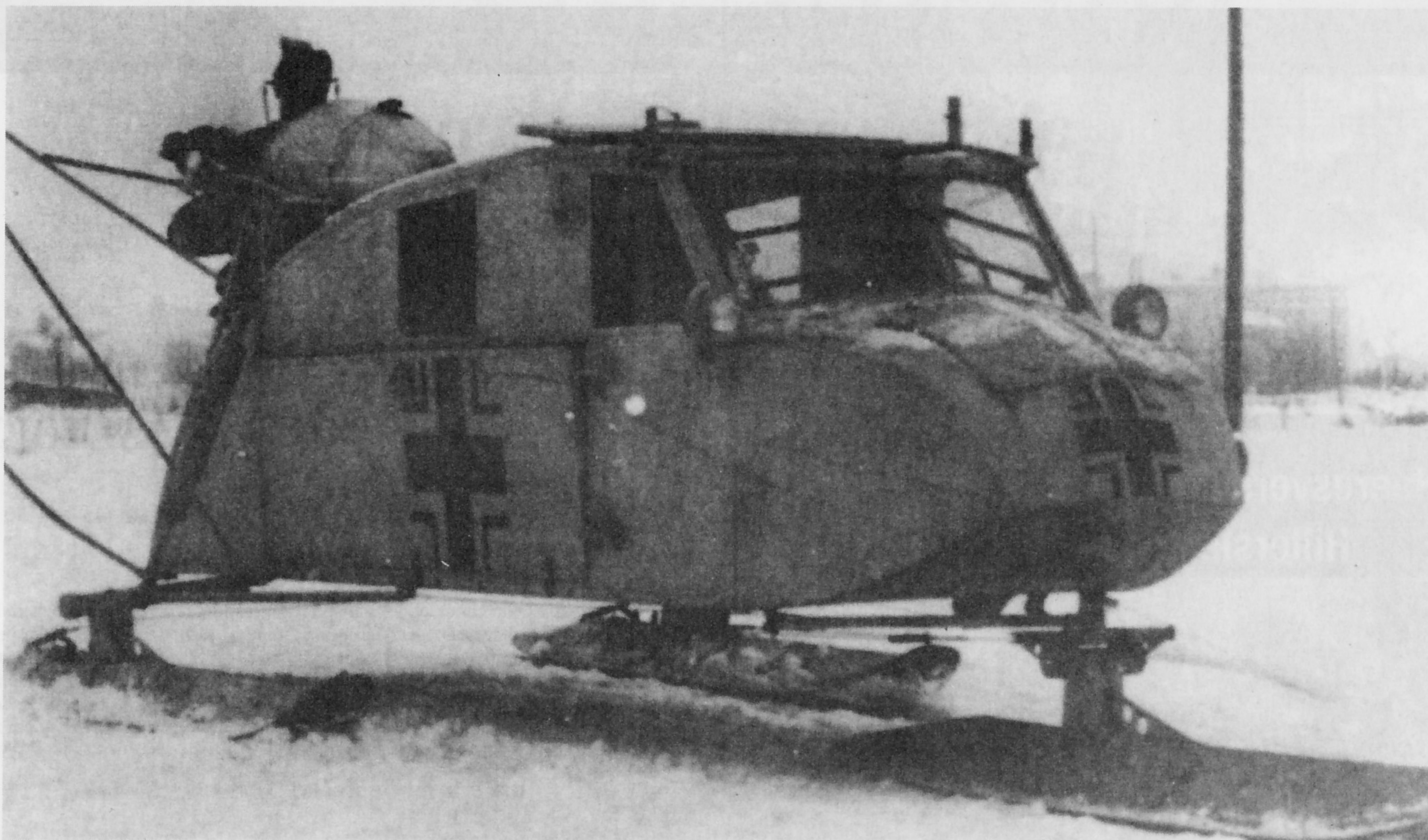
Die breiten Skikufen des Motorschlittens wurden vom Fahrer über einen Drahtseilmechanismus gesteuert. Das Führerhaus des Schlittens ähnelte dem eines Autos mit Lenkrad, Pedale und Armaturenbrett
