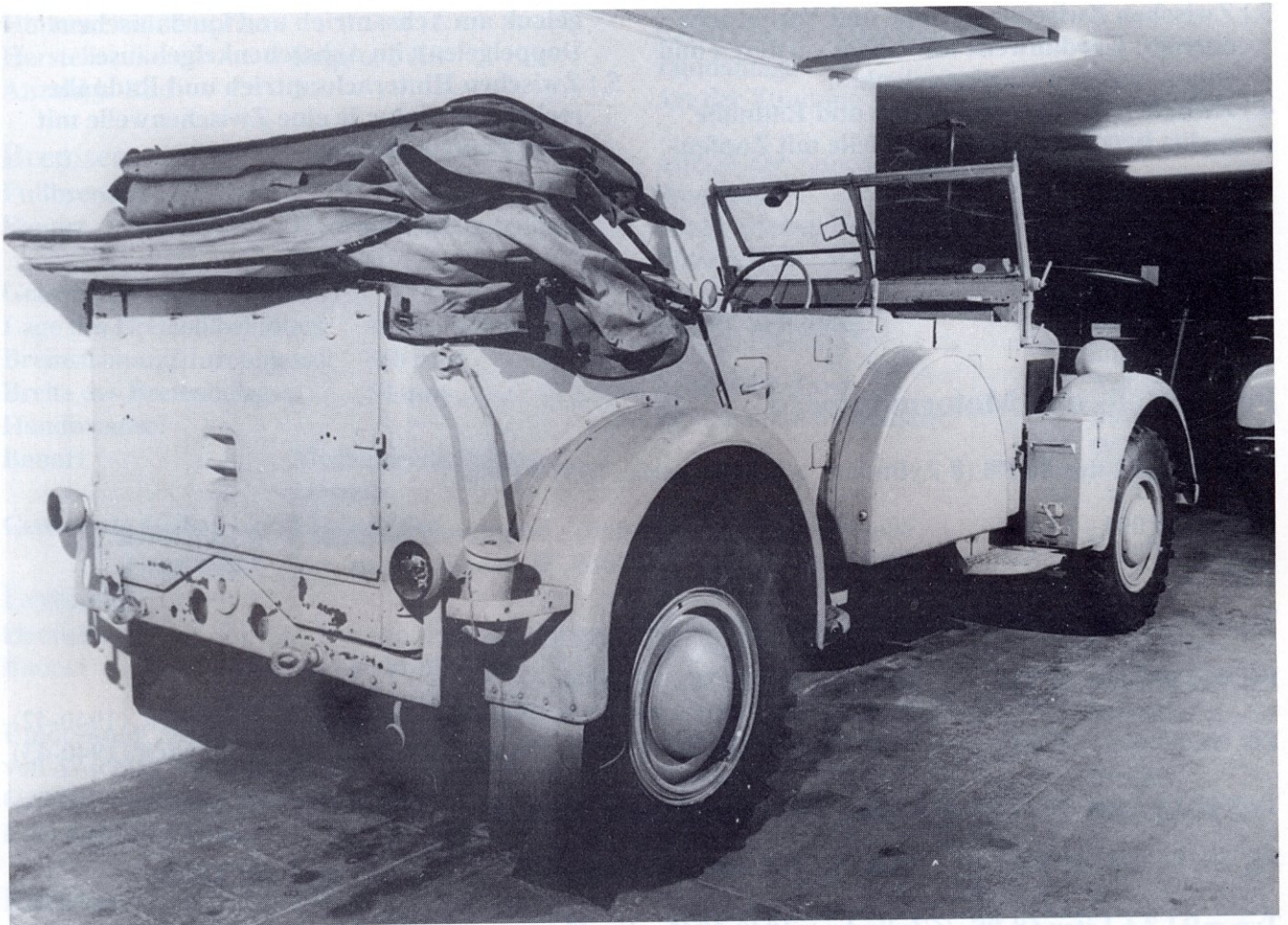
Rückansicht eines mittleren Einheits-PKW, auffallend hier die Abdeckung der seitlichen Stützräder.
