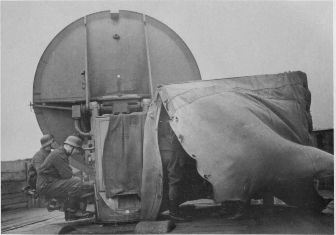
Durch eine Zeltplane geschützt, arbeiten der B1 vor der Braunschen Röhre des Entfernungsfineßmeßgerätes, der B2 am Richtrohr für die Seite und der B3 am Höhenrichtrohr.
