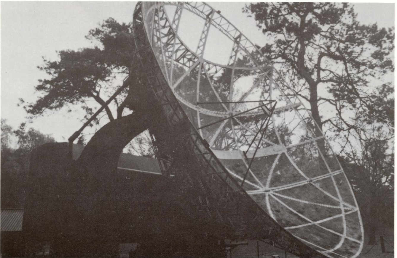
Beide Bilder zeigen das Gerät "Würzburg-Riese" ohne Dipol als Besichtigungsobjekt bei Schaarsbergen.
