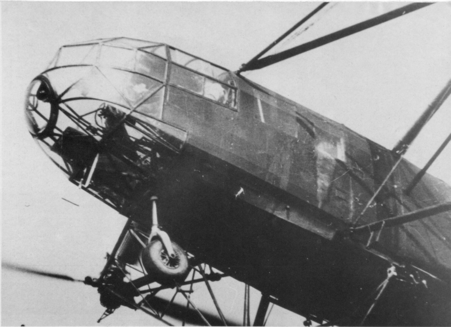
Nahaufnahme der Fa 223 V14 (DM+SR). Unter dem Rumpf ist das Hebegeschirr erkennbar, wie es bei der Fa 223 D eingeführt werden sollte.
