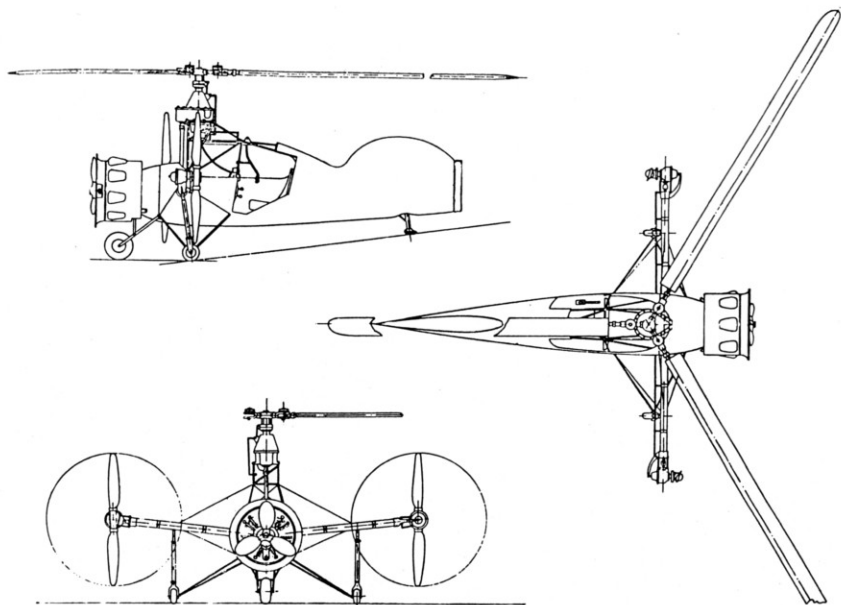
Zeichnung der F1 185 V1 (D-EFLT).
