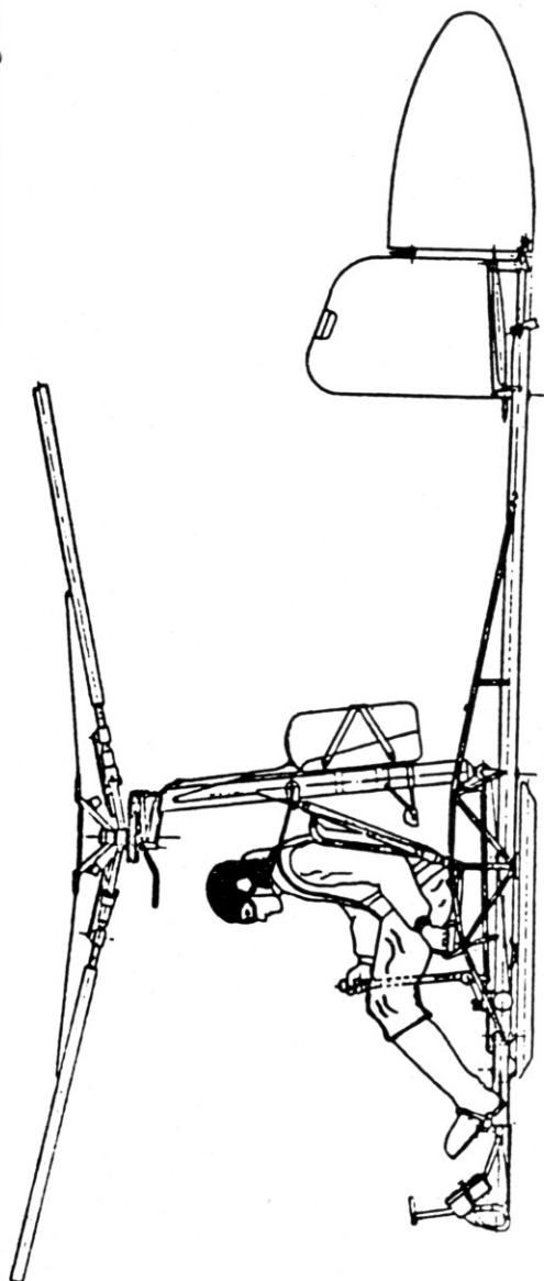
Übersichtszeichnung der Fa 330.
