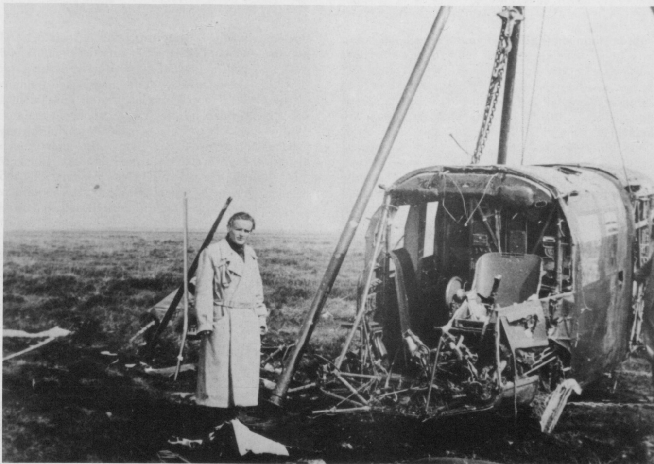
Blick in den Führerraum der Fa 223 V13.
