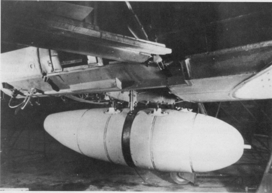
Speziell für Überlandflüge und für die Verwendung als U-Boot-Jagdhubschrauber konnte ein 300-l-Abwurfbehälter mitgeführt werden.
