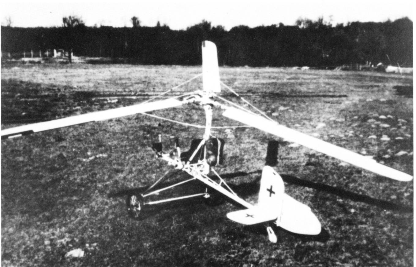
Landausführung der Fa 330 mit Rädern.
