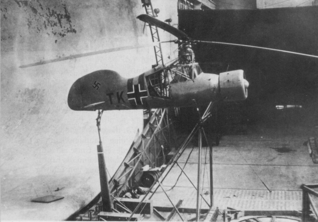
Links: Eine der sechs F1 265 während der Windkanalerprobung in Chalais-Meudon bei Paris.
