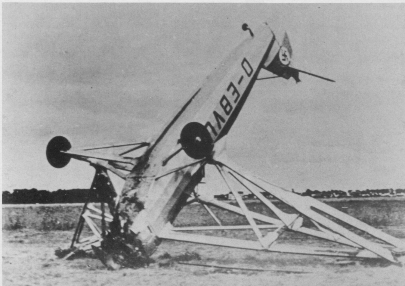
Bruch des ersten Versuchsmusters Focke 61 V1.
