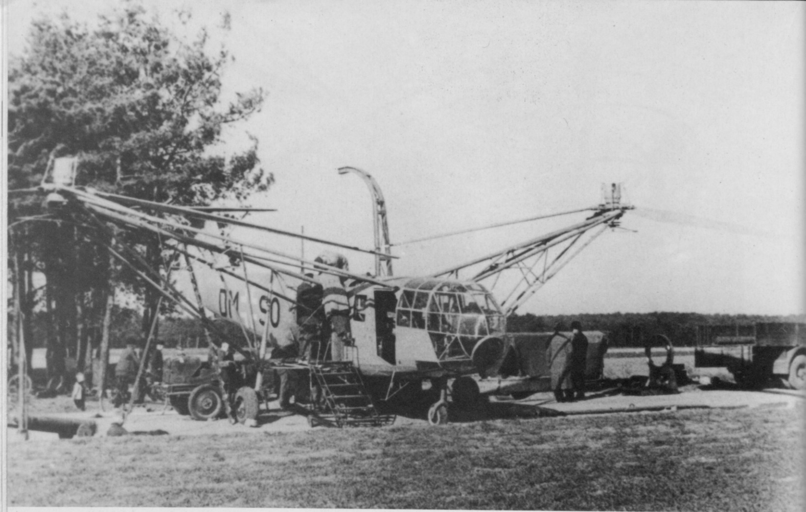
Motorwechsel unter Feldbedingungen 1943 in Norddeutschland.
