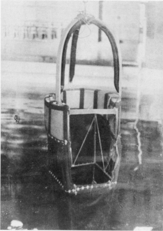
Rettungskorb der Fa 223 C während der Funktionserprobung in der Halle.
