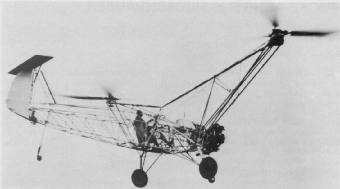
Erstflug der Focke 61 noch ohne Rumpf- verkleidung.
