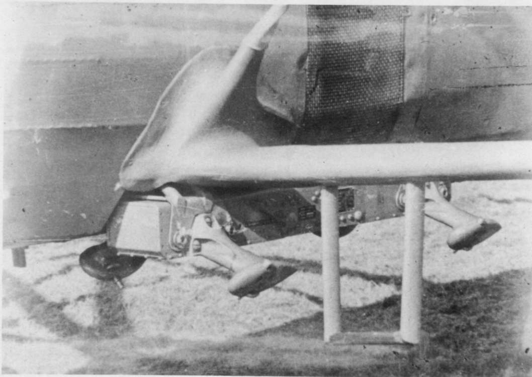
Nahaufnahme des Rumpfs-ETC der Fa 223 A und B.
