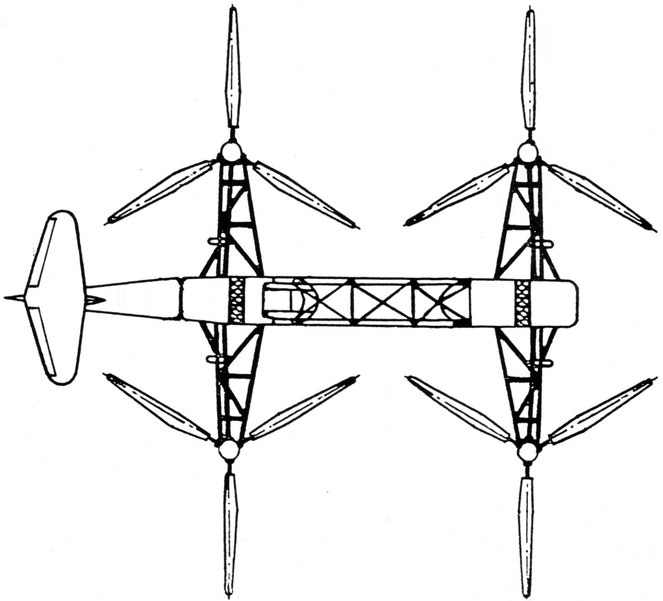
Übersichtszeichnung der Fa 223 "Zwilling" ("Krabbe"), die aus zwei gekoppelten Fa 223 bestehen sollte.
