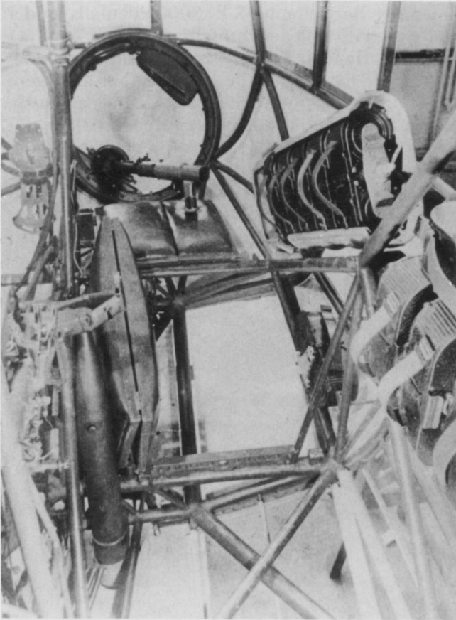
Zwei Aufnahmen des mit einem MG 15 bestückten Waffenstands und der Lagerung der Munitionstrommeln bei der Fa 223 V2.
