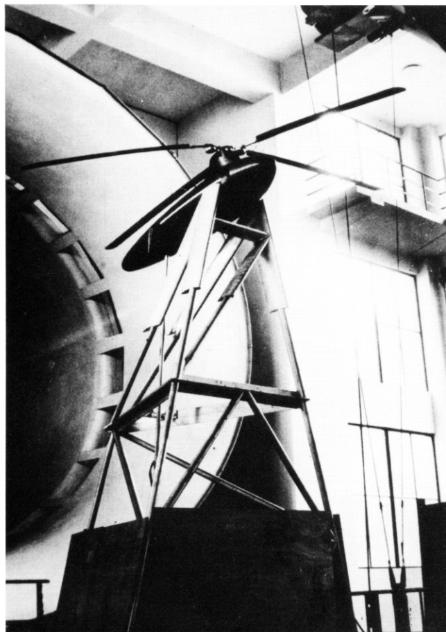
Windkanalmodell der Fl 282 "Kolibri".
