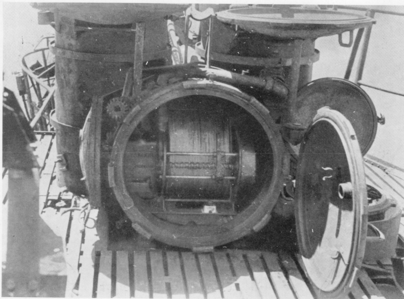
Unten: Windenanlage für den Einsatz der Fa 330 (U 852), Mai 1944.
