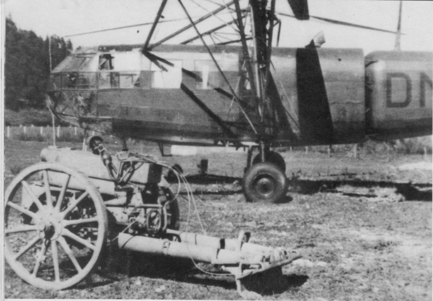
Oben: Ein Gebirgsinfanteriegeschütz GebIG 18L vor der Verlastung.
