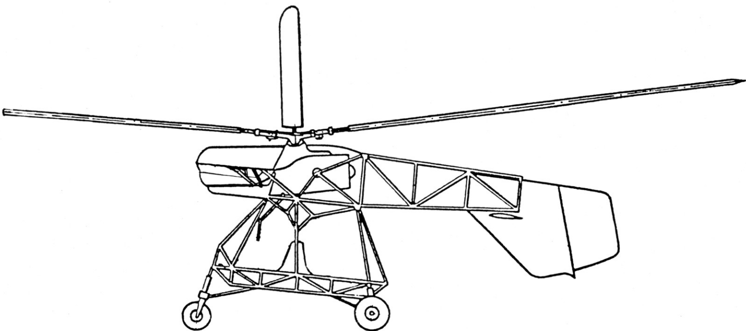
Seitenansicht der Versuchsausführung der F1 339.
