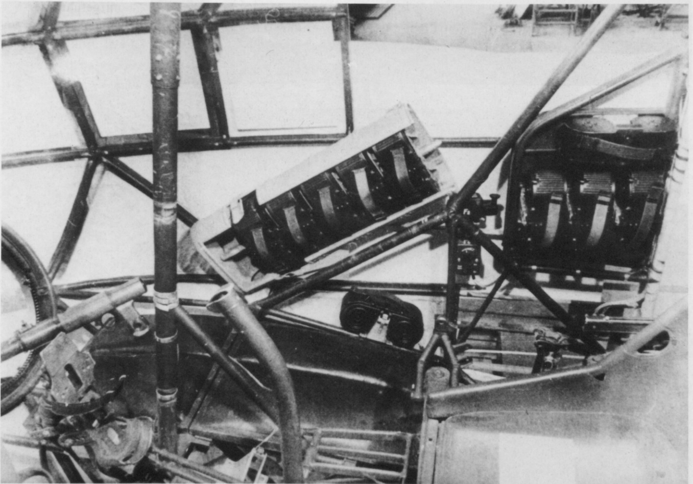
Zwei Aufnahmen des mit einem MG 15 bestückten Waffenstands und der Lagerung der Munitionstrommeln bei der Fa 223 V2.
