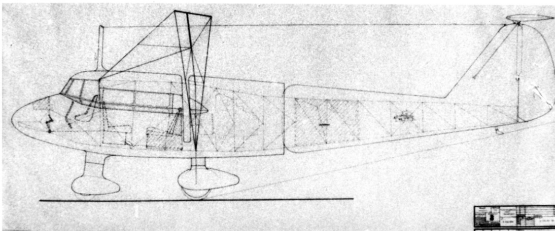
Seitenansicht der geplanten Zivilversion der Fa 223, welche die Typenbezeichnung Fa 266 trug.
