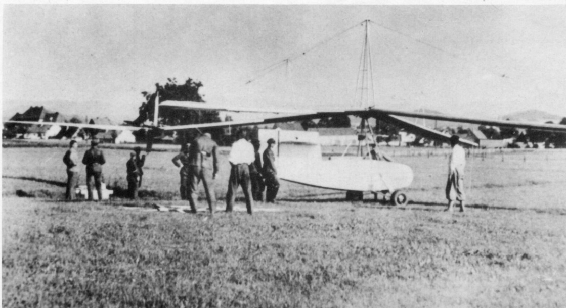
Der Flettner-Versuchshubschrauber mit 30 m-Rotordurchmesser kurz vor dem ersten Fesselflug.
