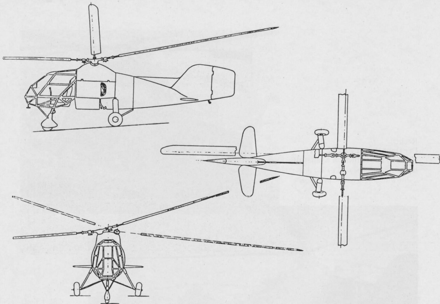
Zeichnung der einsitzigen F1 282 B-1 mit verglastem Führersitz.
