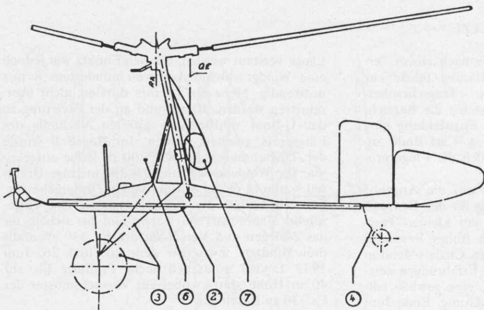
Handbuchzeichnung der Fa 330, die mit einem Rettungsfallschirm (7) ausgerüstet werden sollte.
