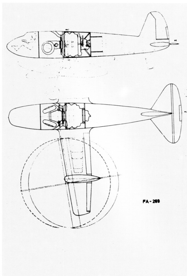
Übersichtszeichnung des ersten Prototyps des Kipprotorflugzeugs Fa 269, welches zunächst einen BMW-Antrieb erhalten sollte.
