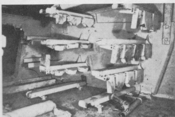
Unten: Das Foto zeigt die Halterungen der Patronengranaten im linken hinteren Turmteil.
