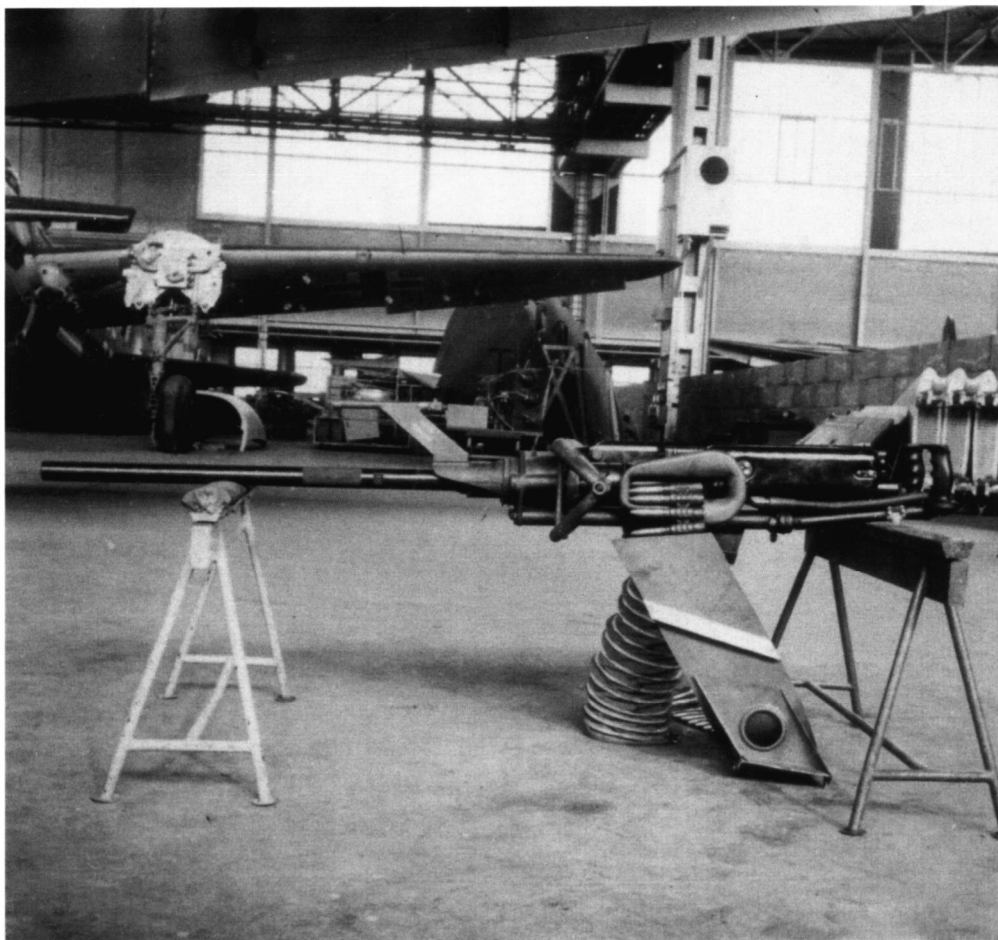
Nahansicht eines ausgebauten MG 151/20 mit Hülsenabfuhr.
