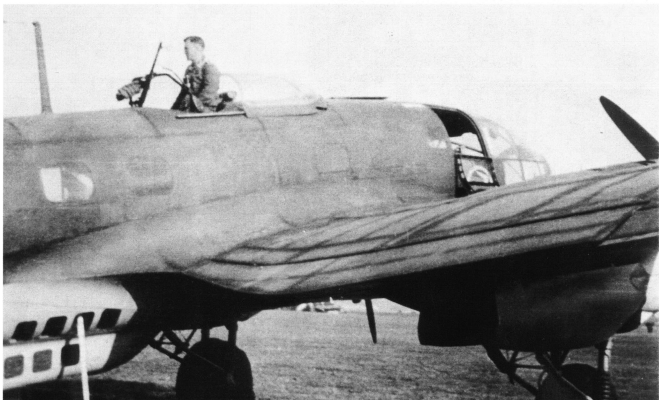
Noch ohne Panzerung war auch der B-Stand der He 111 H-1 bis H-6 ausgelegt.
