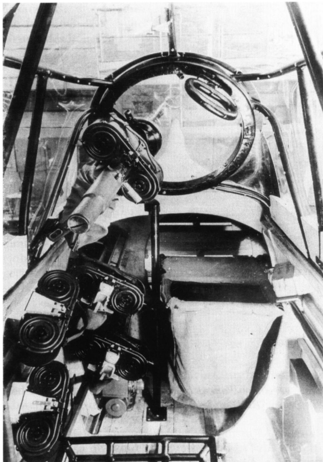
Attrappenfoto der Ju 87 B-1 mit einem MG 15 in einer Linsenfahne.
