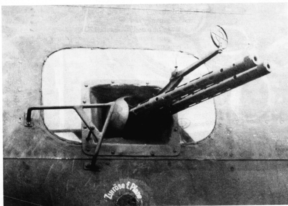
Bei der He 111 H wurden die einzelnen MG 17 mit der Zeit gegen MG 81 Zwillingswaffen ausgetauscht.
