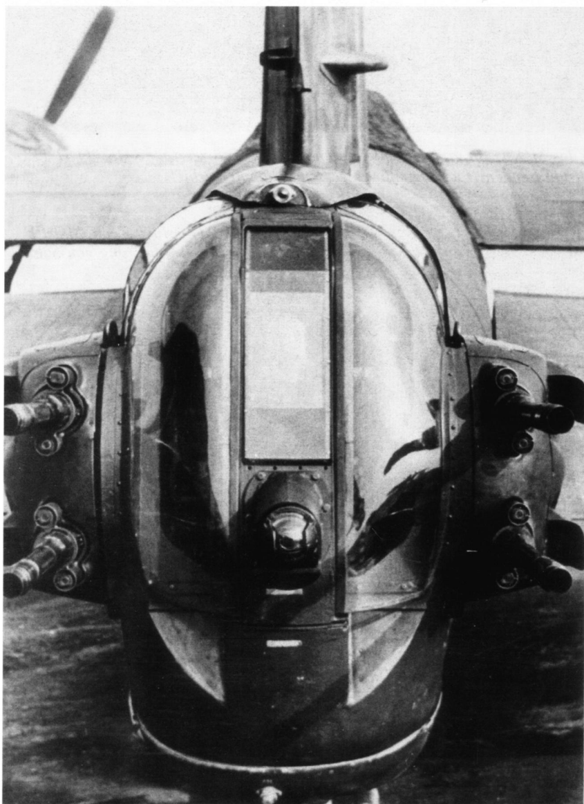
Im Heck dieser He 177 wurde versuchsweise dieser Heckstand installiert, dessen Bestückung ebenfalls aus vier MG 131 bestand.
