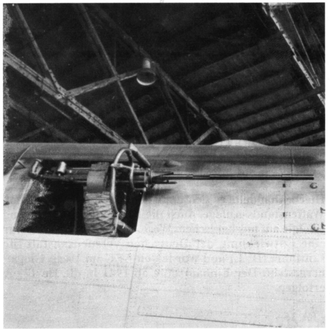
Als bewegliche Seitenbewaffnung, hier bei einer Ju 290 A, war das schwere MG 151/20 meist unverzichtbar.
