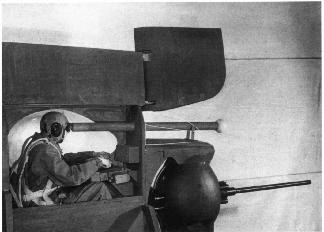
Der vorläufige Waffeneinbau für ein MG 151/20 mit Zielfernrohr, wie er bei der Ju 188 G-2 geplant war.
