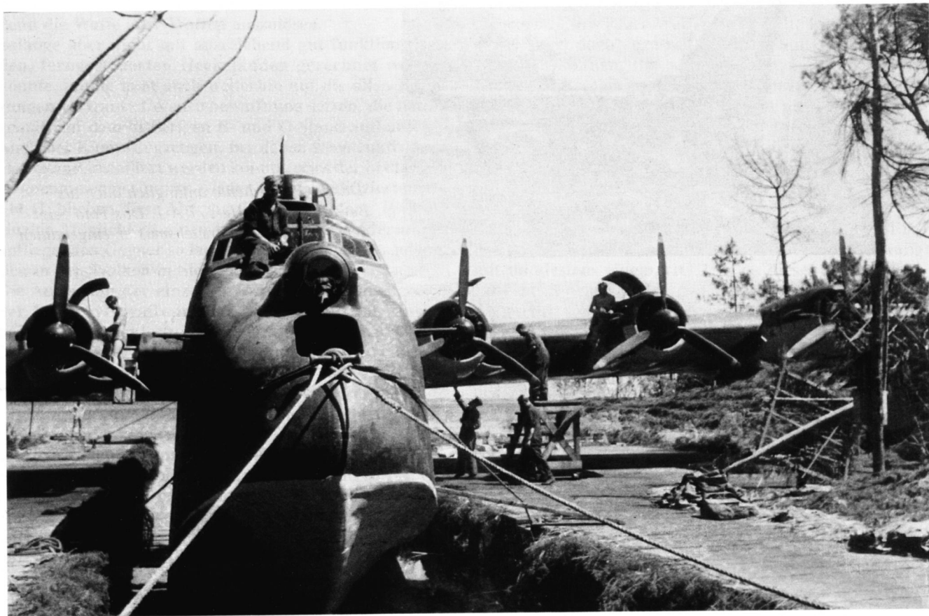
Auf dem Rumpfbug mehrerer BV 222-Großflugboote fand sich ein MG 131 in teilgepanzerter Linsenlafette.
