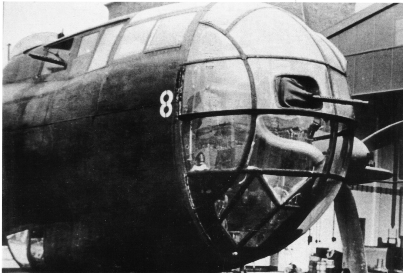
Mustereinbau des MG 131 bei der Do 217 M-1.
