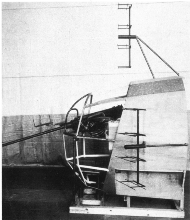
Attrappenmäßiger Einbau eines MG 151/20 bei der Ju 290.
