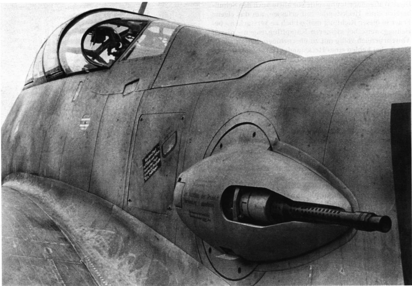
Nahansicht der beweglichen Bewaffnung mit aufgesetzter Verkleidung.
