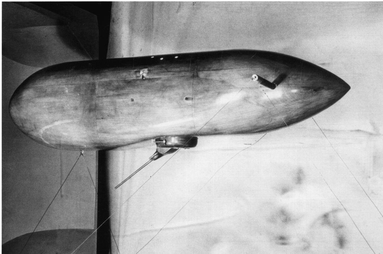
Windkanalmodell eines fernbedienten Waffenstandes mit MG 151/20-Bestückung.
