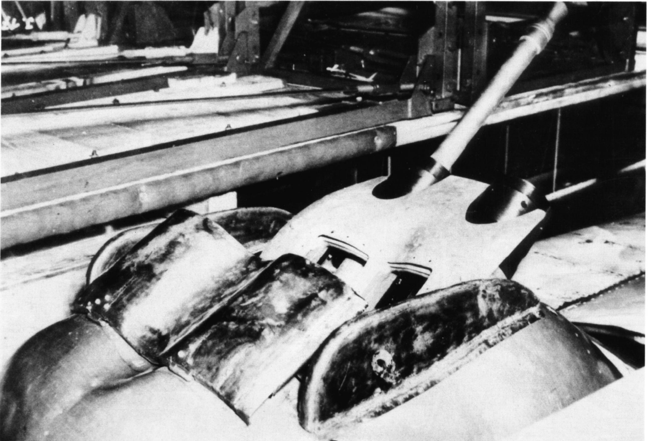
Musterbau eines Waffenstandes mit MG 131-Bestückung, der bei Arado für die Ar 240 entwickelt wurde.
