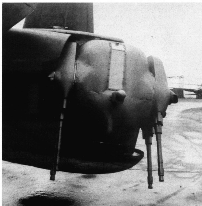
Zwei Ansichten des für die Ju 288 und die He 219 geplanten MG 131-Heckturmes.
