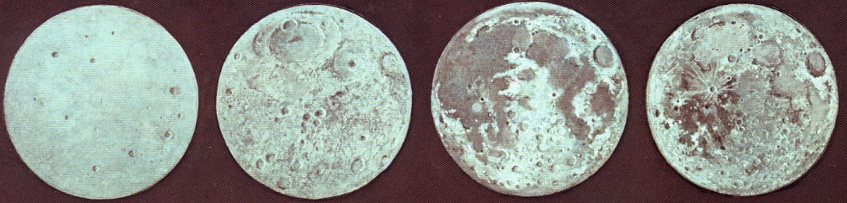
Der Mond vor 4,5 Milliarden Jahren. Eine feste Kruste hat sich gebildet, Krater entstehen.
