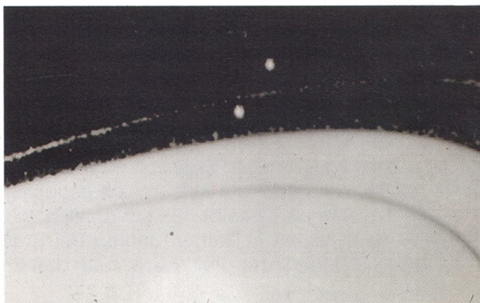
Die beiden Schäferhundmonde halten ihre „Herde“, die Teilchen des F-Ringes, zusammen.
